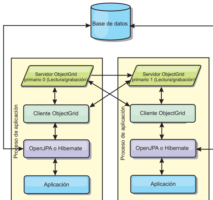
Figura 13. Topología incorporada con particiones JPA
