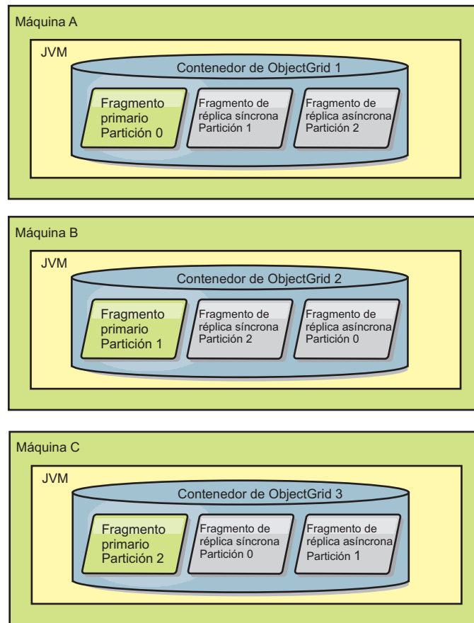
Figura 31. Colocación de un conjunto de correlaciones de ObjectGrid con una política de despliegue de 3 particiones con un valor minSyncReplicas de 1, un valor maxSyncReplicas de 1 y un valor maxAsyncReplicas de 1
