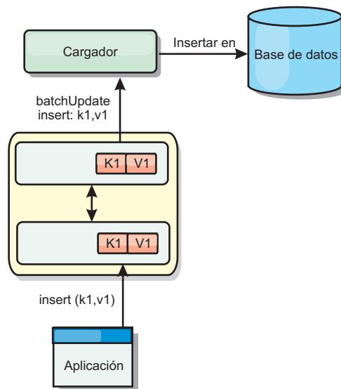
Figura 21. Almacenamiento en memoria caché de grabación directa
