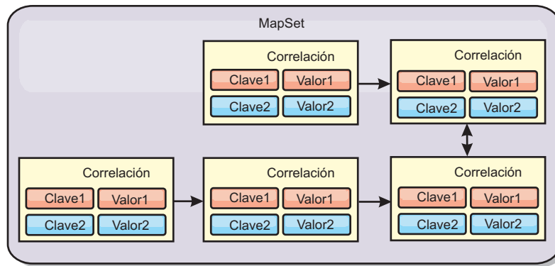
Figura 8. Conjuntos de correlaciones
