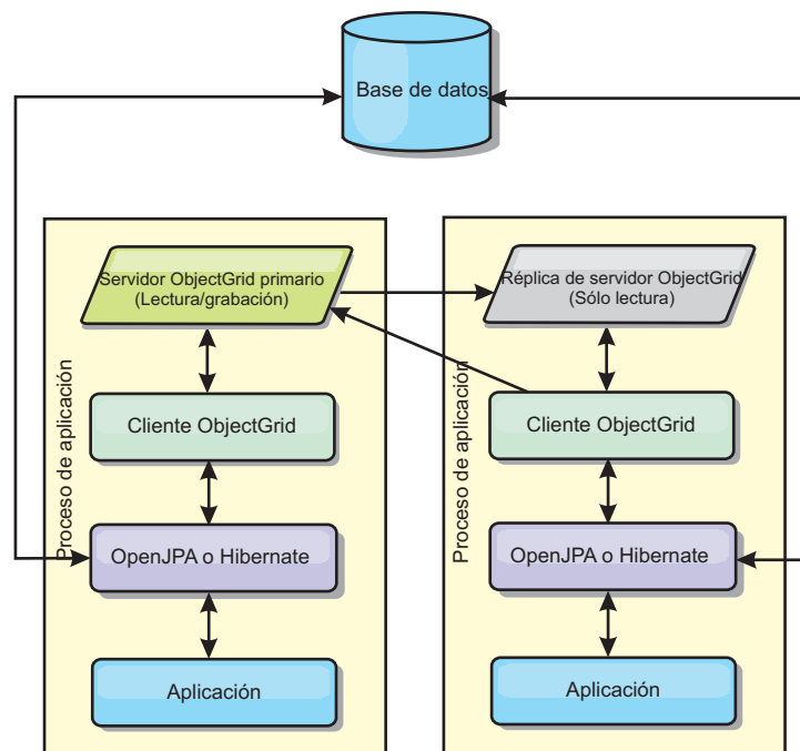
Figura 12. Topología incorporada JPA
