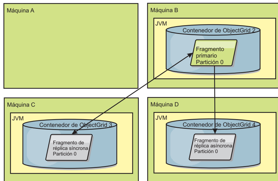
Figura 35. La máquina B contiene el fragmento primario. En función de cómo se establece la modalidad de reparación automática y la disponibilidad de los contenedores, un nuevo fragmento de réplica síncrona se podría colocar o no en una máquina.
