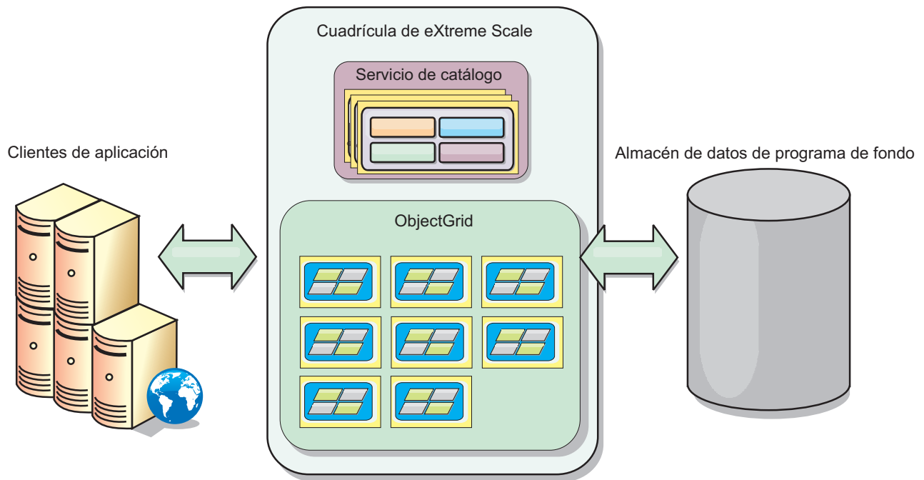
Figura 1. Topología de nivel superior
