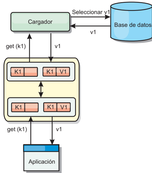
Figura 20. Almacenamiento en memoria caché de lectura directa
