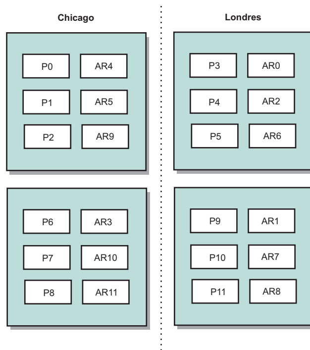
Figura 10. Primarios y réplicas en las zonas
