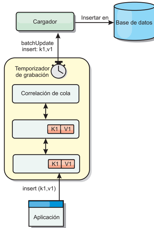
Figura 22. Almacenamiento en memoria caché de grabación diferida
