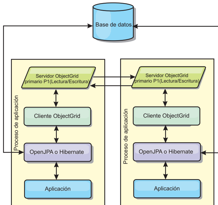
Figura 11. Topología interno del dominio JPA
