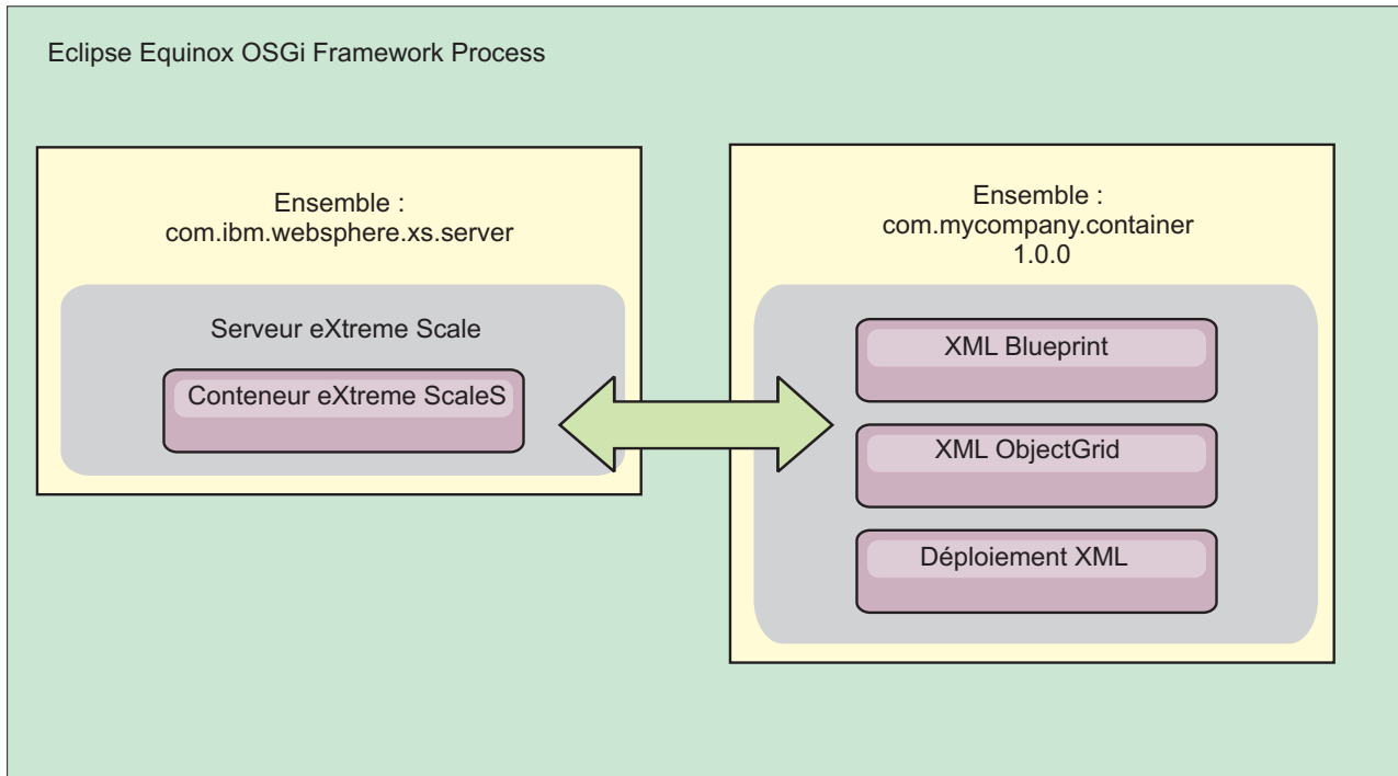
Figure 51. Processus Eclipse Equinox pour inclure toute la configuration et toutes les métadonnées dans un ensemble OSGi
