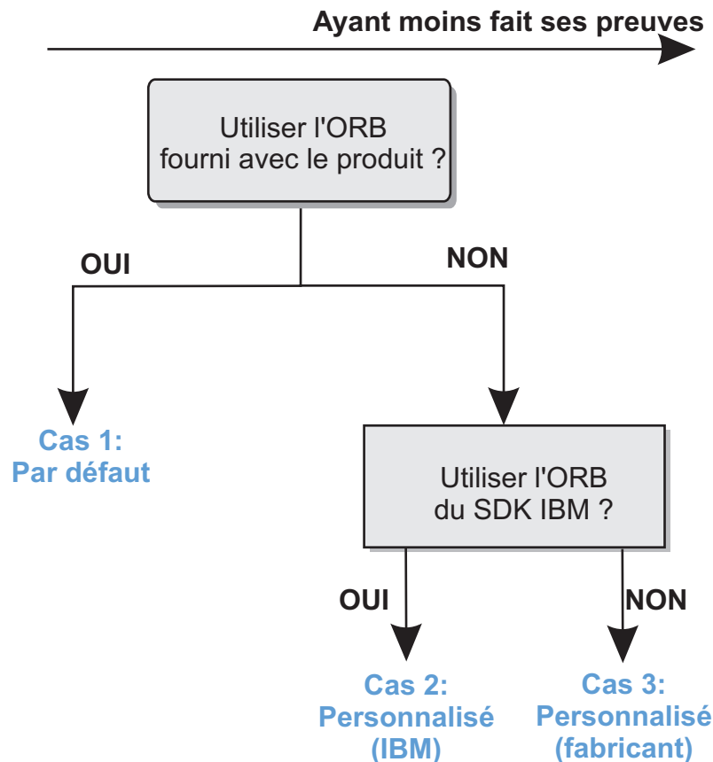
Figure 35. Choix de l'ORB
