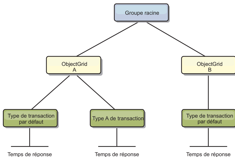
Figure 59. Exemple de structure de module ObjectGridModule
