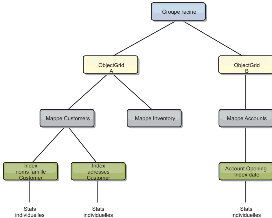
Figure 63. Exemple de structure de module hashIndexModule
