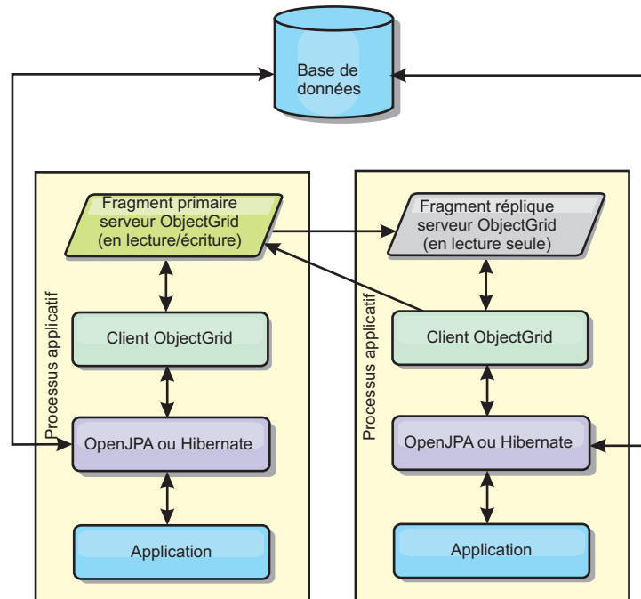
Figure 41. Topologie imbriquée JPA
