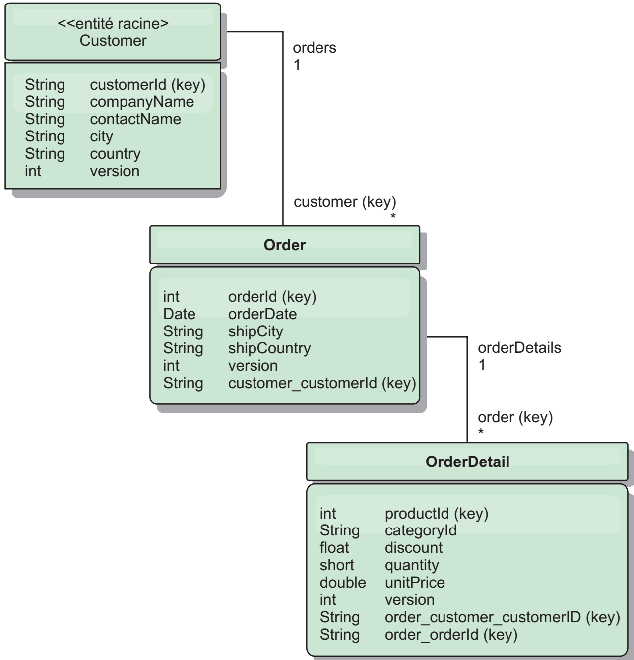
Figure 46. Schéma des entités Customer et Order
