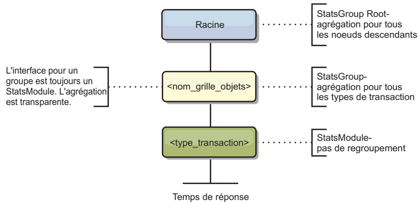
Figure 58. Structure de module ObjectGridModule
