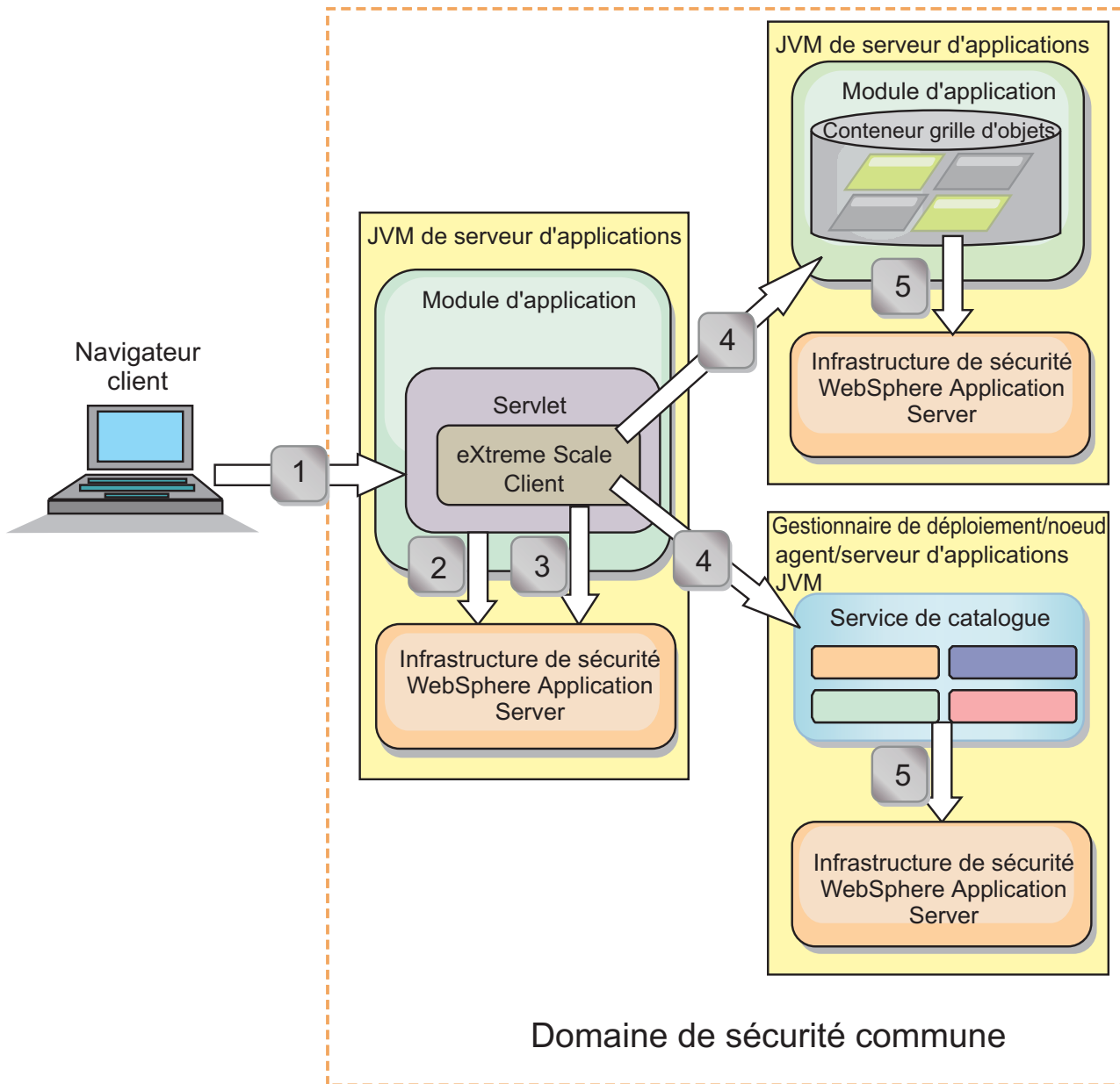
Figure 68. Flux d'authentification pour les serveurs dans le même domaine de sécurité
