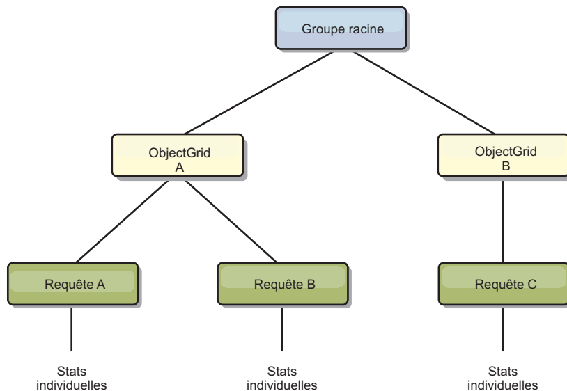
Figure 67. Exemple de structure queryModule QueryStats.jpg
