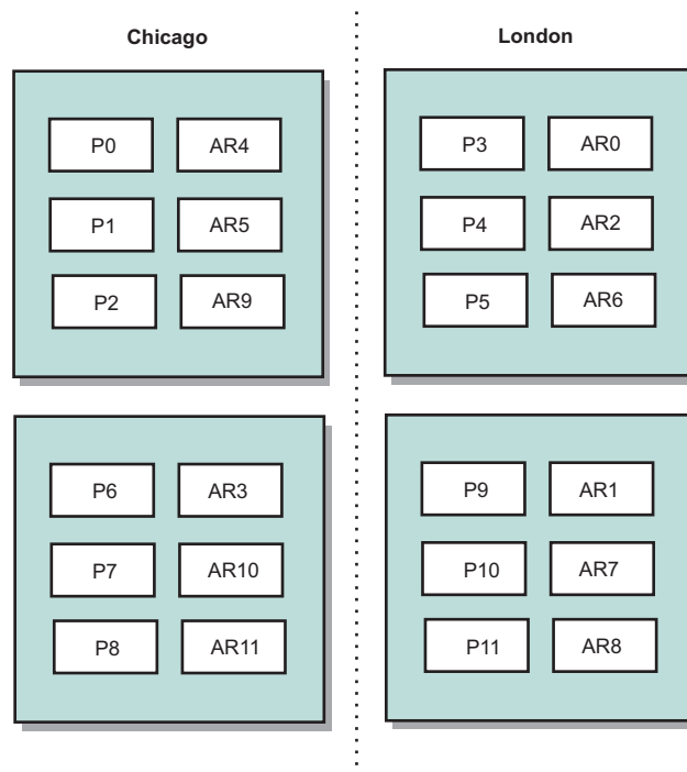
Figure 29. Segments principaux et répliques dans les zones
