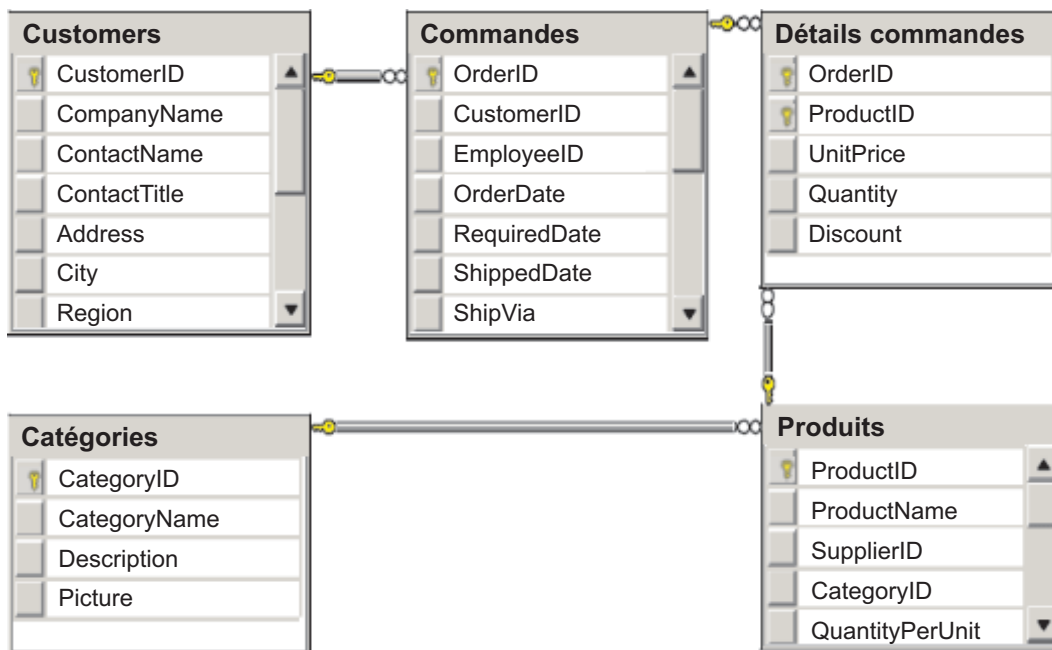
Figure 45. Schéma de l'exemple Microsoft SQL Server Northwind
