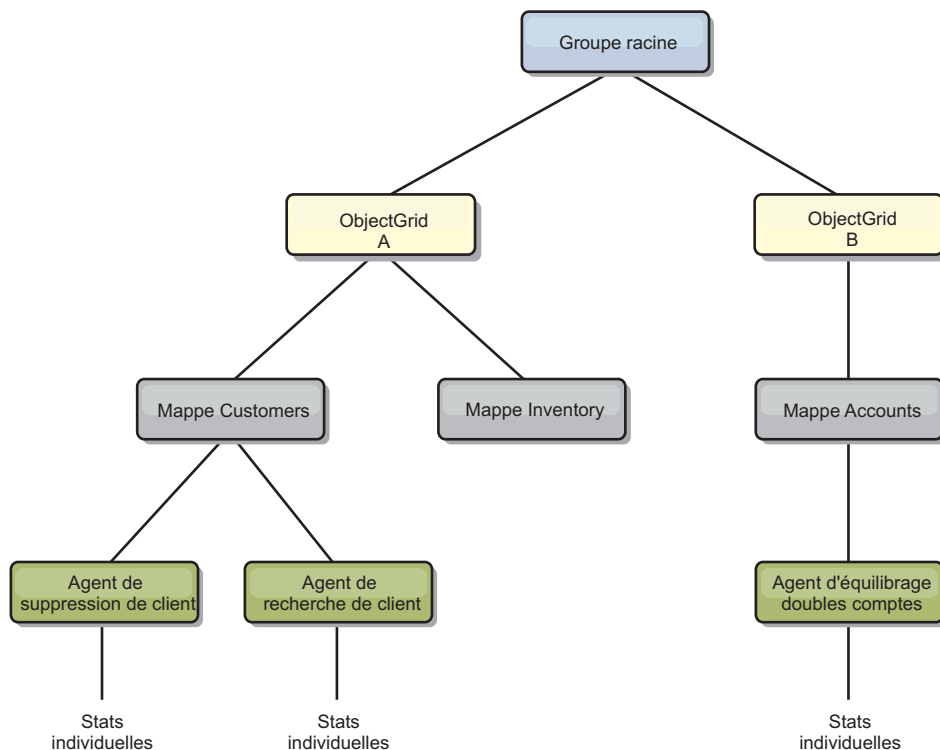
Figure 65. Exemple de structure agentManagerModule
