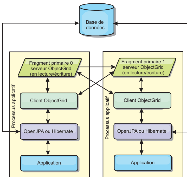
Figure 42. Topologie imbriquée et partitionnée JPA
