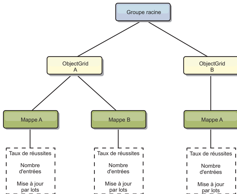
Figure 61. Exemple de structure de module mapModule
