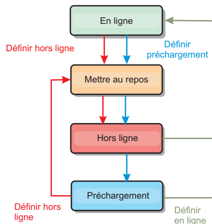
Figure 50. Etats de disponibilité d'une instance ObjectGrid
