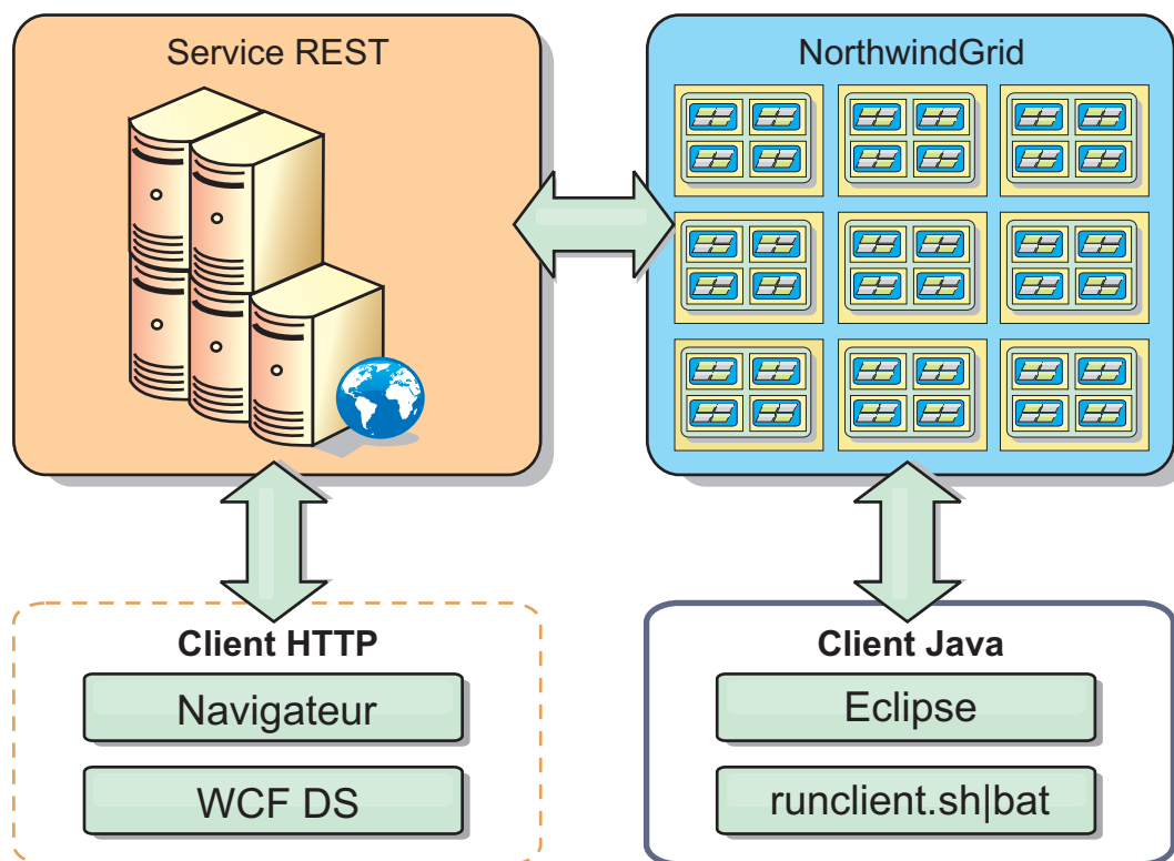
Figure 44. Exemple Mise en route de topologie. Les clients HTTP en utilisant le service de données REST et les clients Java peuvent accéder à la même grille de données.
