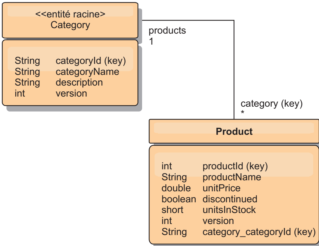
Figure 47. Schéma des entités Category et Product
