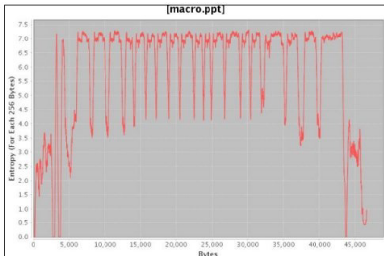
圖 3. 顯示內嵌 Script 的檔案熵圖的範例
