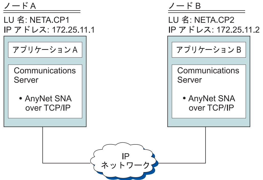
図 23. TCP/IP ネットワークを介した APPC または CPI-C アプリケーションの実行
