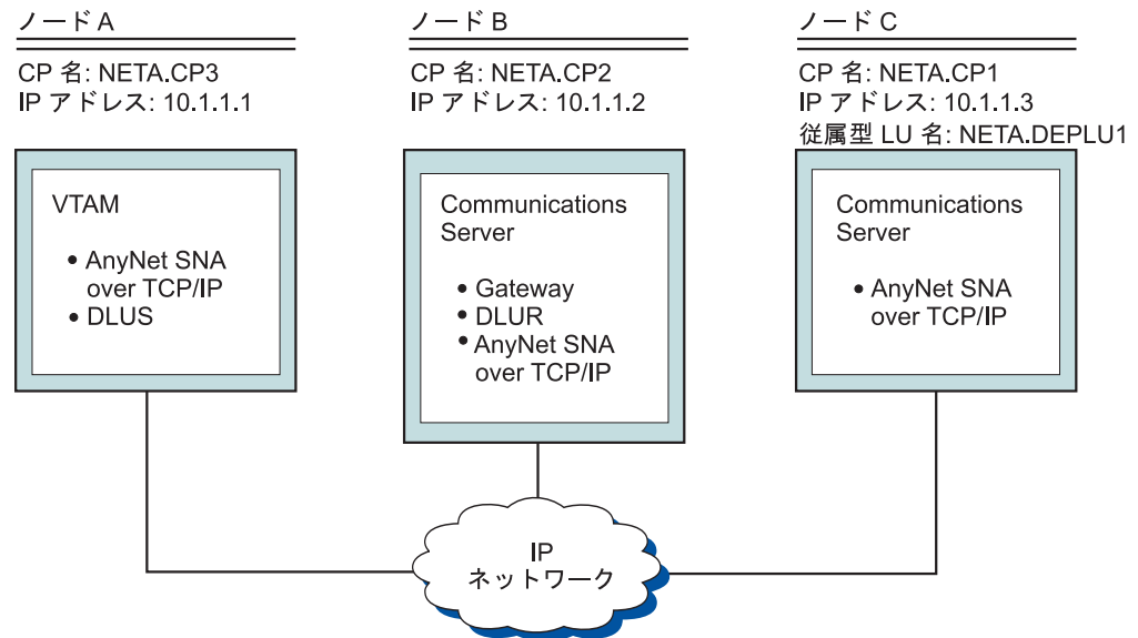
図 26. TCP/IP ネットワークを介する 3270 エミュレーションのための SNA ゲートウェイの使用
