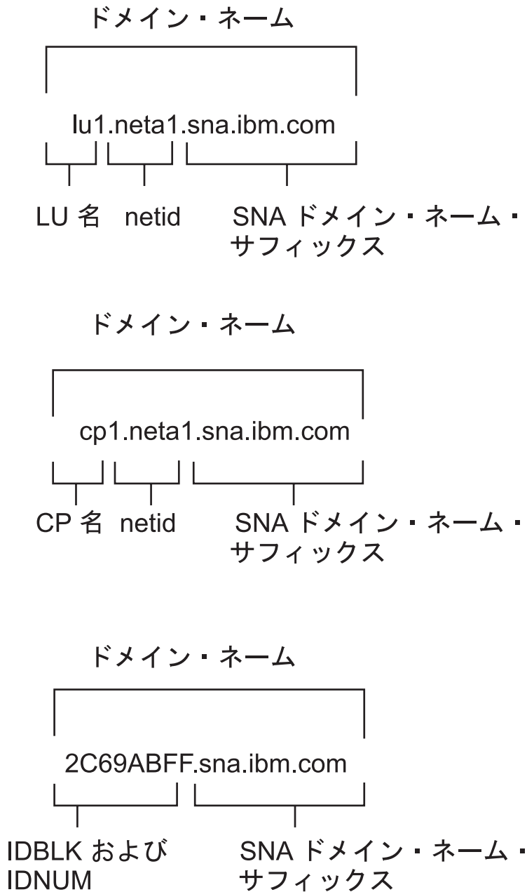
図 19. SNA over TCP/IP が作成するドメイン・ネームの形式
