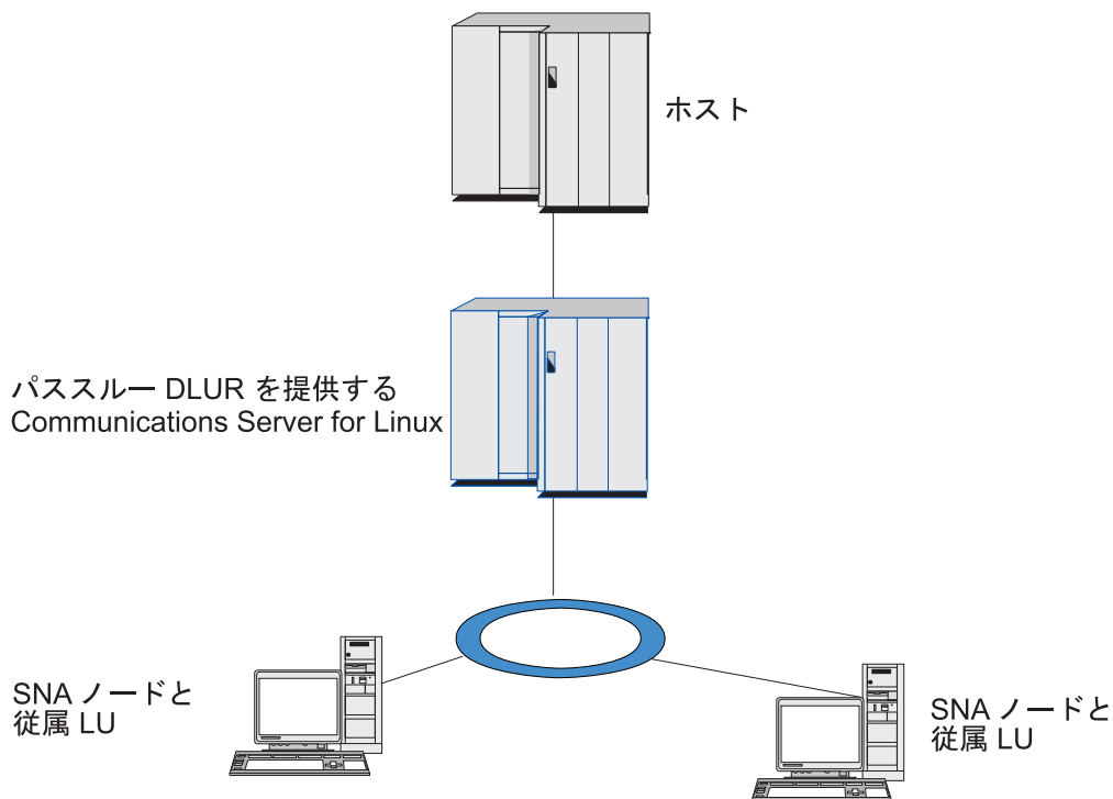
図8. DLUR を提供する Communications Server for Linux ノード
