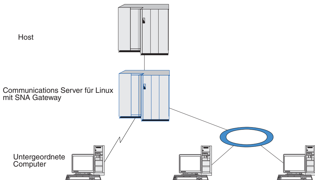
Abbildung 7. SNA Gateway
