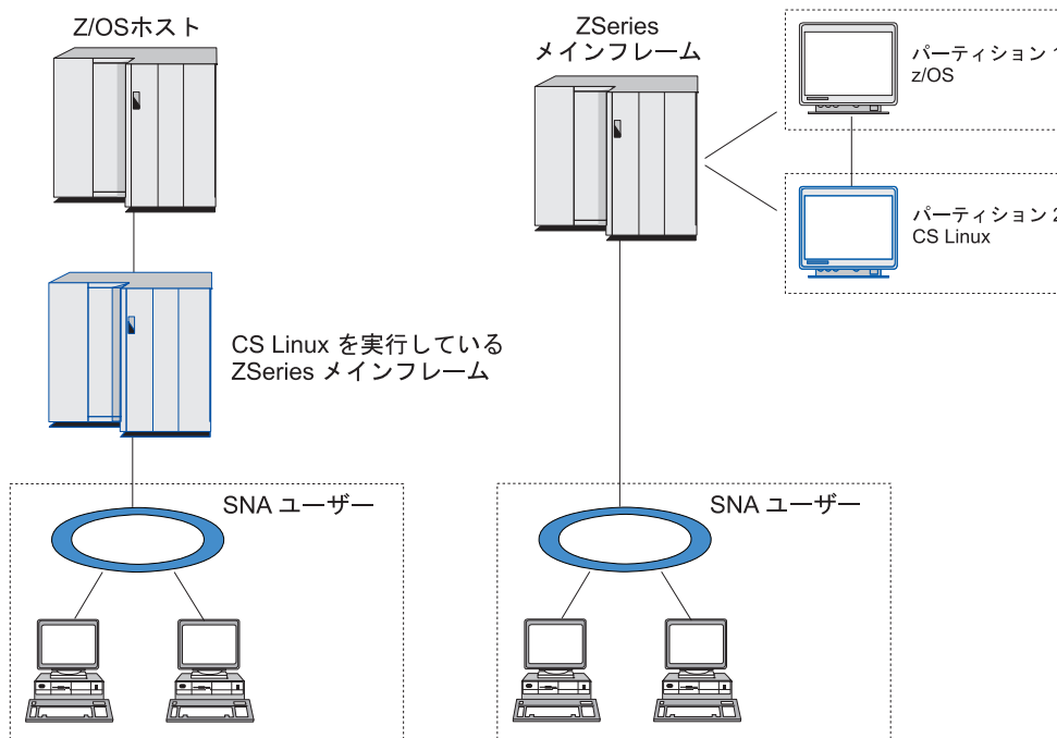
図1. Communications Server for Linux on System z のホスト通信
