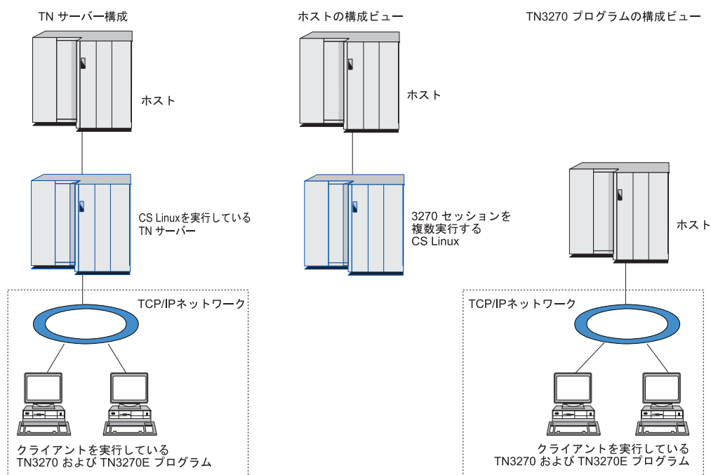
図 4. TN サーバー
