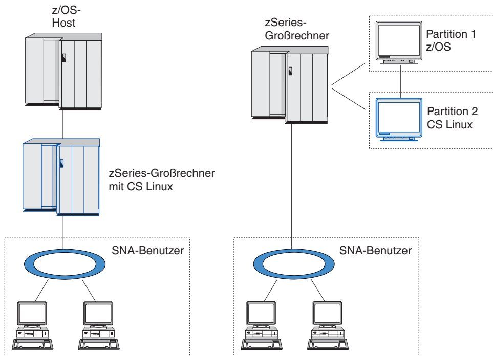
Abbildung 1. Hostkommunikation von Communications Server für Linux auf System z
