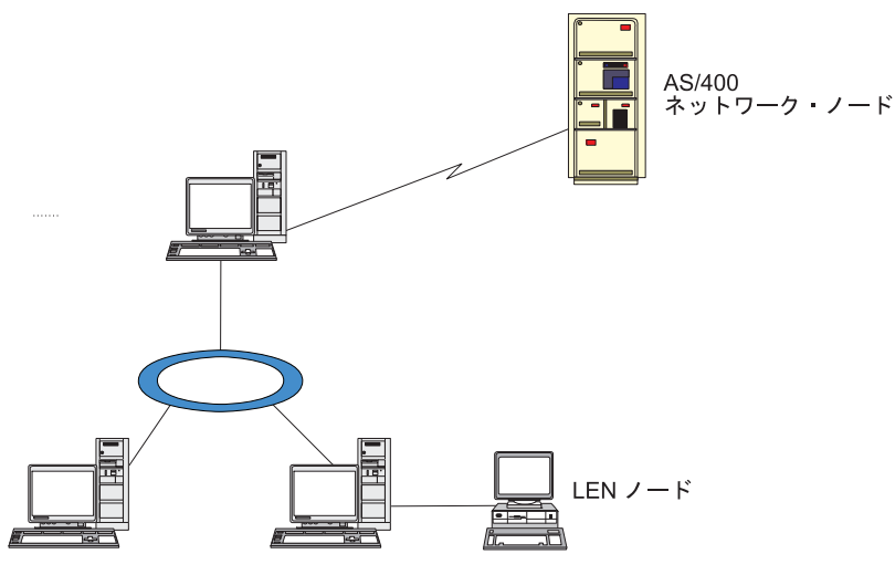
図 7. APPN ネットワークの CS Linux ノード
