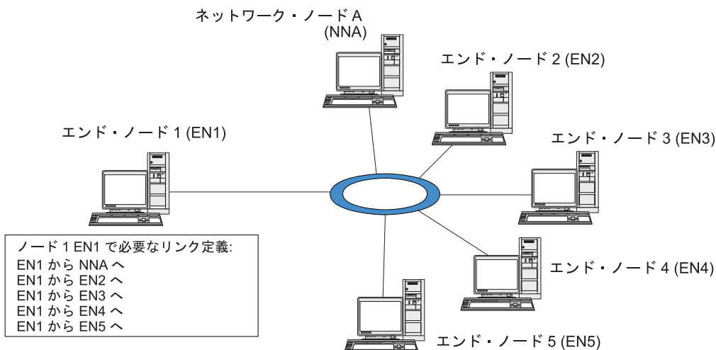
図 9. 共用アクセス・トランスポート機能を使用する APPN ネットワーク
