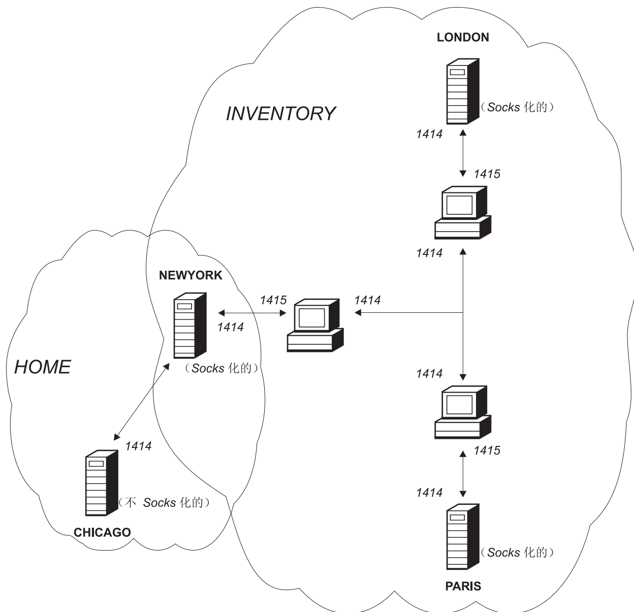
图 7. MQIPT 群集支持
