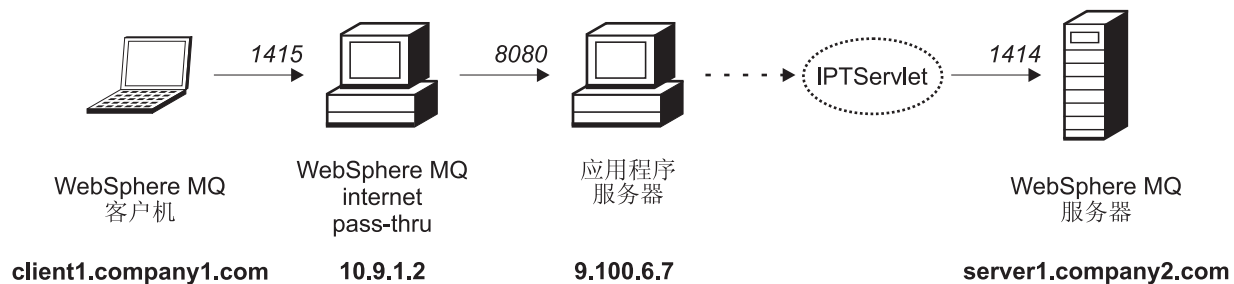
图 28. Servlet 网络图
