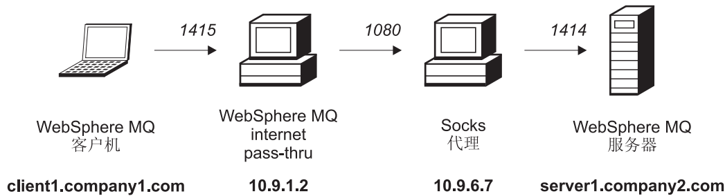
图 24. SOCKS 客户机网络图
