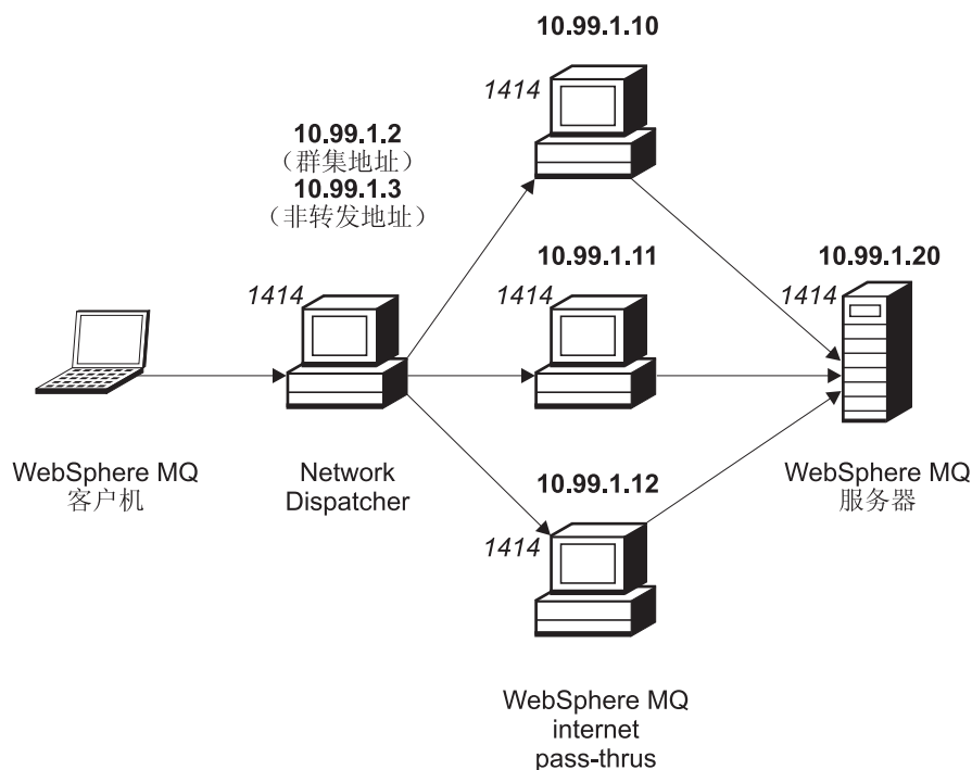
图 6. Network Dispatcher 与 MQIPT 一同使用
