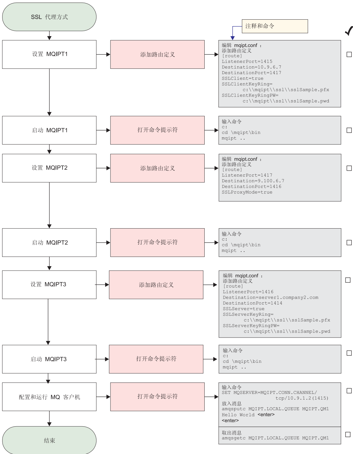
图 27. SSL 代理配置
