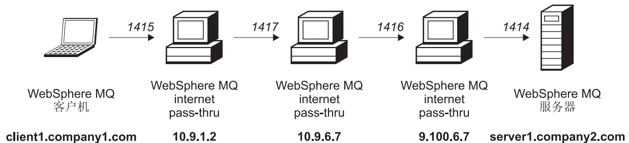
图 26. SSL 代理网络图
