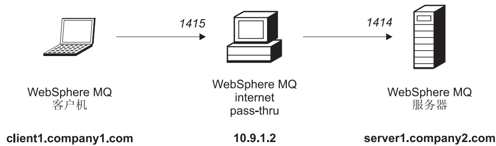
图 20. QoS 网络图
