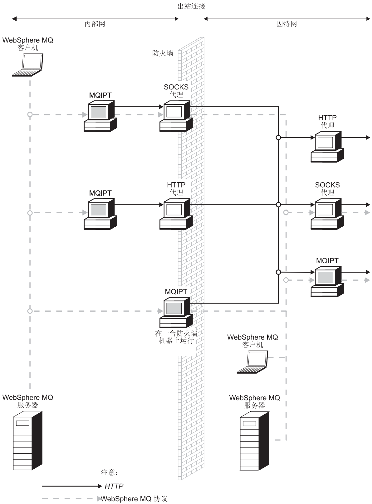
图 5. WebSphere MQ 拓扑结构显示了可能的 MQIPT 配置 (1/2)
