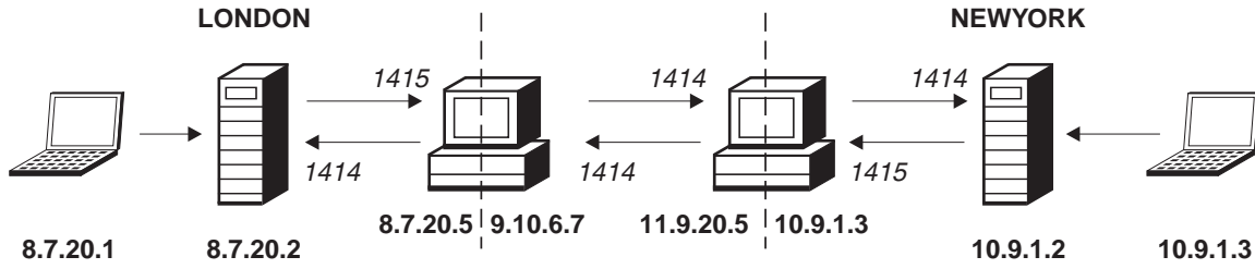
图 30. 群集网络图
