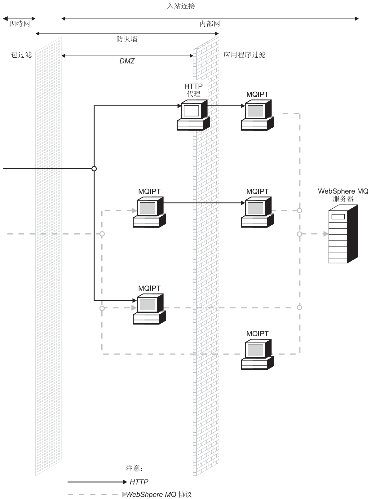
图 5. WebSphere MQ 拓扑结构显示了可能的 MQIPT 配置 (2/2)
