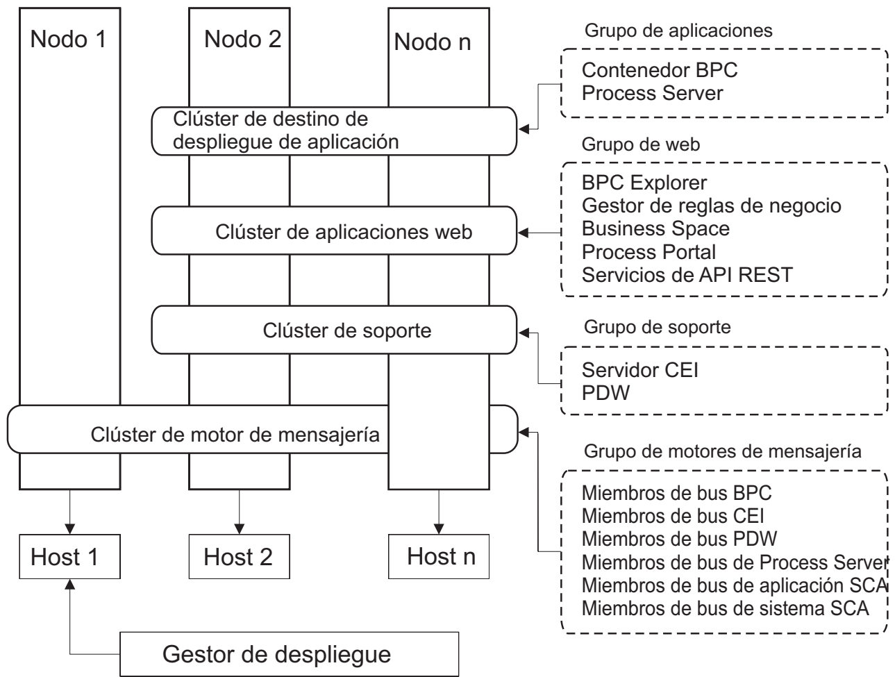
Figura 7. Patrón de topología Mensajería remota, Soporte remoto y Web
