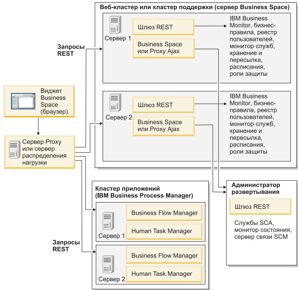
Рисунок 1. Типичная топология
