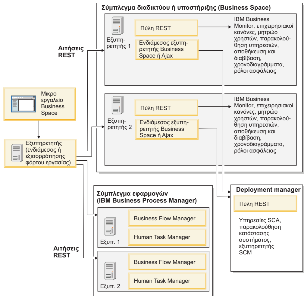
Σχήμα 1. Τυπική τοπολογία
