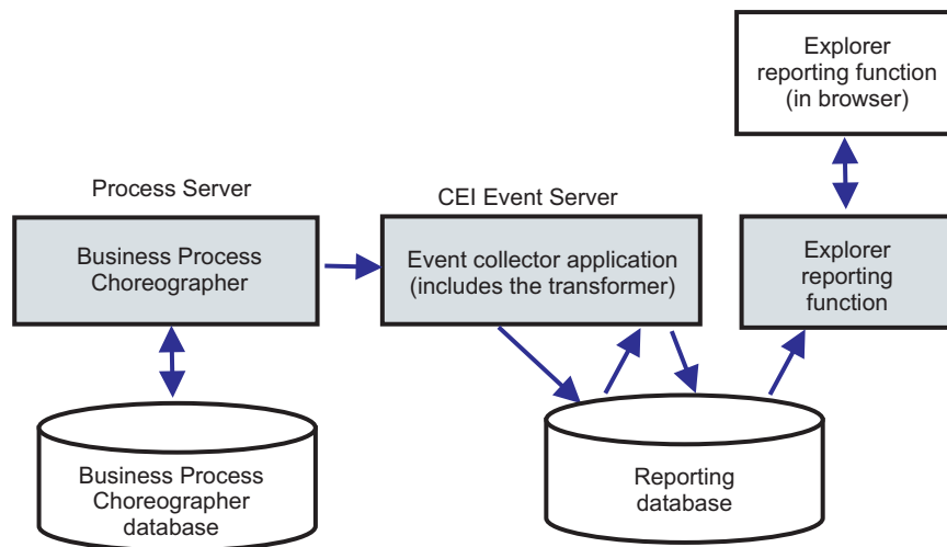
Abbildung 10. Berichtskonfiguration von Business Process Choreographer Explorer für hohe Produktionsleistung
