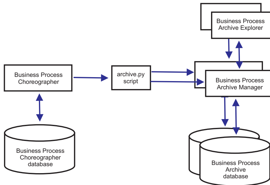
Abbildung 12. Business Process Choreographer verwendet zwei Business-Prozessarchive
