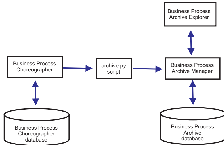
Abbildung 11. Business Process Choreographer verwendet ein Business-Prozessarchiv
