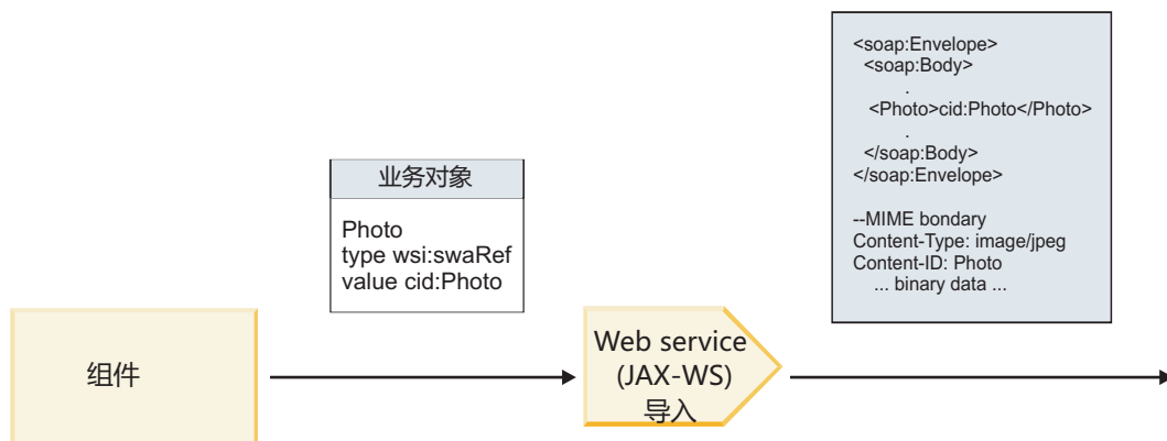
图 62. Web Service (JAX-WS) 导入绑定生成包含 swaRef 附件的 SOAP 消息的方式
