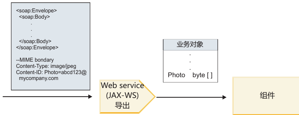
图 64. Web Service (JAX-WS) 导出绑定处理带有所引用附件并与 WS-I 一致的 SOAP 消息的方式
