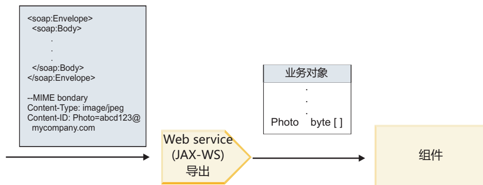
图 58. Web Service (JAX-WS) 导出绑定处理引用了附件的 SOAP 消息的方式
