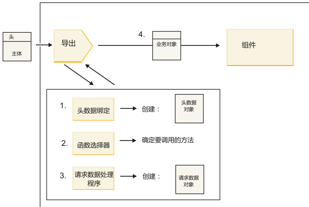
图 48. 通过导出的组件请求流
