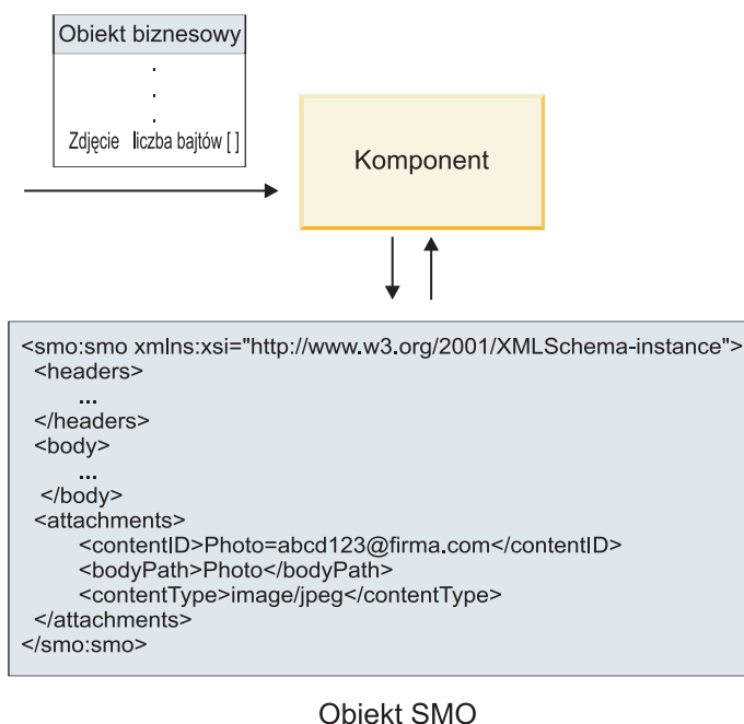
Rysunek 20. Sposób wyświetlania załączników przywoływanych w obiekcie SMO
