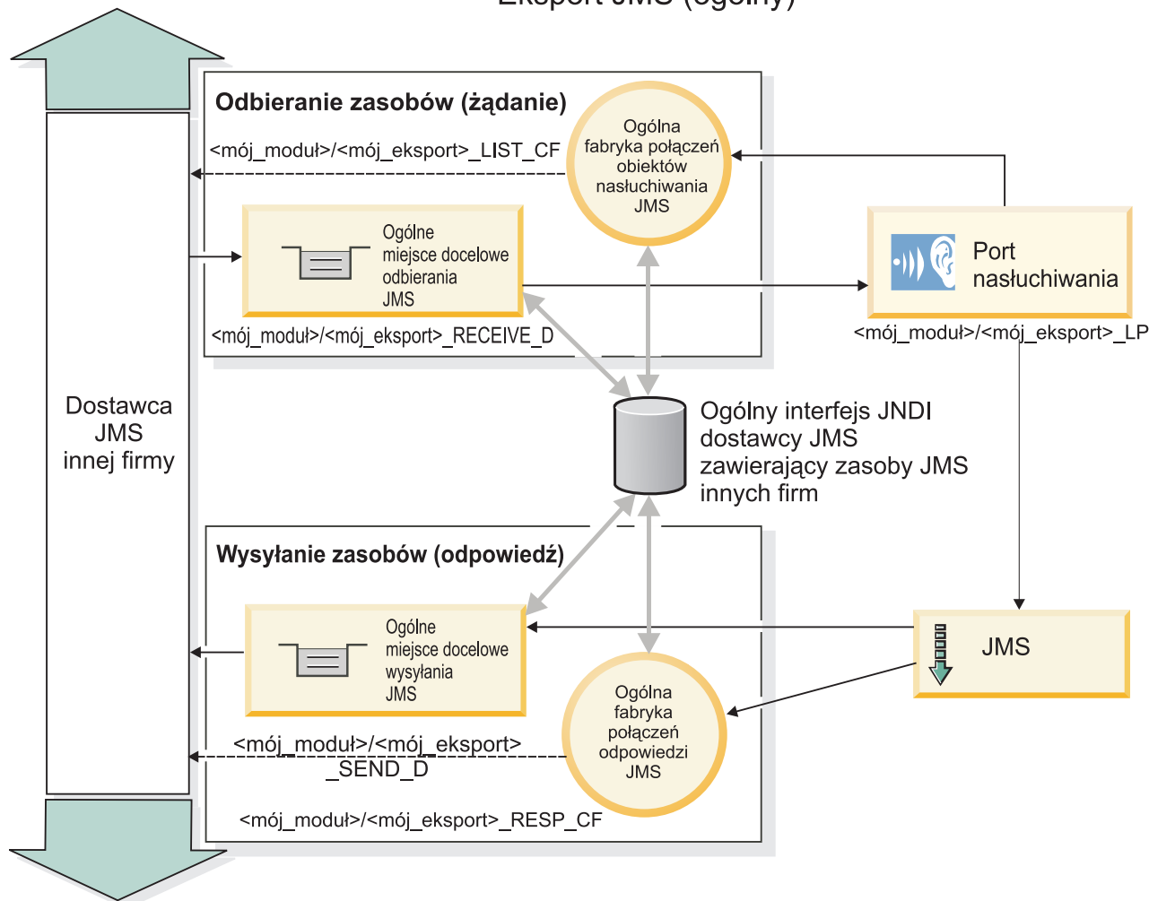
Rysunek 36. Zasoby ogólnego powiązania eksportu JMS
