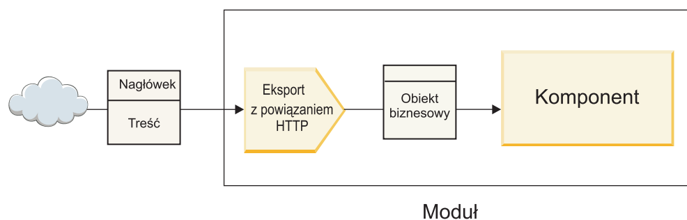
Rysunek 46. Eksport z powiązaniem HTTP
