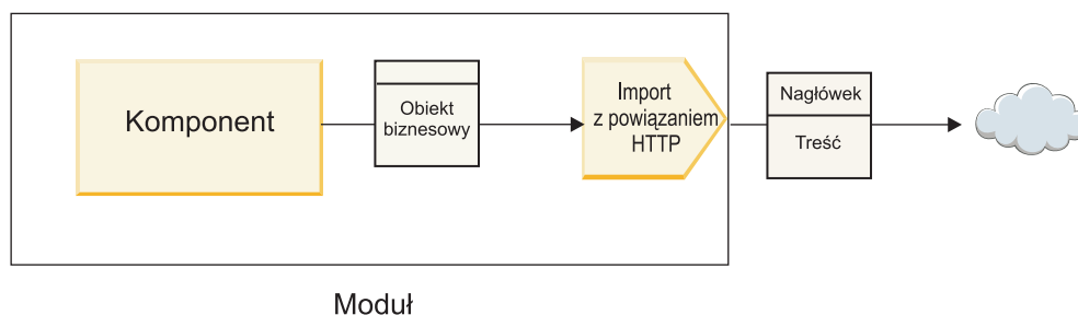
Rysunek 2. Import z powiązaniem HTTP
