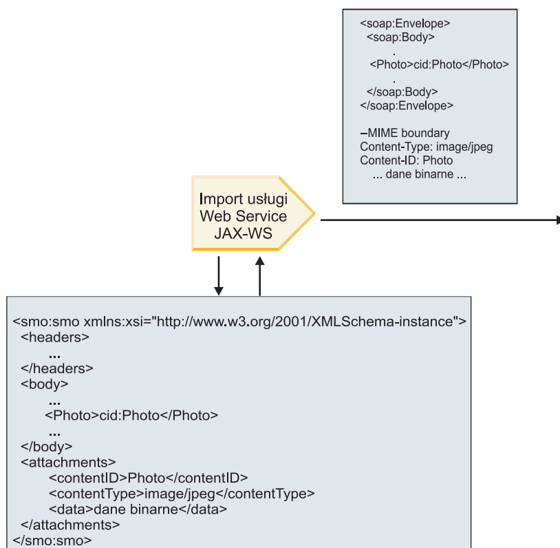
Rysunek 63. Sposób dostępu do załącznika swaRef w obiekcie SMO w celu utworzenia komunikatu SOAP
