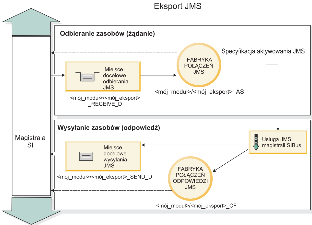
Rysunek 78. Zasoby powiązania eksportu JMS
