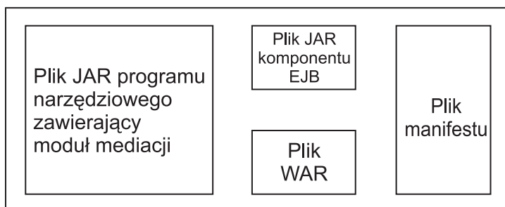
Rysunek 89. Uproszczony przykład pliku EAR zawierającego moduł mediacji. Plik EAR zawiera pliki JAR. Plik programu narzędziowego JAR zawiera moduł mediacji.
