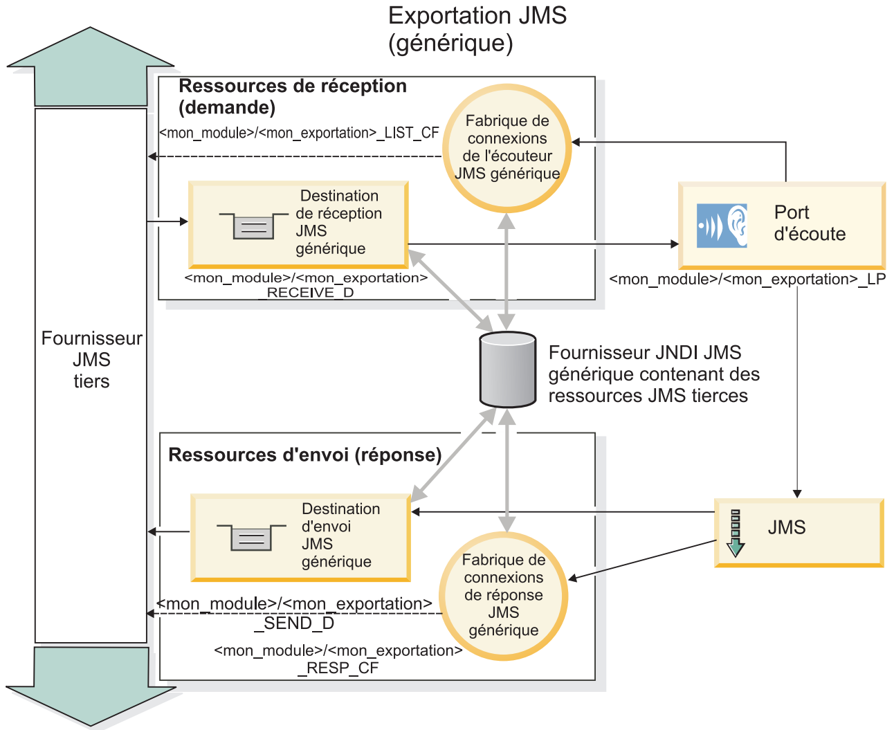
Figure 81. Ressources de liaisons d'exportation JMS génériques
