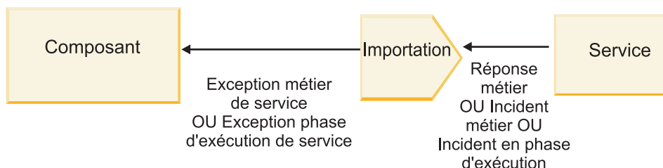
Figure 55. Manière dont les informations d'erreur sont envoyées depuis le service au composant via l'importation
