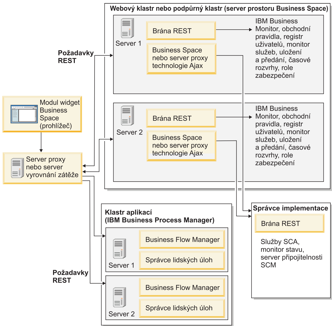
Obrázek 1. Typická topologie
