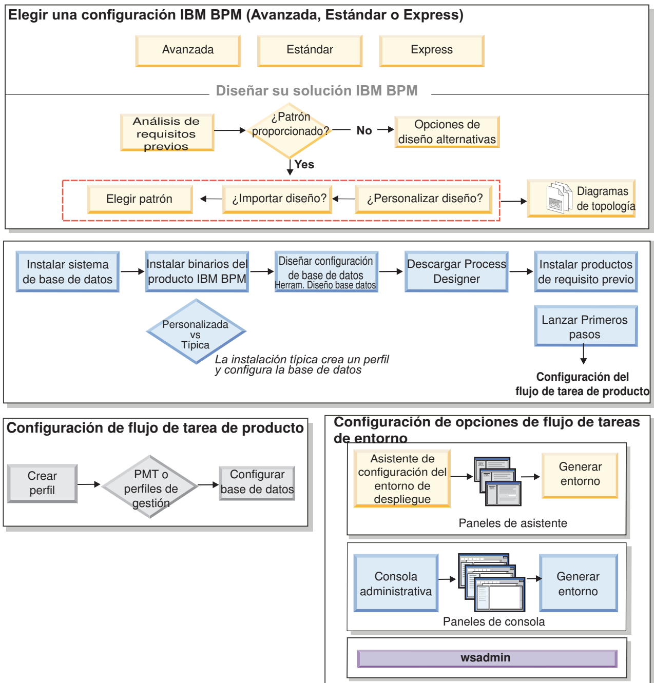
Figura 13. El flujo de tareas de la planificación, instalación y configuración el producto y el entorno
