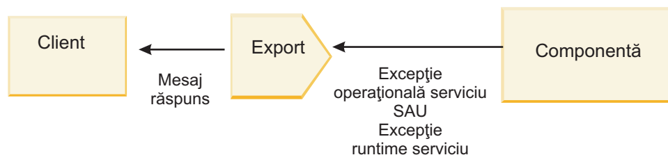
Figura 8. Cum sunt trimise informațiile despre defect de la componentă prin legarea de export clientului
