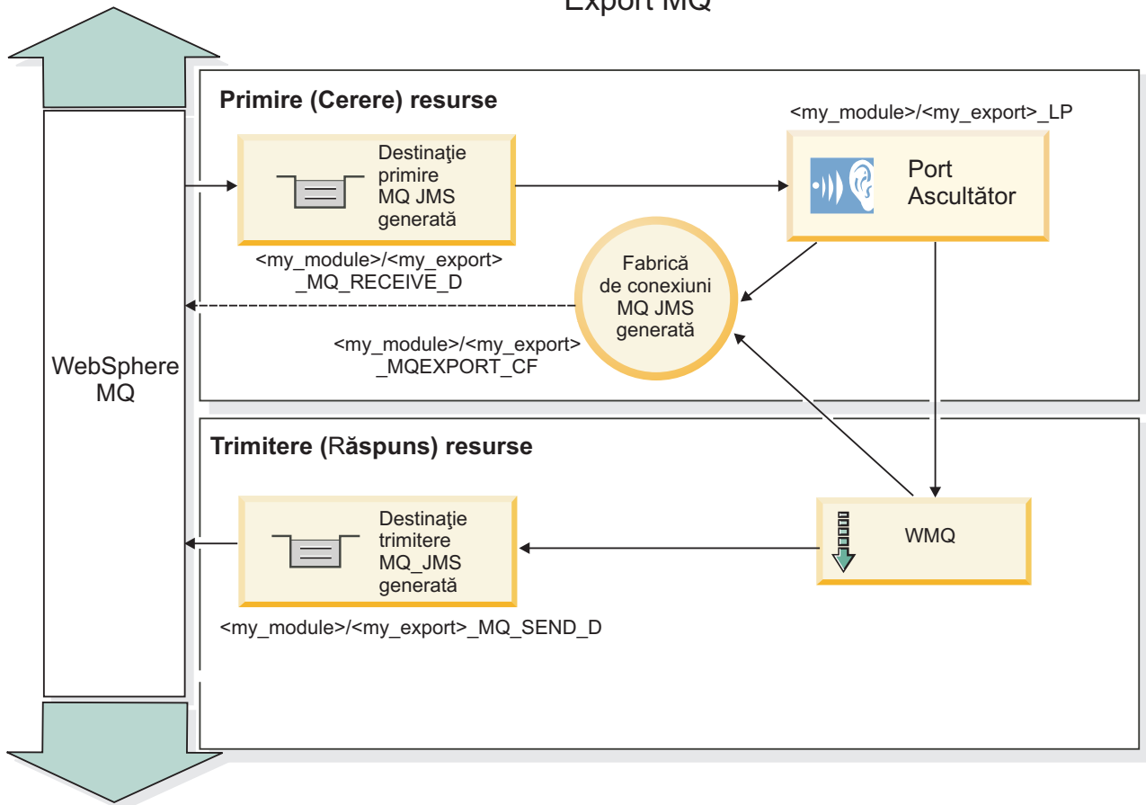
Figura 40. Resurse pentru legarea de export WebSphere MQ
