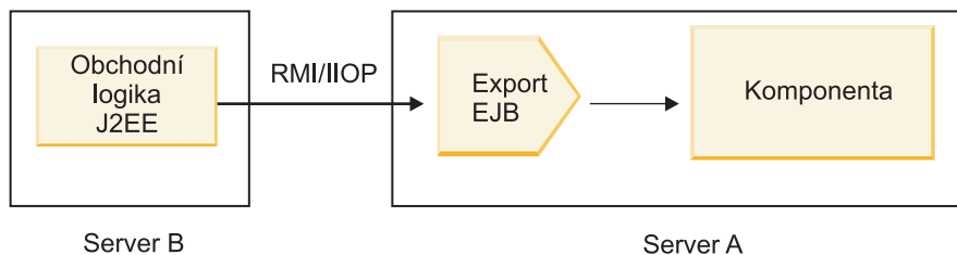
Obrázek 30. Vzdálené volání z klienta do komponenty SCA prostřednictvím exportu EJB
