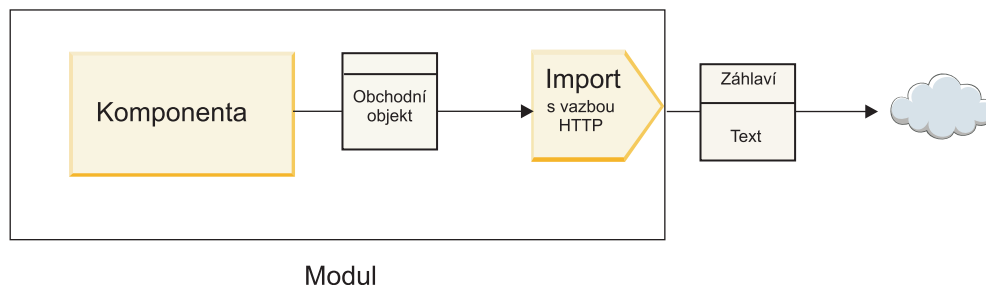
Obrázek 2. Import s vazbou HTTP
