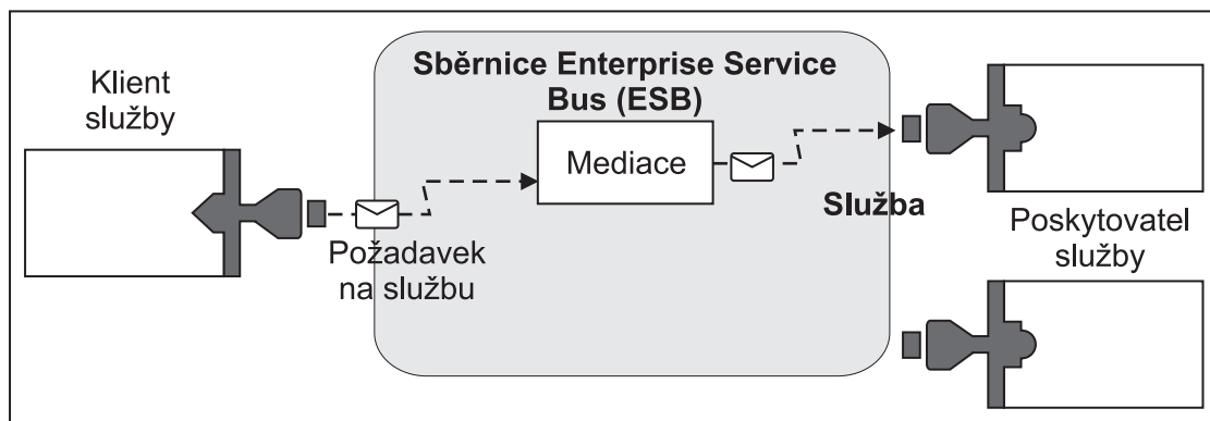
Obrázek 42. Sběrnice Enterprise Service Bus. Sběrnice Enterprise Service Bus trasuje zprávy mezi aplikacemi, které jsou klienty nebo poskytovateli služeb. Sběrnice převádí přenosové protokoly a transformuje formát zpráv mezi žadateli a poskytovateli. Na tomto obrázku používá každá aplikace jiný protokol (reprezentovaný jiným geometrickým tvarem konektoru) a jiný formát zpráv.
