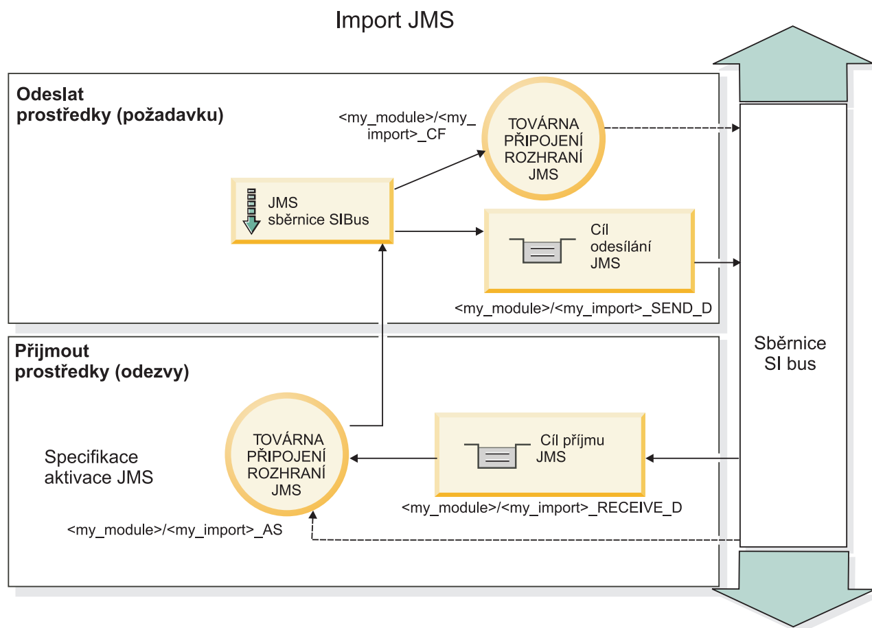
Obrázek 32. Prostředky vazby importu JMS
