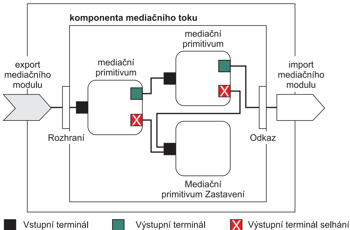
Obrázek 43. Zjednodušený příklad mediačního modulu. Mediační modul obsahuje jednu komponentu mediačního toku, která obsahuje mediační primitiva.
