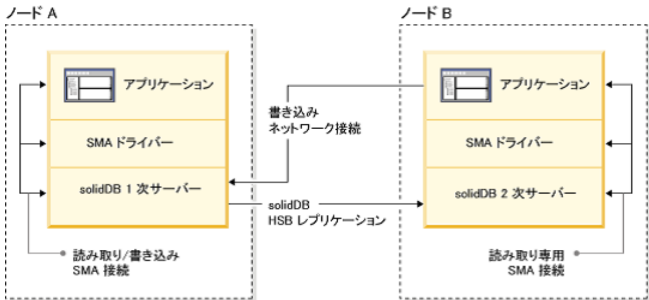
図3. ホット・スタンバイを使用する SMA 透過接続性のアーキテクチャー
