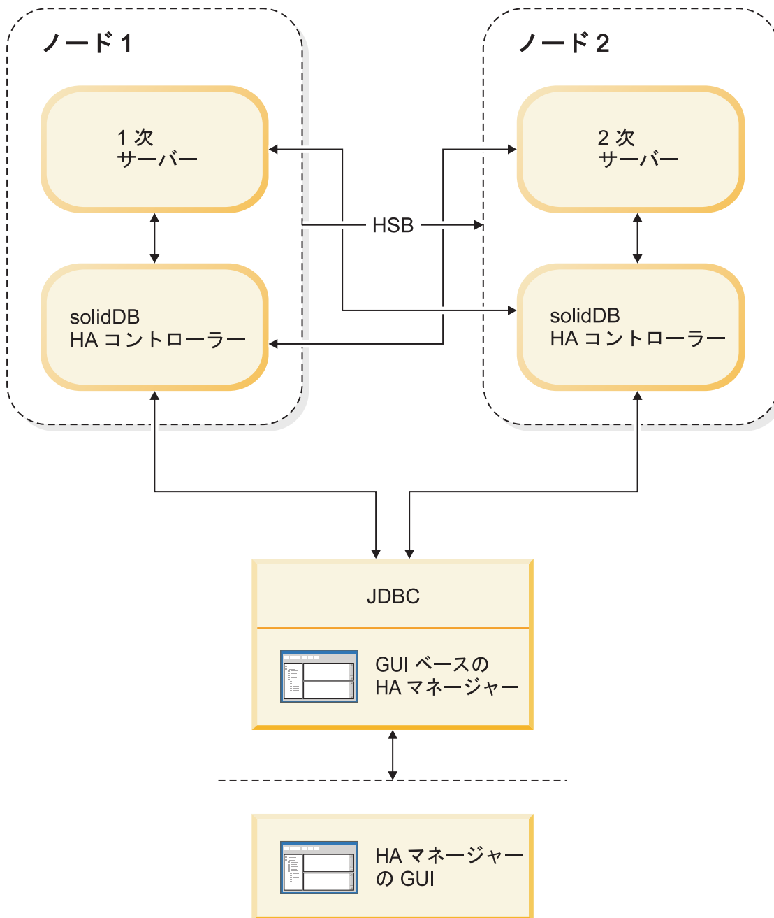
図 8. 高可用性コントローラーのアーキテクチャー
