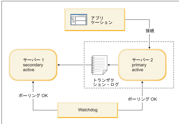
図 21. 1 次サーバーがダウンしたシナリオと修復方法
