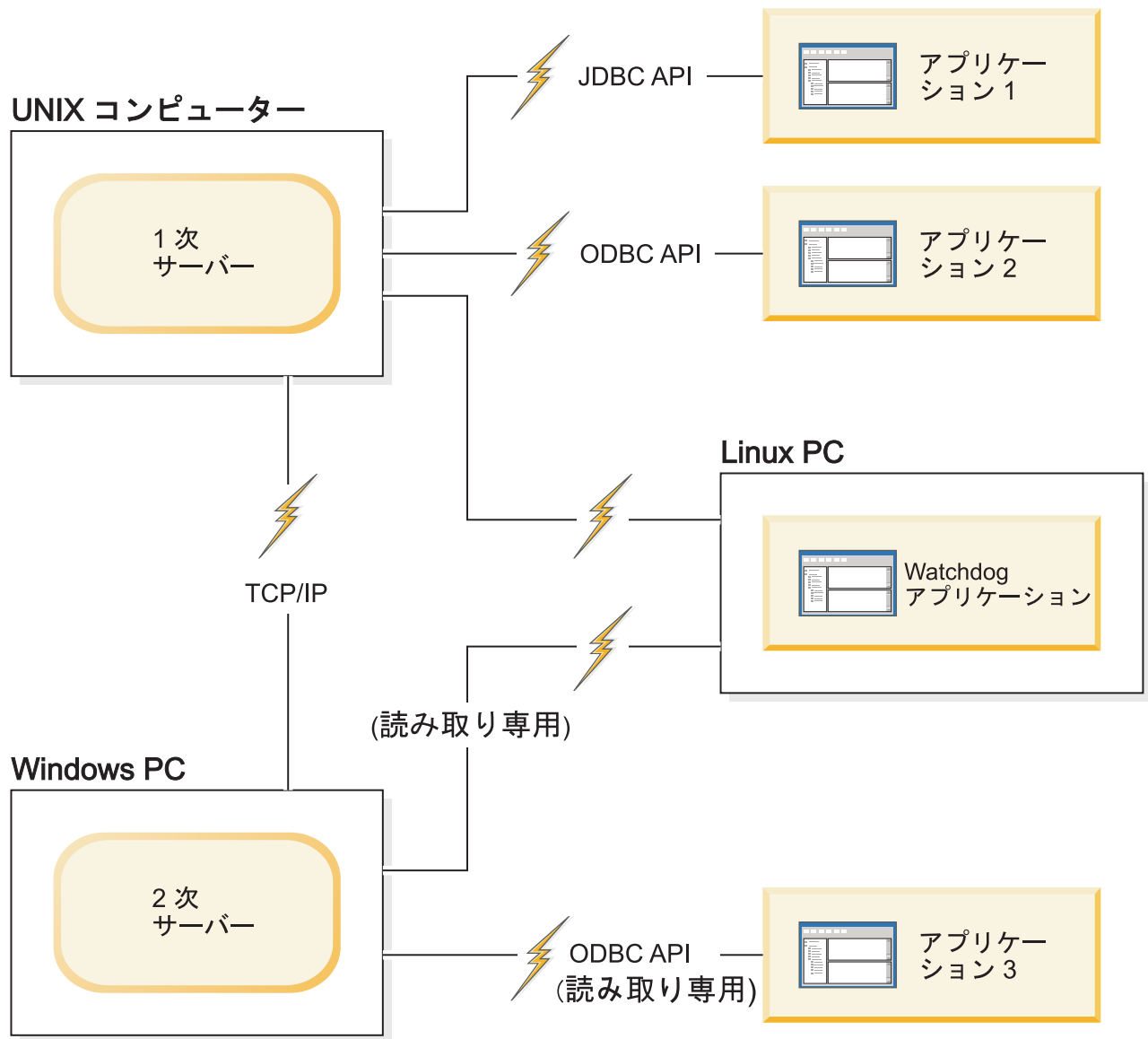
図 20. Watchdog を使用した異機種混合 HotStandby 構成
