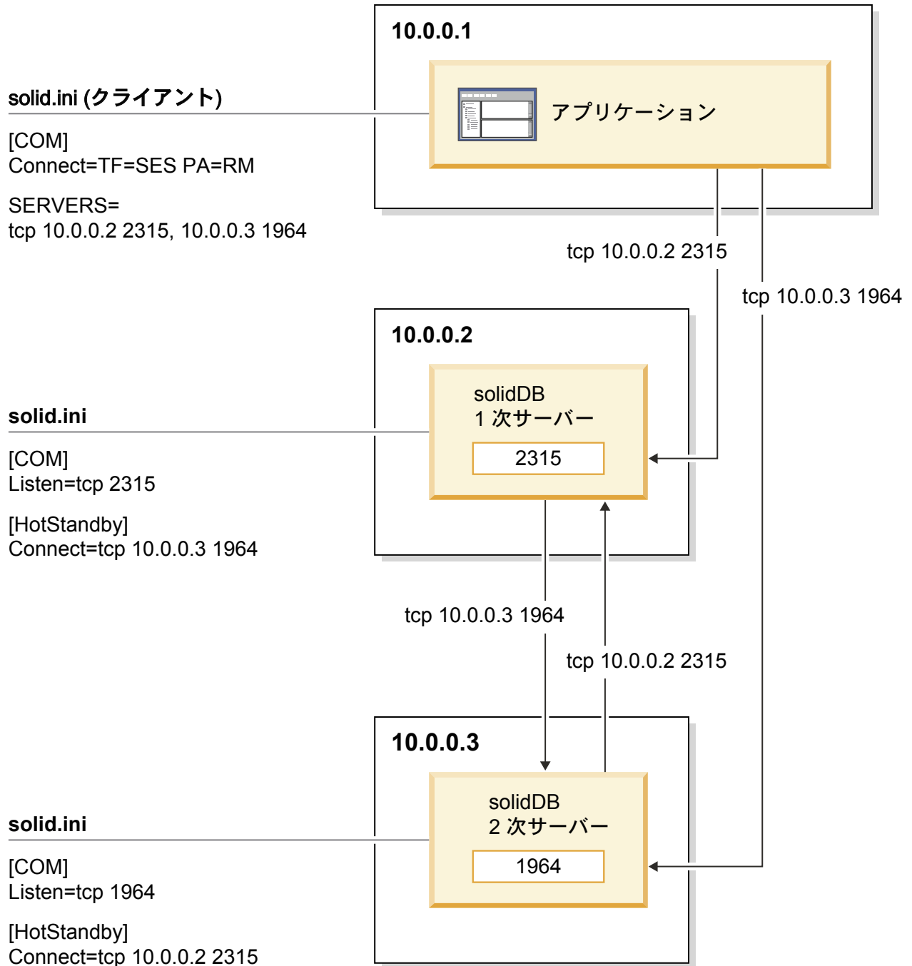
図 14. 例: TC 接続
