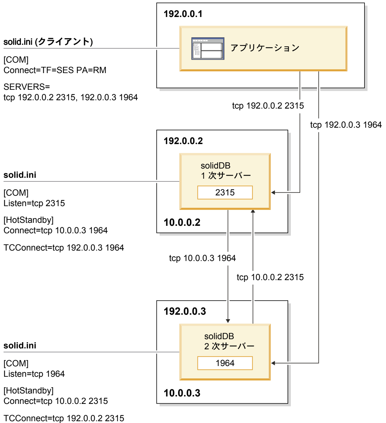
図 15. 例: マルチホーム・サーバーを使用した TC 接続
