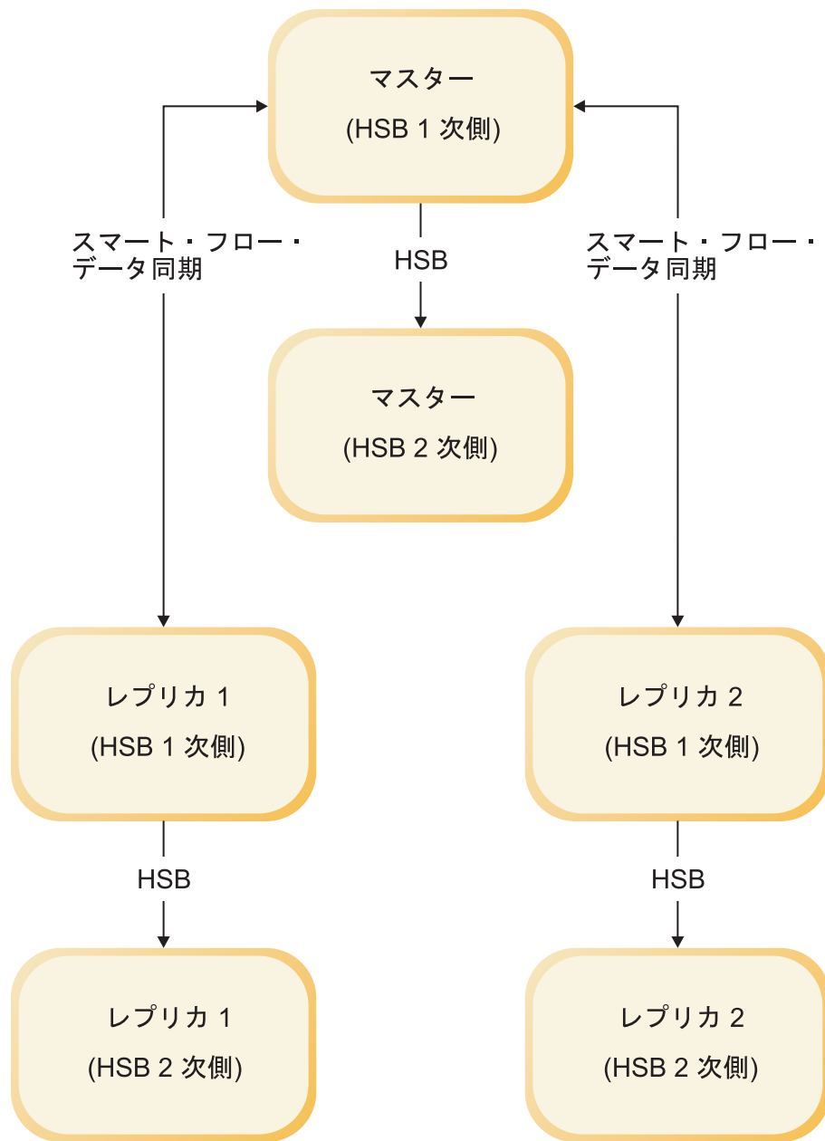
図7. マスターおよびレプリカ・サーバー・スキームでの HotStandby
