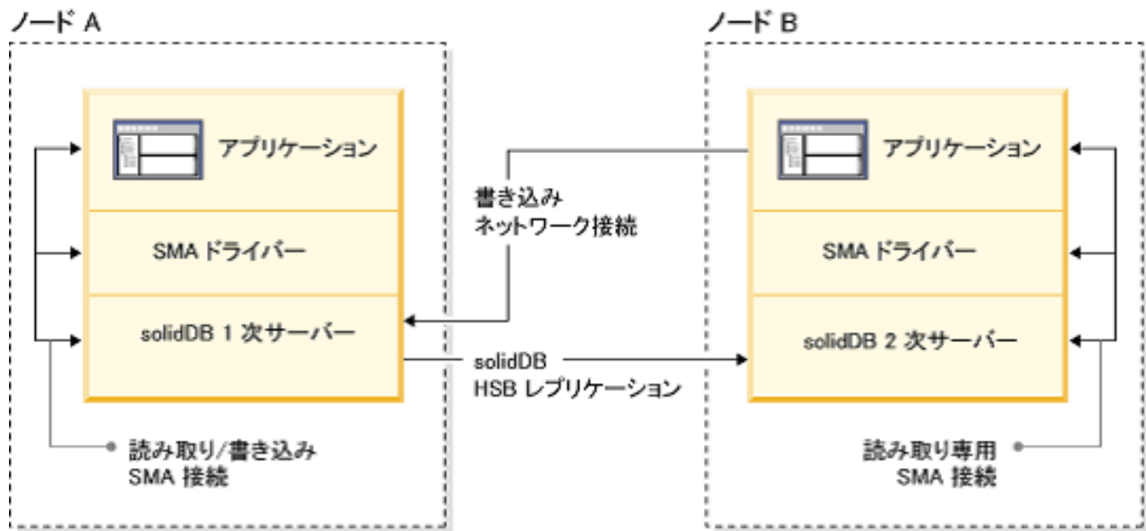
図6. ホット・スタンバイを使用する SMA 透過接続性のアーキテクチャ
