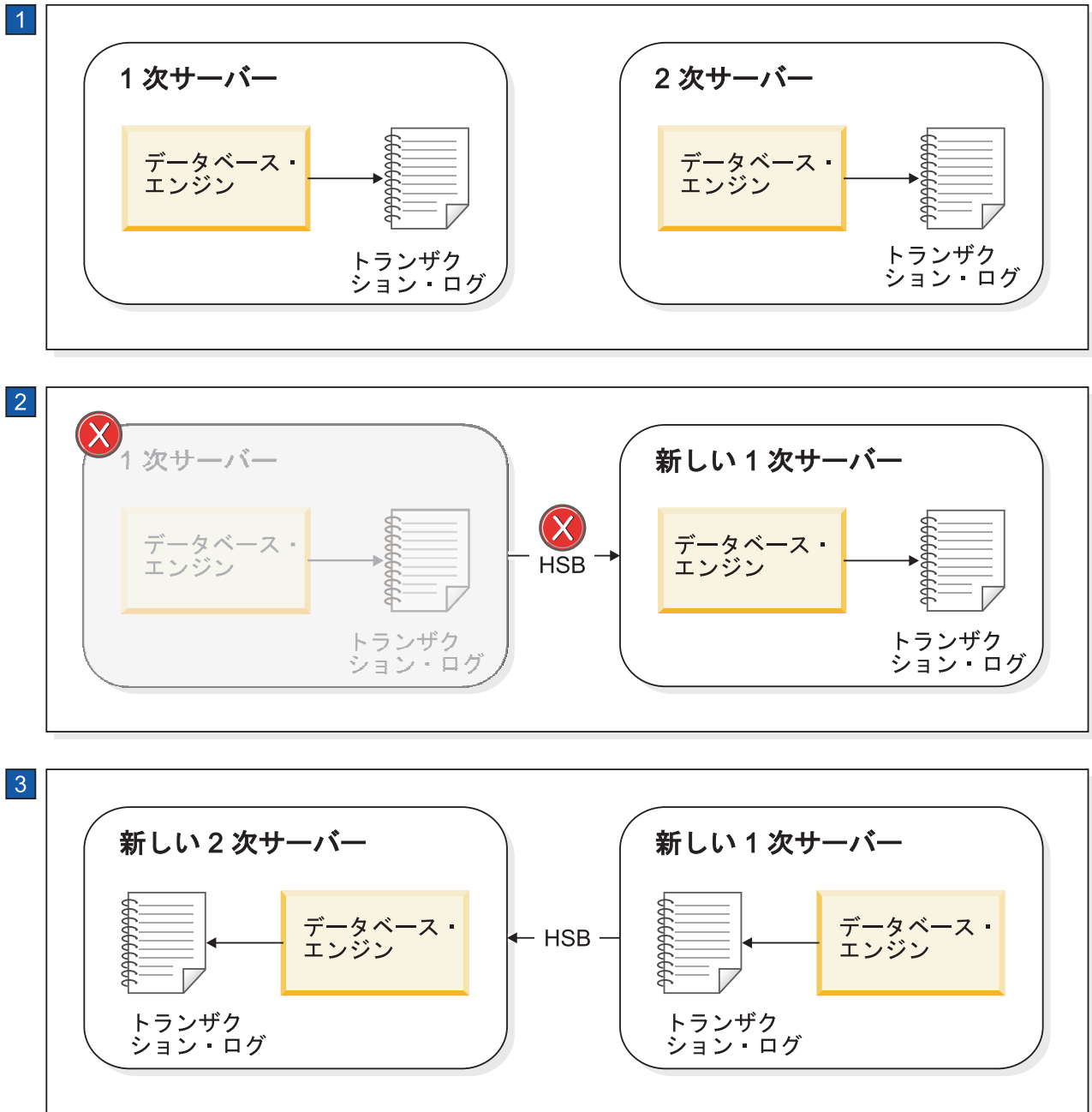
図4. サーバーのフェイルオーバーとキャッチアップの例
