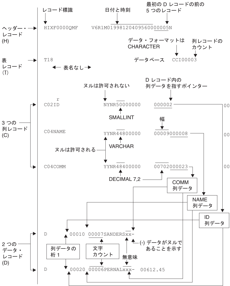
図 71. サンプル IXF レコードのフォーマット (OUTPUTMODE=CHARACTER)
