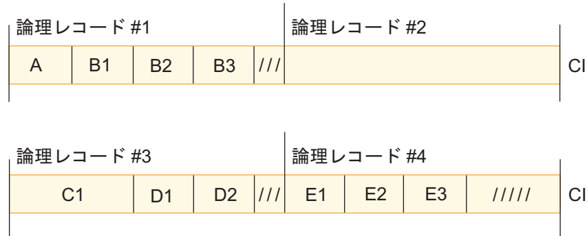
図 227. 2 つの読み取り操作が必要になる論理レコードの例
