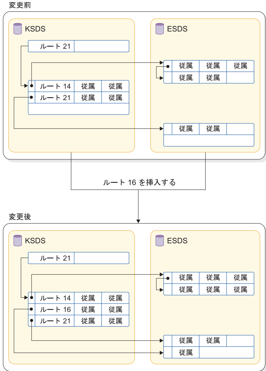
図 27. HISAM データベースへのルート・セグメントの挿入 (CI の中に空き論理レコードが存在する場合)
