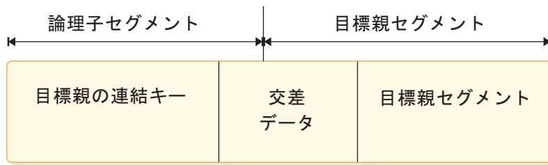
図 86. ユーザー入出力域に戻される連結セグメントのフォーマット
