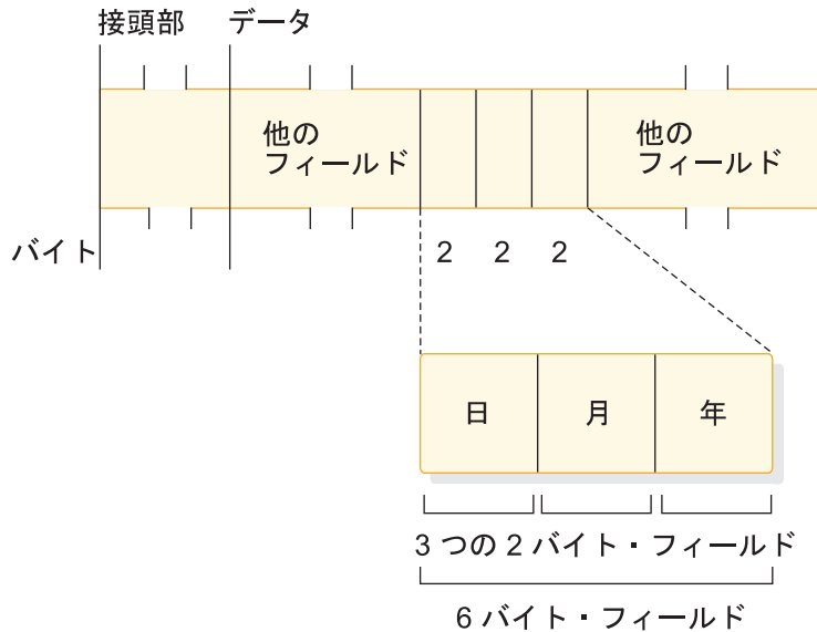
図 232. セグメント内の日付フィールドが、3 つの 2 バイト・フィールド、かつ 1 つの 6 バイト・フィールドとして定義されている例
