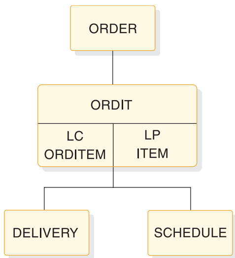
図 95. シンボリック・ポインターを使用する単方向関係のための論理データ構造
