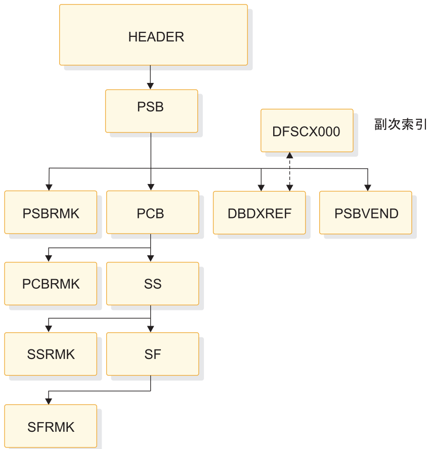
図 19. プログラム仕様ブロックの IMS カタログ・レコードのフォーマット
