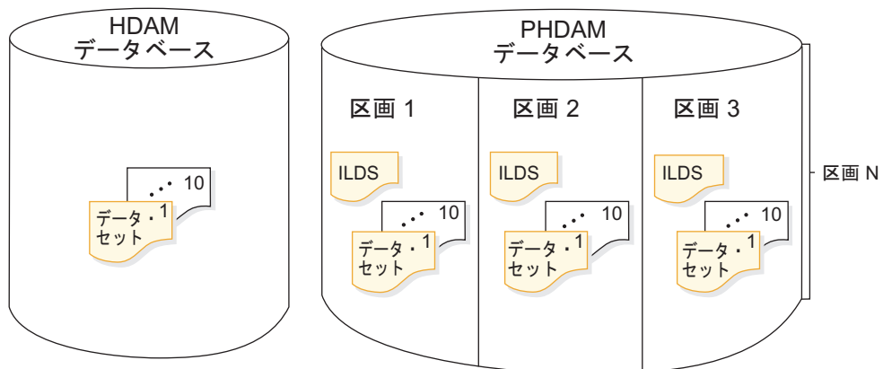
図 33. HDAM データベースと PHDAM データベースの論理ビューの比較
