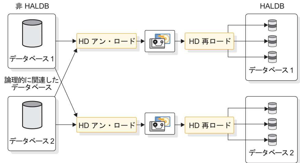
図 310. 論理関係を持つデータベースのマイグレーション
