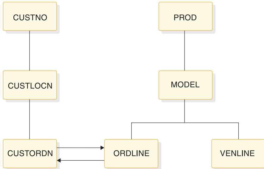
図 73. 2 つの親を持つように見えるセグメントの例
