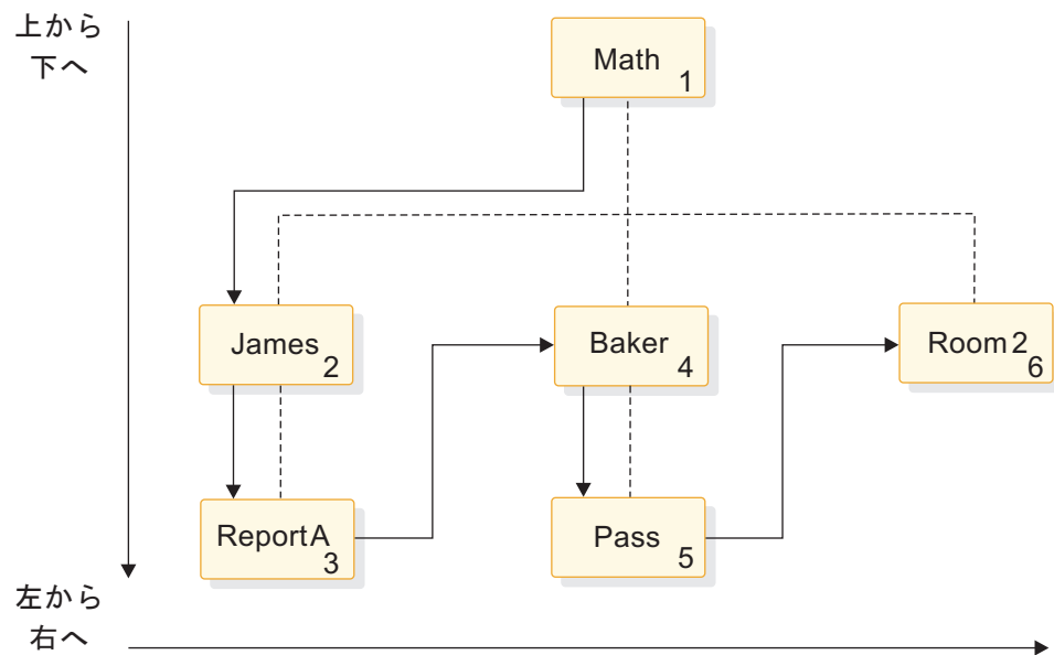
図 3. 学校用データベースのセグメント・タイプの階層順
