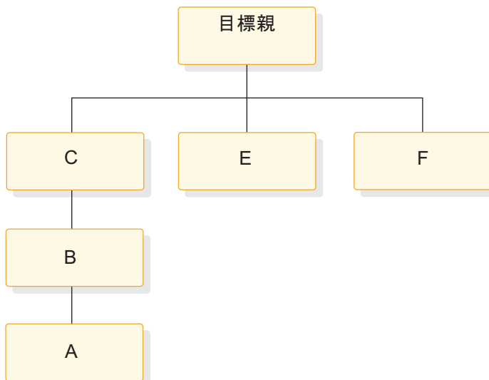
図 98. 最初の論理関係の交差によって可能となった論理データベース階層
