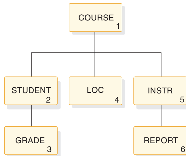
図 209. INSTR および LOC セグメントをアクセスする必要があるアプリケーションのための階層
