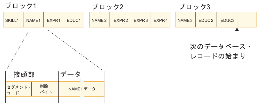
図 21. ブロックに保管された HSAM データベース
