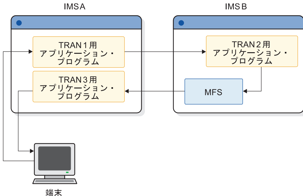
図 56. ISC VTAM で IMS から IMS へ
