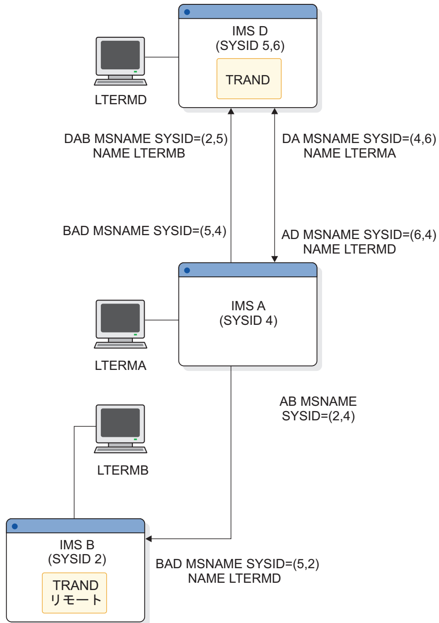
図 117. リモート LTERM
