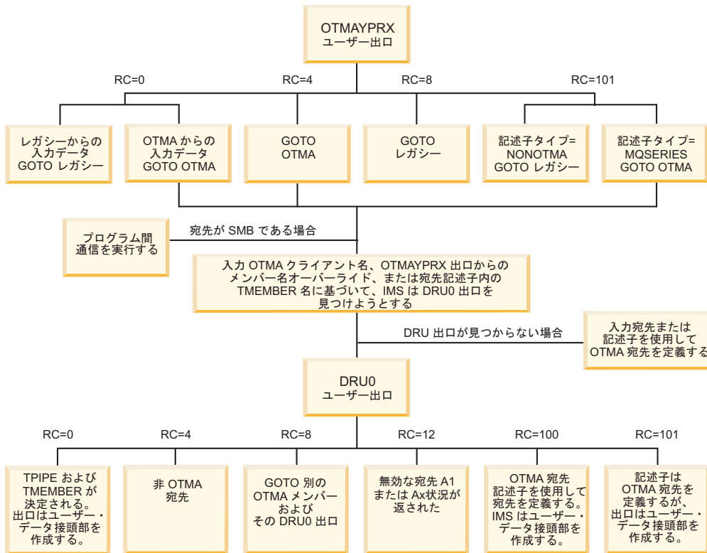
図 136. OTMAYPRX OTMA ユーザー出口および DFSYDRU0 OTMA ユーザー出口のメッセージ宛先の決定方法
