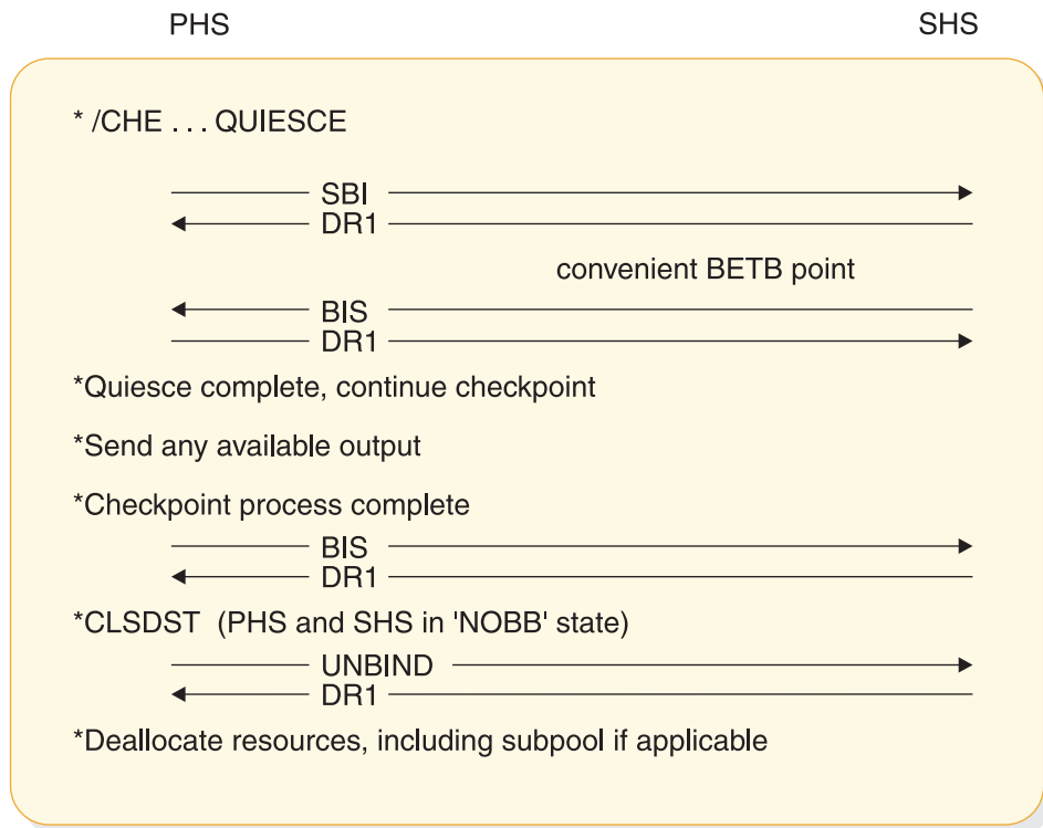
図 98. SBI/BIS を使用した PHS のシャットダウンの例
