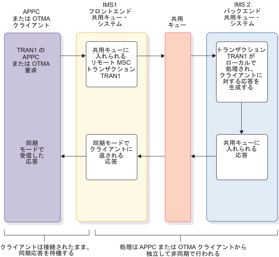
図 121. リモート MSC トランザクションを使用した、APPC または OTMA トランザクションのバックエンド IMS システムへの経路指定
