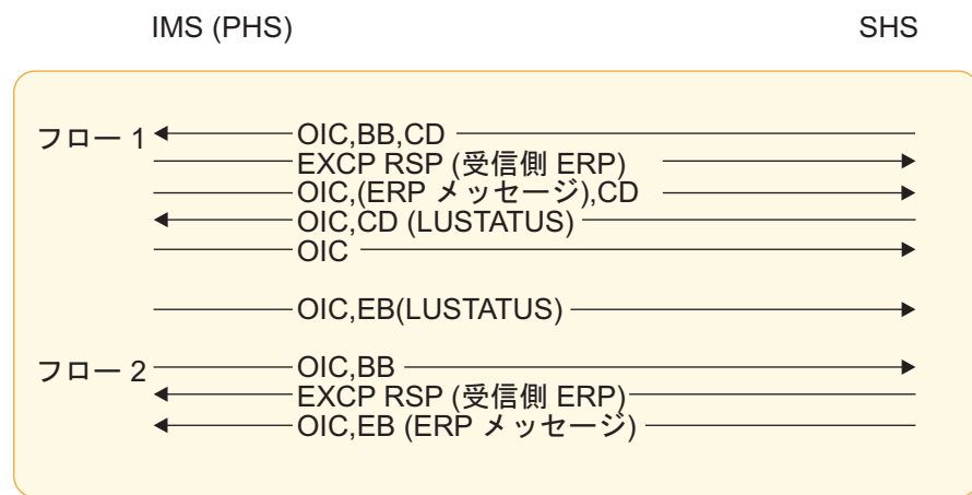
図 106. MULT1 として定義された IMS コンポーネントの受信側 ERP の例
