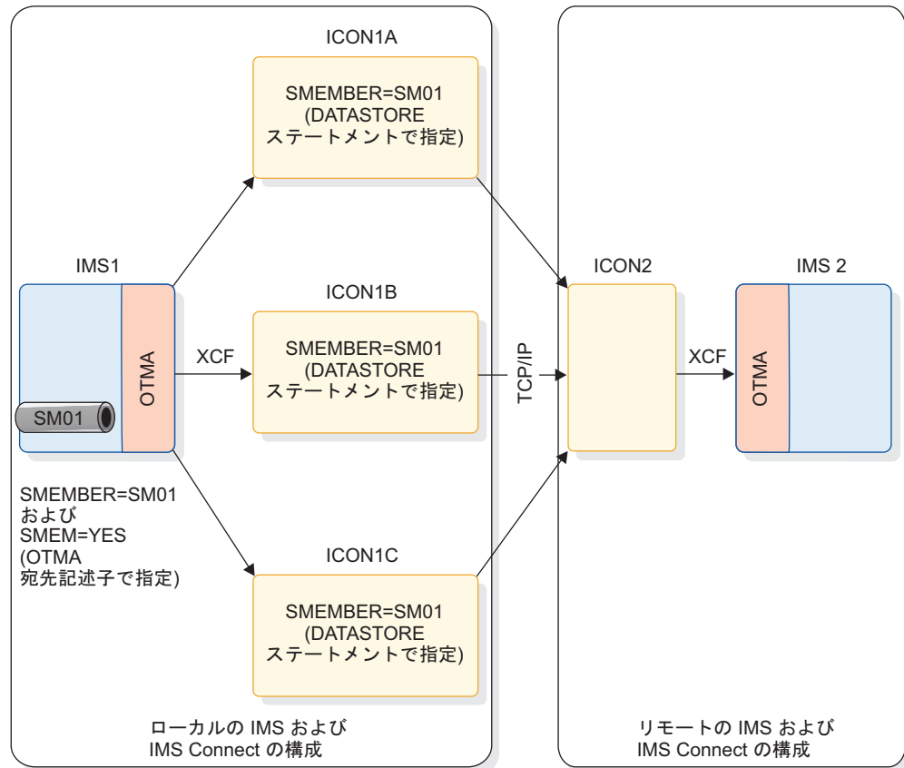
図 135. OTMA IMS 間 TCP/IP 接続でのスーパー・メンバー・グループの使用
