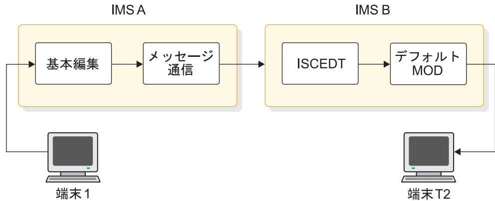
図 61. IMS 端末間メッセージ通信経路指定の ISC 例
