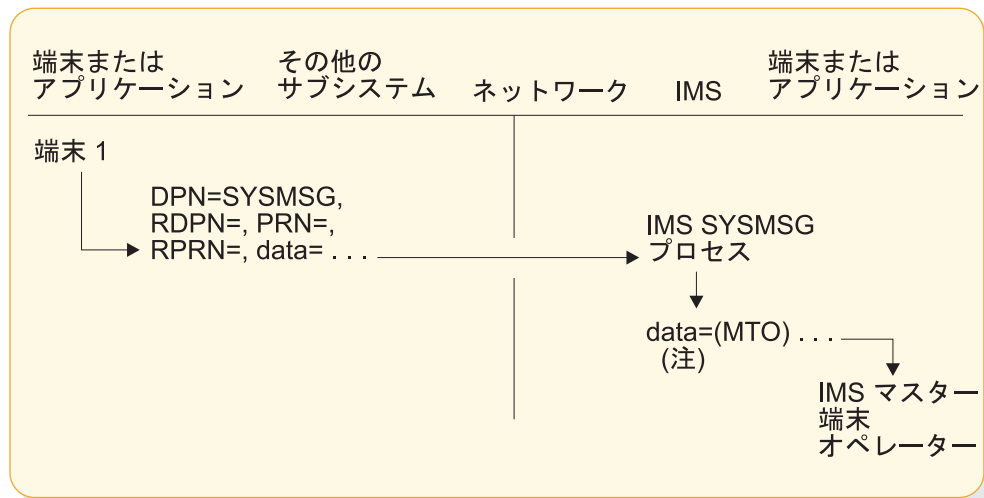
図 72. 他のサブシステム端末から IMS A への PRN のない SYSMMSG の例
