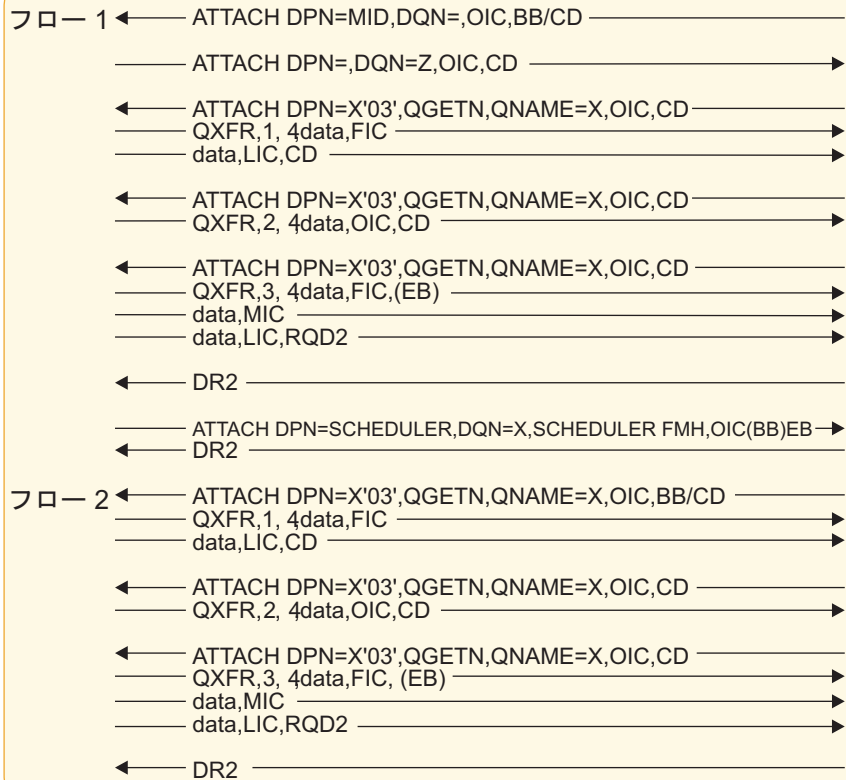
図 91. 例 1: 要求時ページ化出力、定義されていないオペレーター論理ページング (OLP)、QGETN FM ヘッダーによる順次リトリーブ
