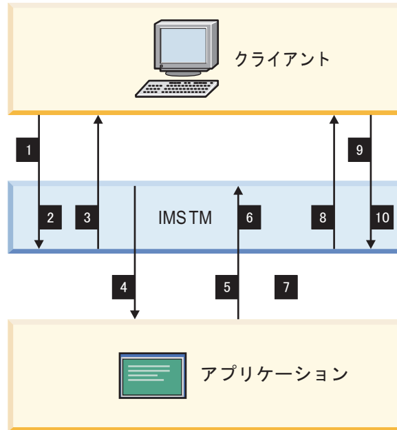
図 142. コミット後送信 (IMS 標準) フロー
