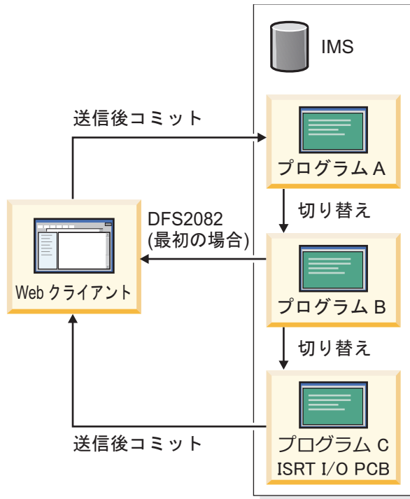
図 139. 単一ストリームのプログラム間通信
