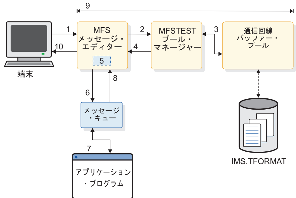
図 50. MFS テスト環境の概要
