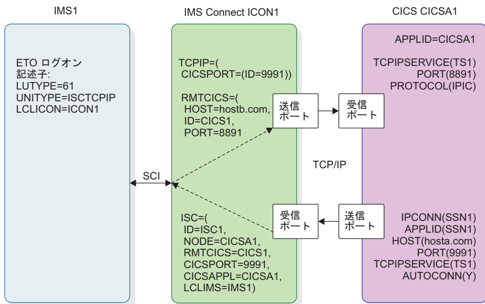
図 20. TCP/IP を使用する ISC 並列セッションに対する IMS Connect サポートの概要
