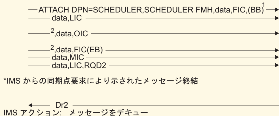
図 94. 自動ページ化出力の例
