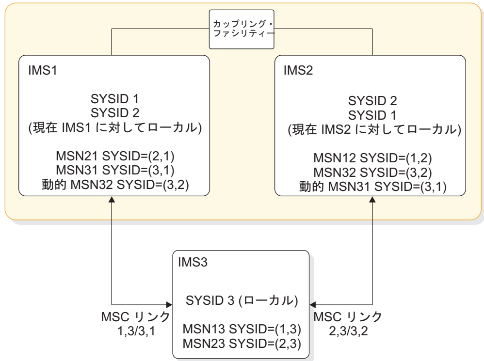
図 120. 共用キューを使用する IMSplex と共存する MSC ネットワーク
