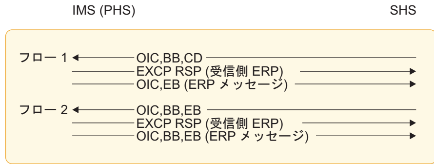
図 104. SINGLE1 として定義された IMS コンポーネントの受信側 ERP の例
