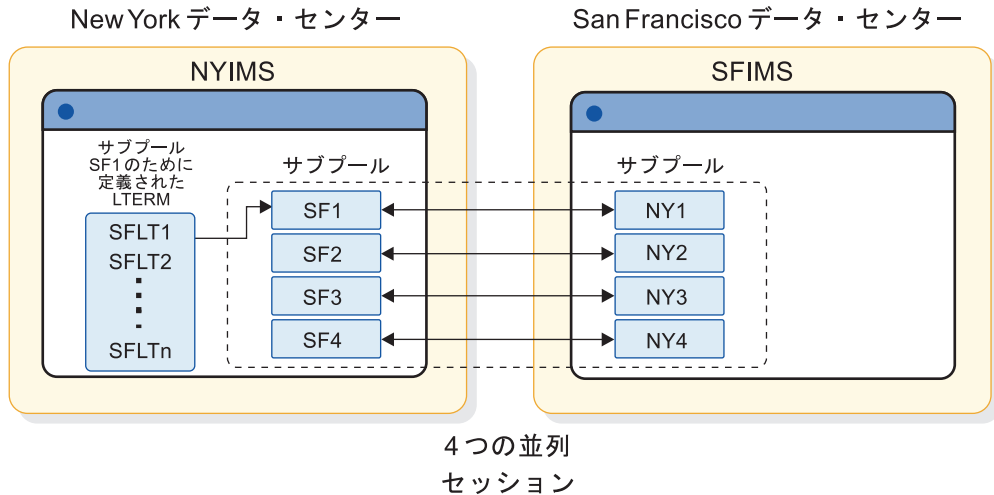
図 66. ISC ノードとして、お互いに定義された 2 つの IMS システム
