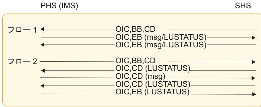
図 88. SINGLE2 として IMS に対して定義された PHS コンポーネントのブラケット・プロトコルの例
