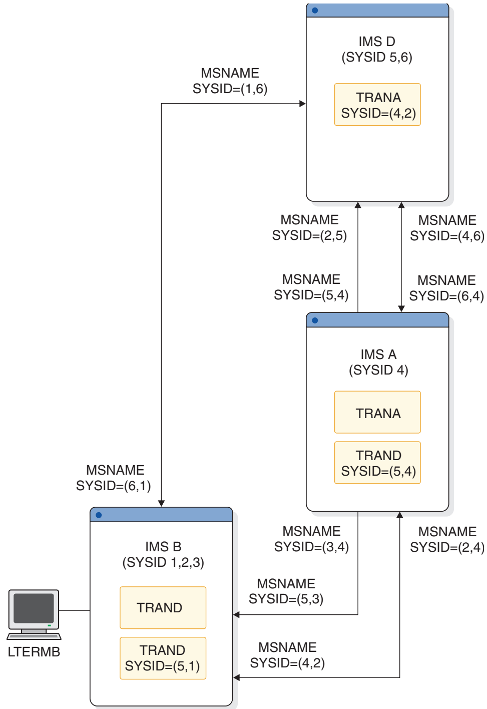
図 116. メッセージ経路指定
