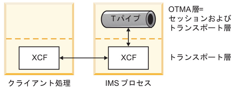
図 131. トランザクション・パイプを OTMA クライアント/サーバー環境に適合させる方法
