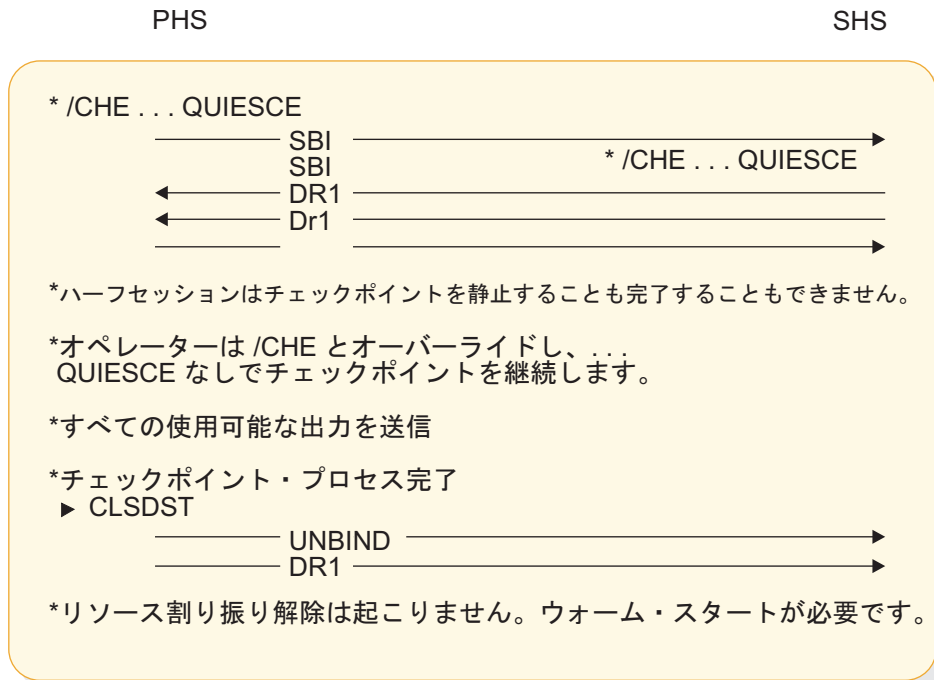
図 100. オペレーターによるオーバーライドが原因で障害が起こる、SBI/BIS を使用した PHS と SHS の同時シャットダウンの例
