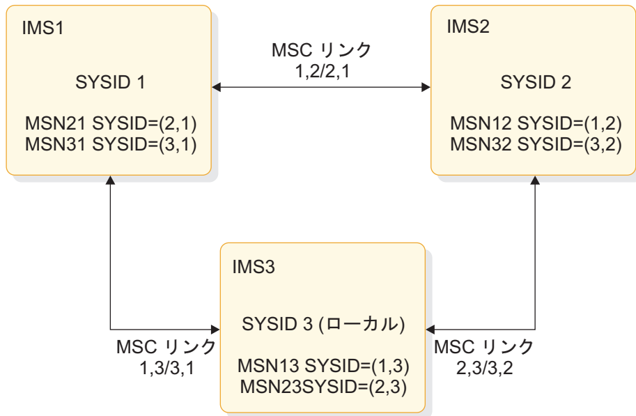
図 119. IMSplex を持たない MSC ネットワーク
