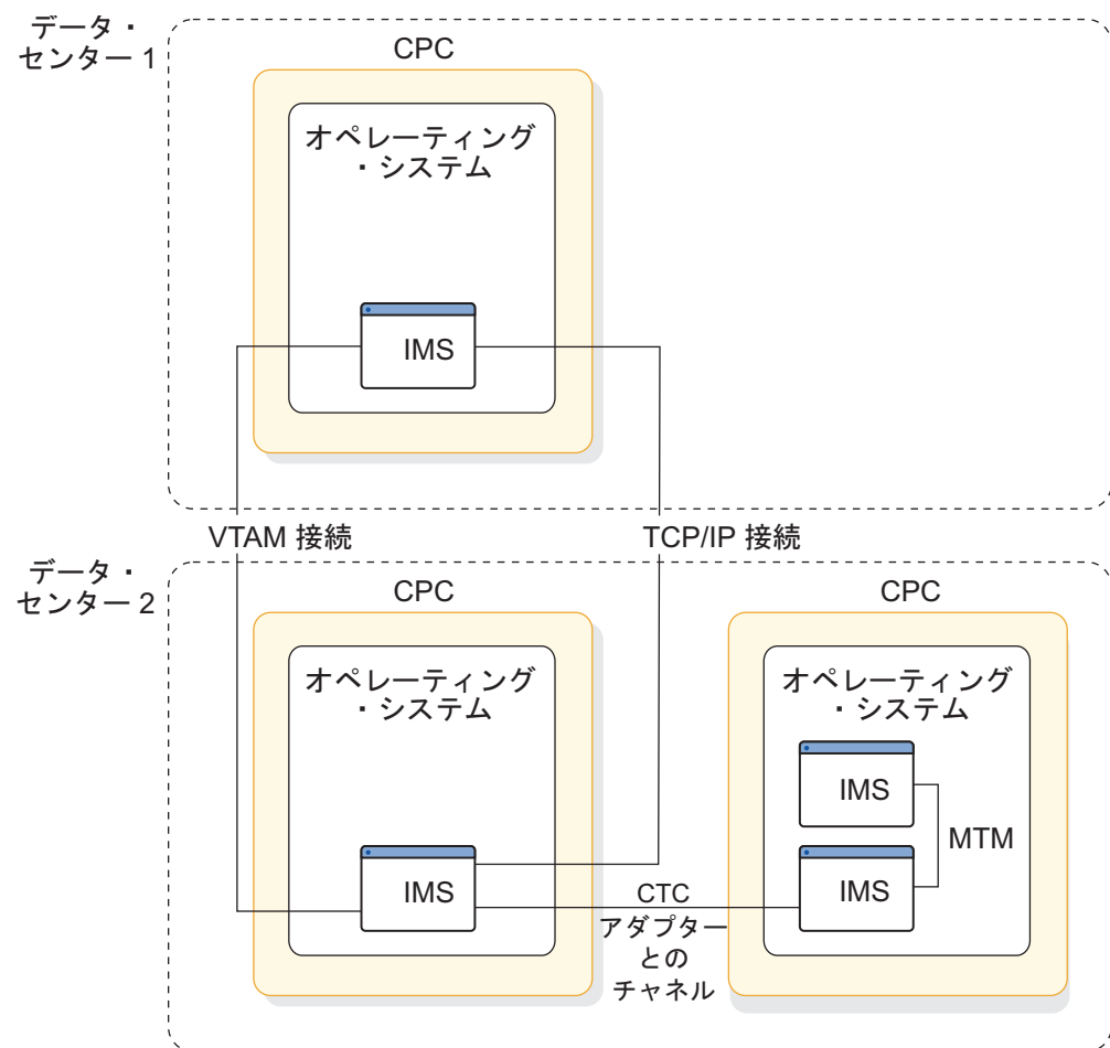
図 109. MSC 物理リンク・タイプ
