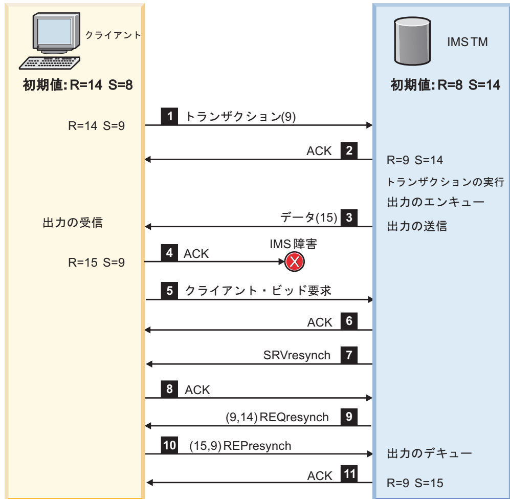
図 152. OTMA 再同期メッセージ・フローのサンプル
