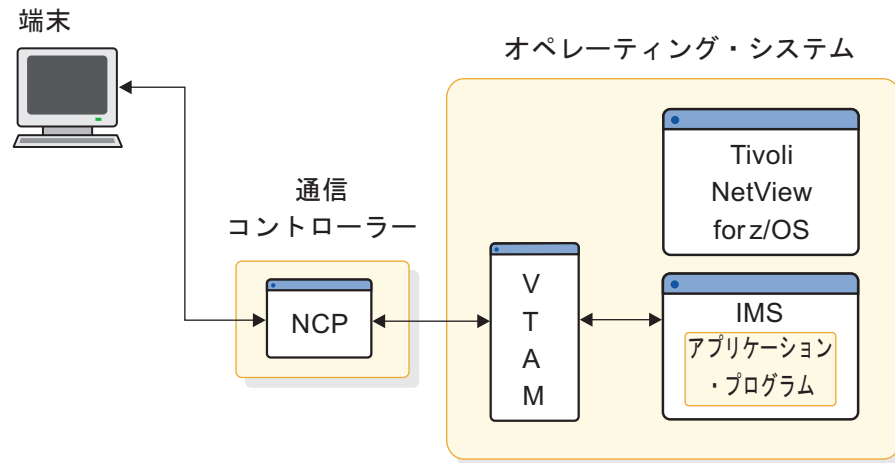
図 40. ネットワークのコンポーネント
