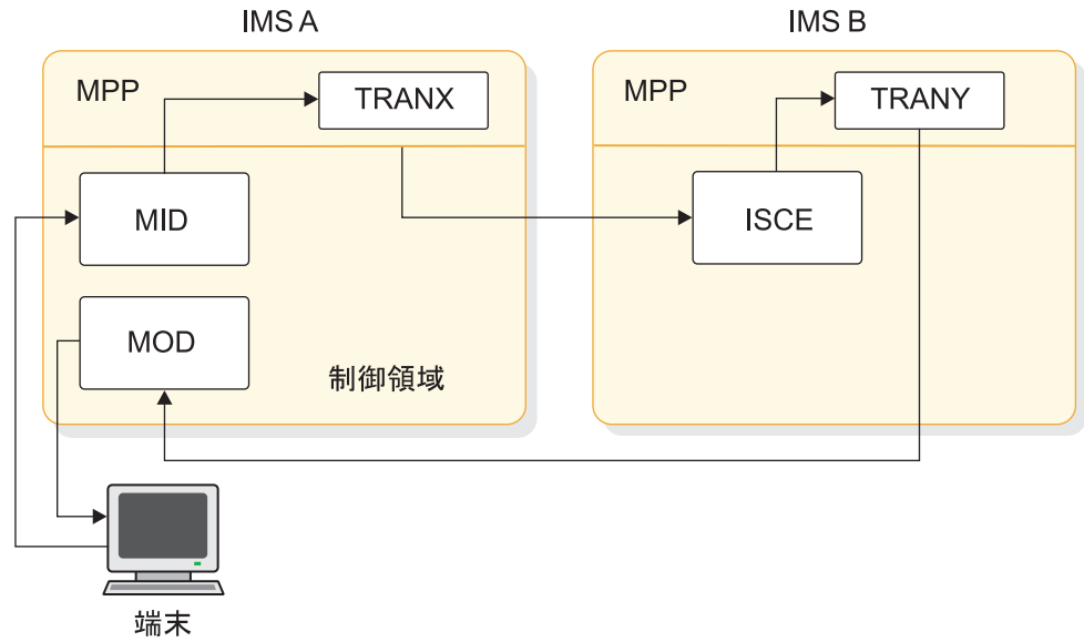
図 64. MFS での IMS 間アプリケーション経路指定の ISC 例
