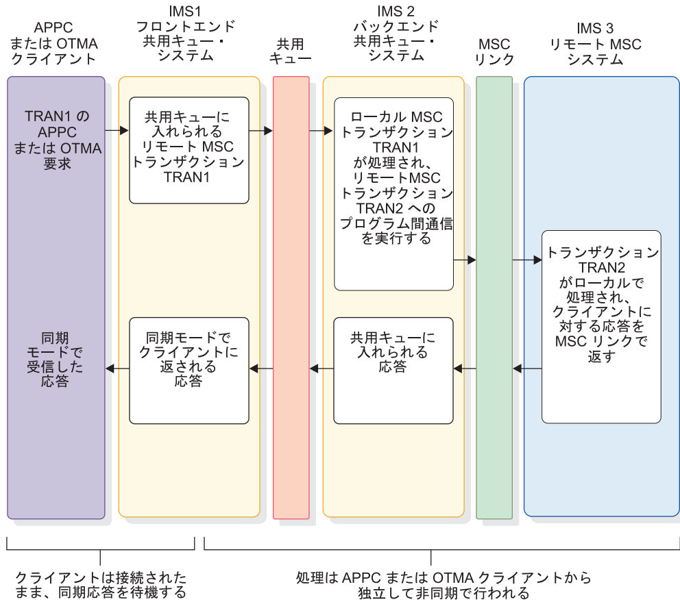
図 124. 1 つのプログラム間通信を伴う、MSC と共用キューを使用して経路指定される APPC または OTMA トランザクション
