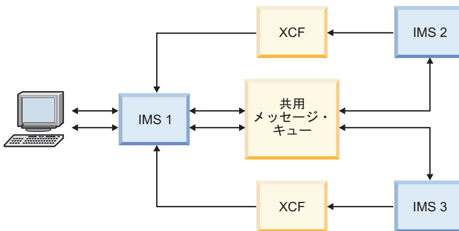
図 137. 共用キュー・グループの複数の IMS システムで処理される OTMA メッセージ
