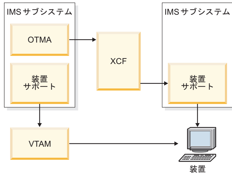
図 126. IMS は、OTMA クライアント内でインプリメントされている装置サポートを使用している装置を使用して通信を行います。
