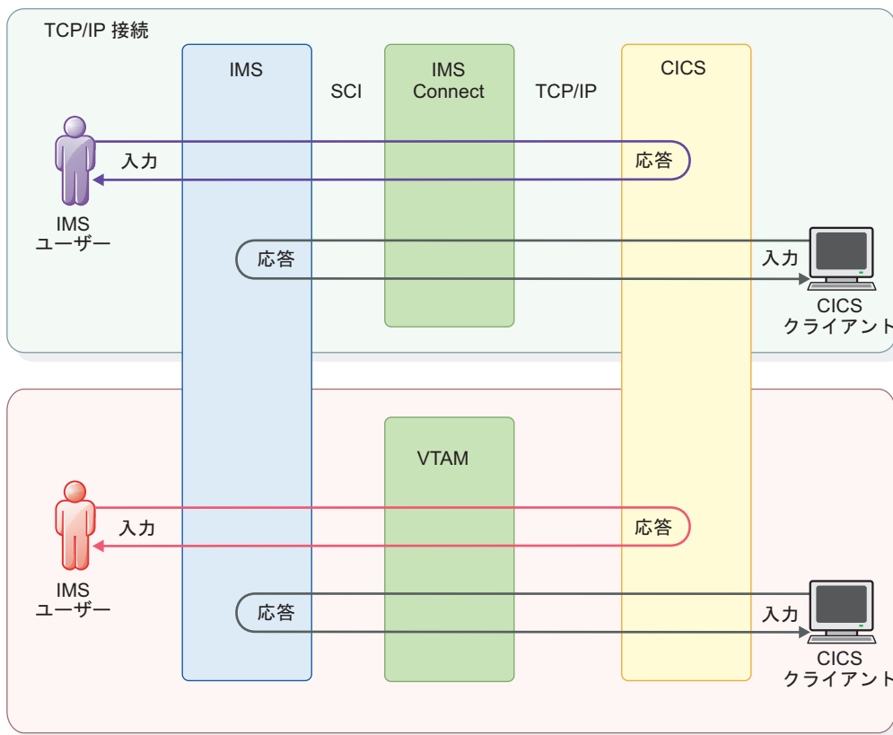
図 81. ISC TCP/IP と ISC VTAM 通信フローの比較
