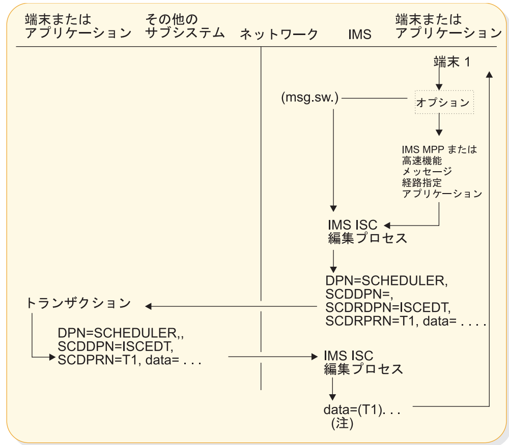
図 71. ISC 編集でのメッセージ経路指定の例
