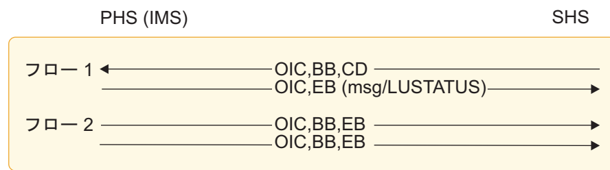
図 87. SINGLE1 として IMS に対して定義された PHS コンポーネントのブラケット・プロトコルの例
