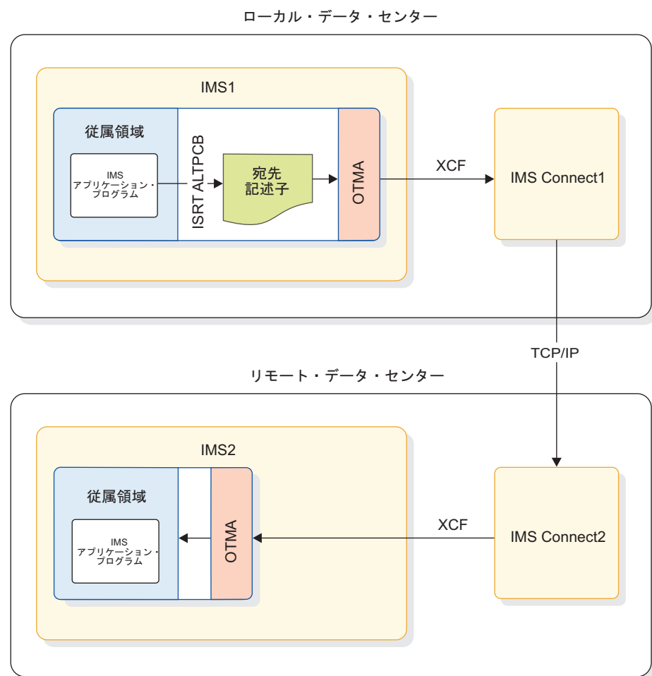
図 128. OTMA トランザクション・メッセージの IMS 間 TCP/IP 通信フロー
