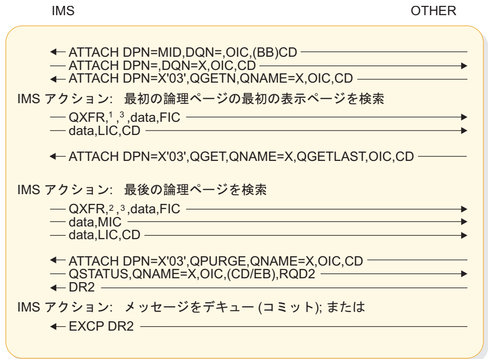
図 92. OLP が定義され、QGET (最後のページ要求であり、カーソルによる) が使用されている要求時ページ化出力の例。メッセージをデキューするために使用される QPURGE
