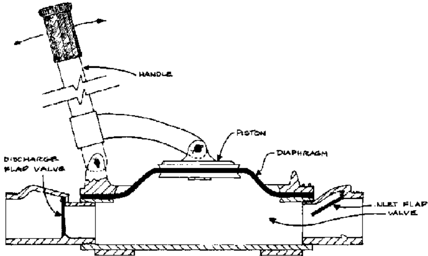
FIG. VII-9. DIAPHRAGM PUMP
