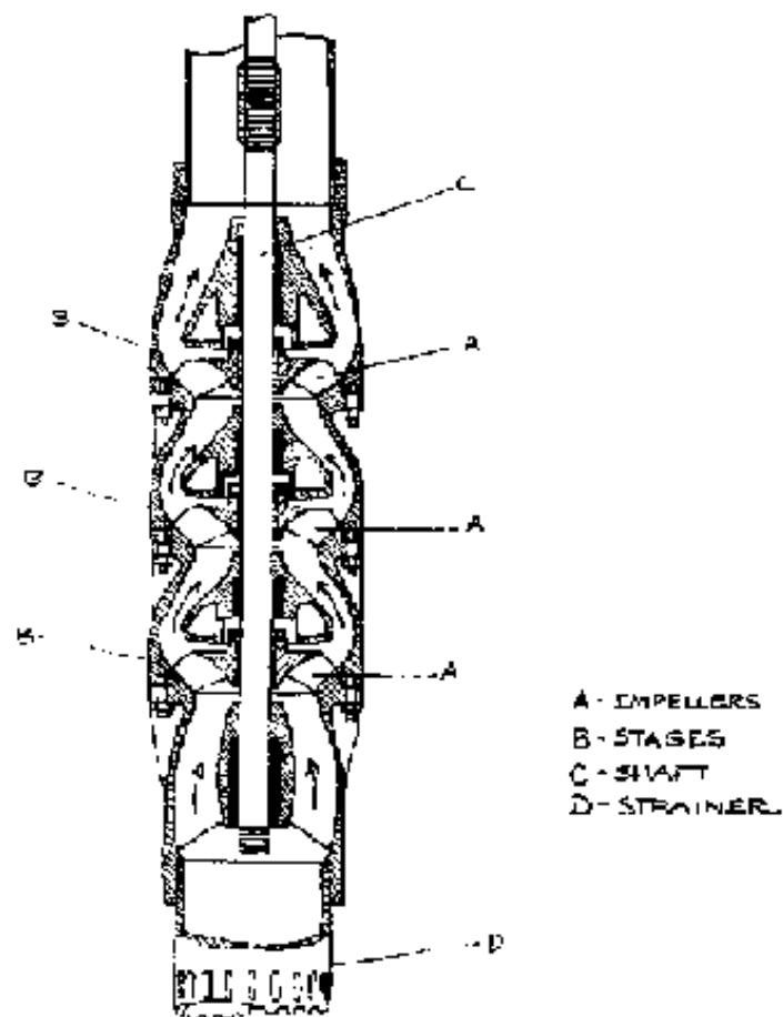
FIG. VII-14. TURBINE PUMP
