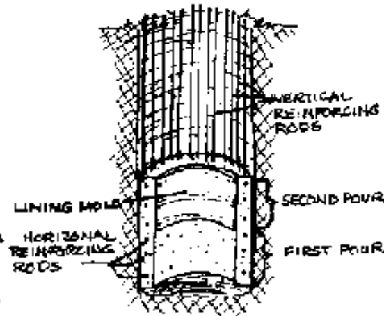
FIG. 1-2. DIG-A-METER, POUR-A-METER
