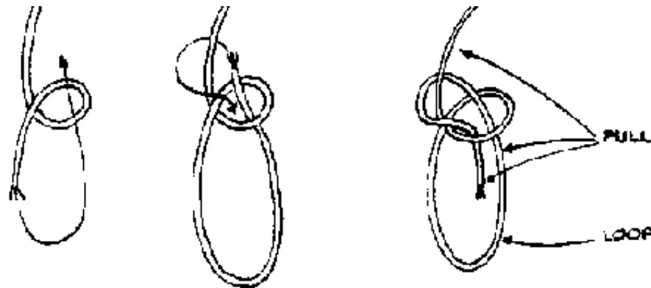
FIG. 5-9. BOWLINE
