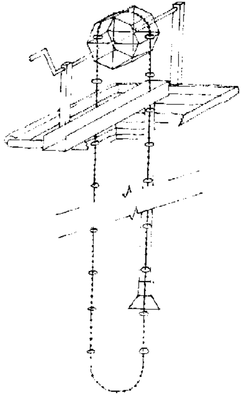
FIG. VII-12. CHAIN PUMP
