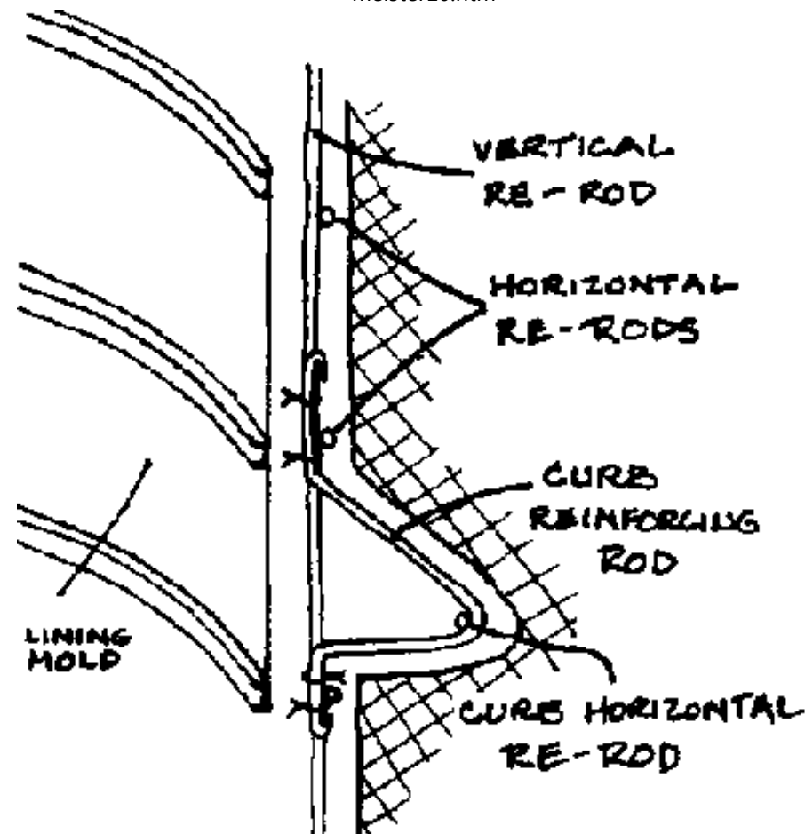
FIG. 7-4. LINING CURB
