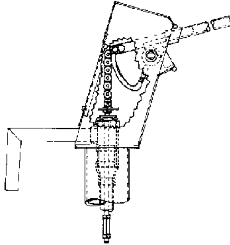
FIG. VII-7. JALNA PUMP HEAD
