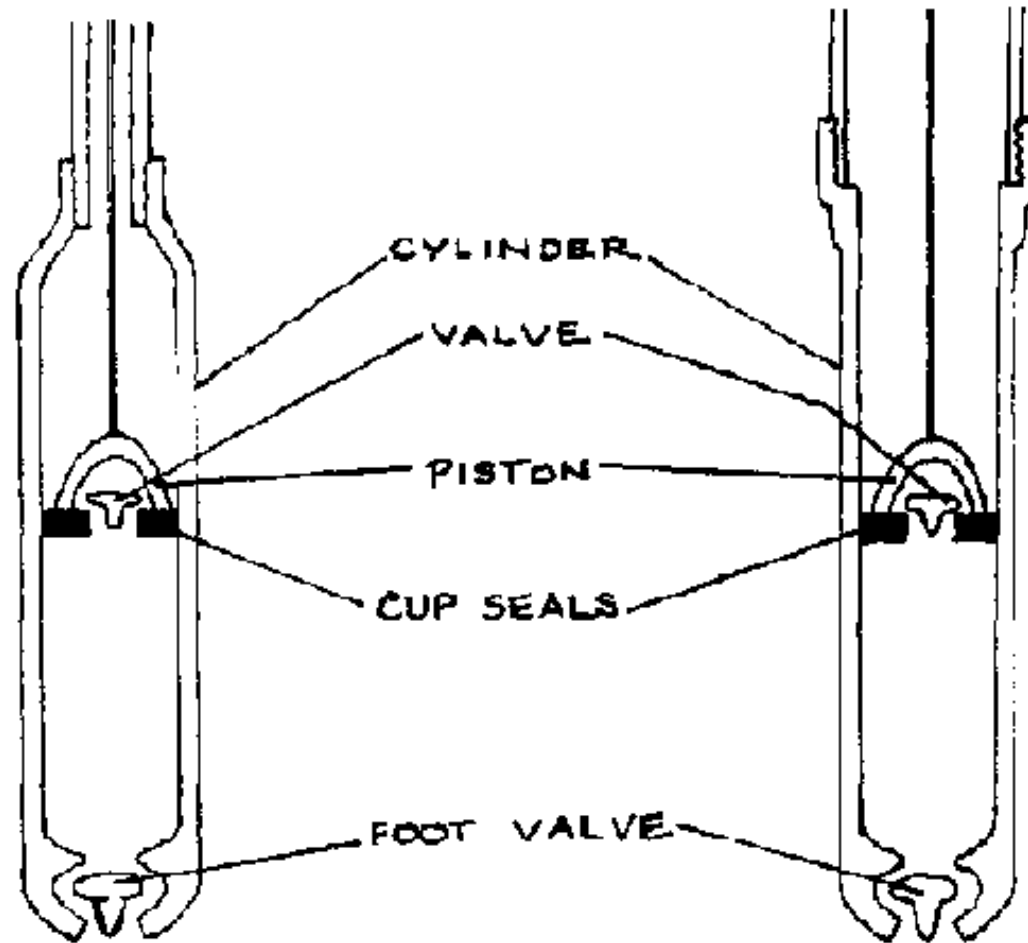
FIG. VII-5. NON-EXTRACTABLE CYLINDER & FIG. VII-6. EXTRACTABLE CYLINDER
