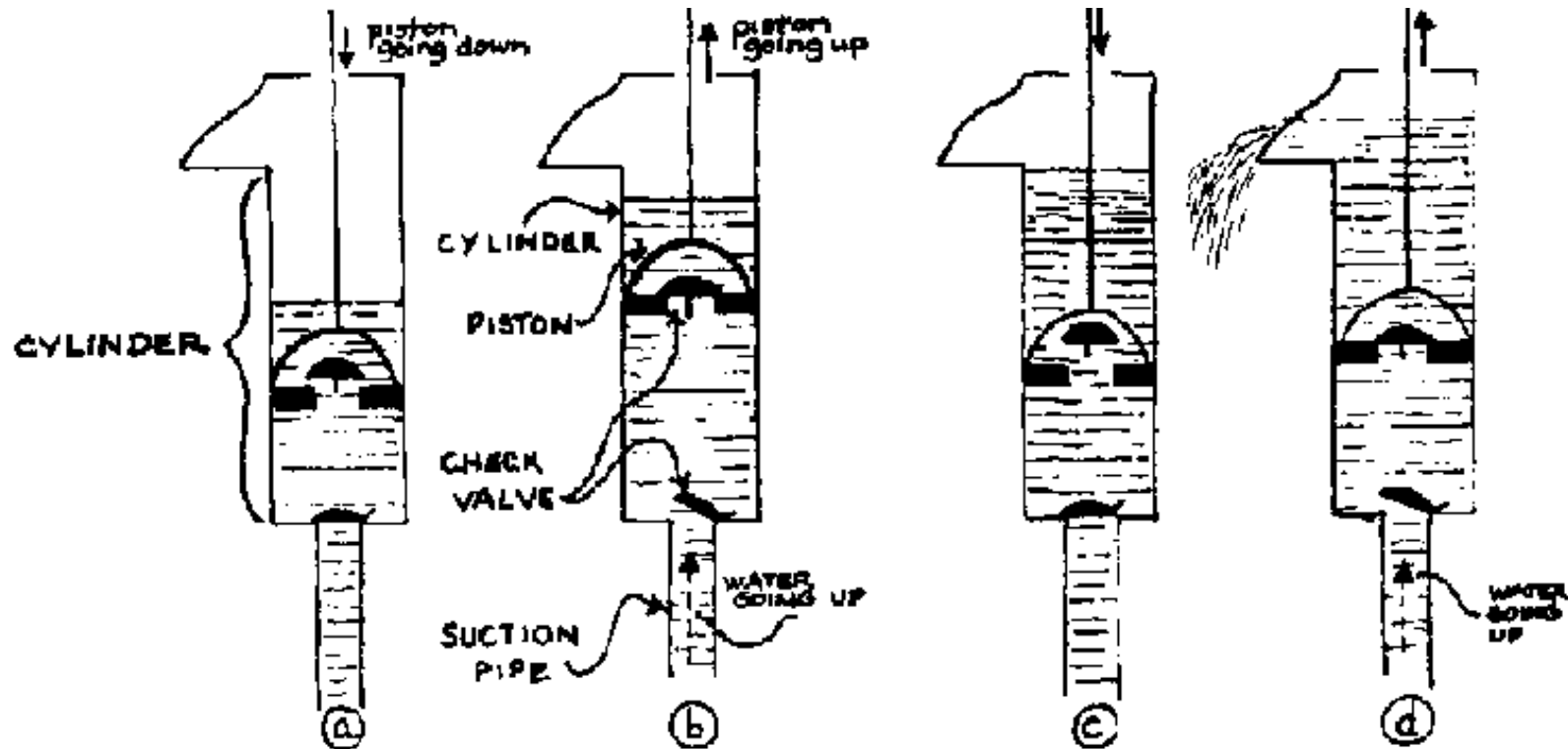
FIG. VII-1. PUMP ACTION
