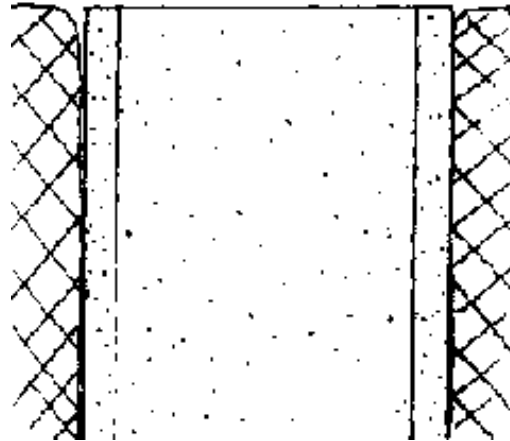
FIG. 8-2. NO HEADWALL
