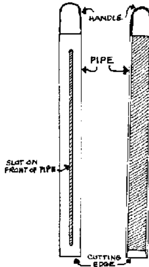
FIG. 12-9. HOLLOW ROD BIT
