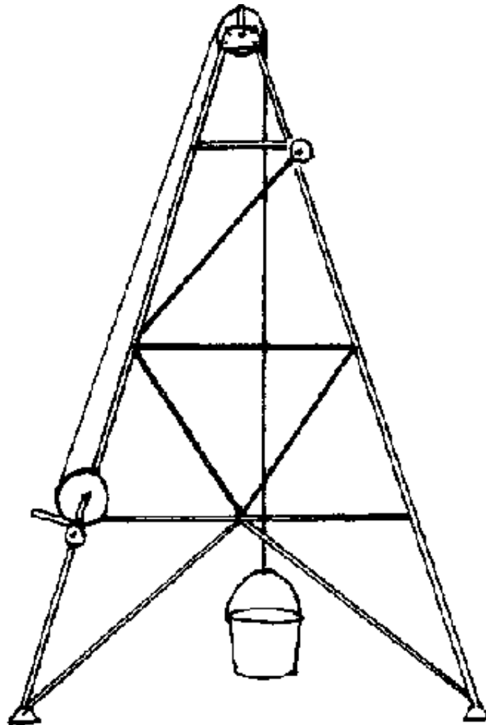
FIG. 5-6. HEADFRAME
