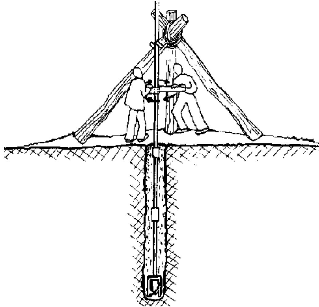
FIG. 12-1. HAND AUGERING
