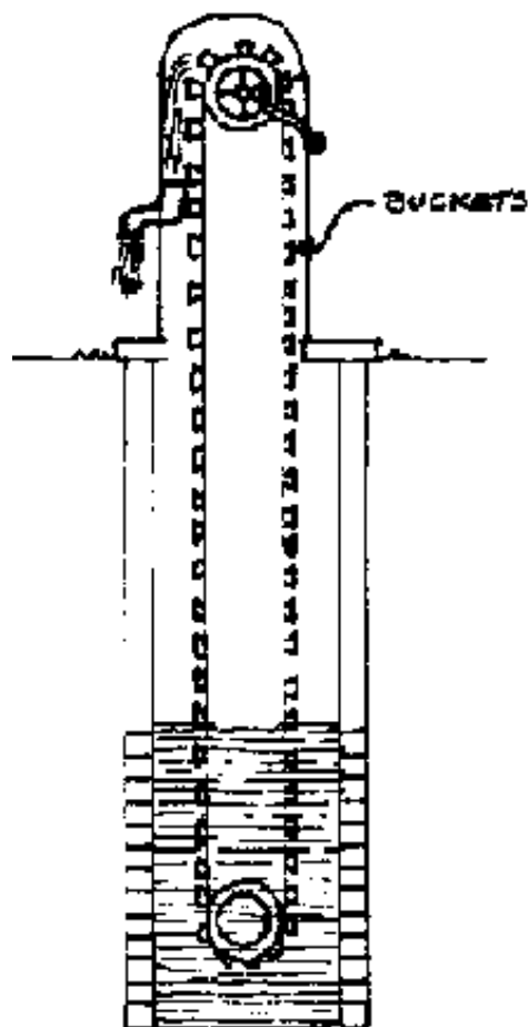
FIG. VII-11. BUCKET PUMP
