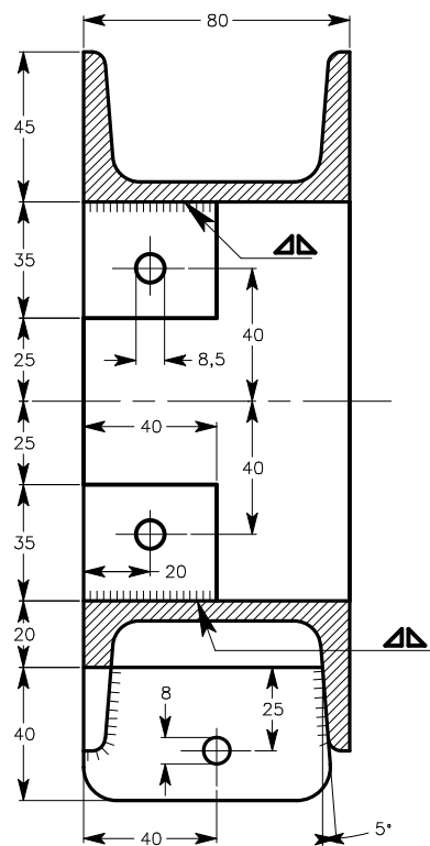
B-B
