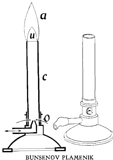
BUNSENOV PLAMENIK
