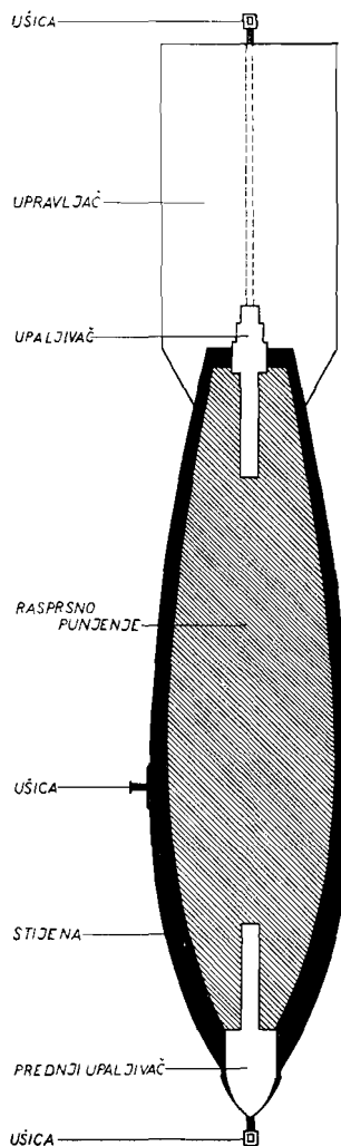
PRESJEK KROZ BOMBU
