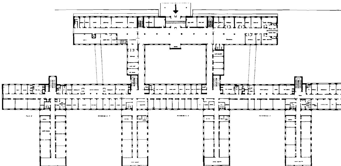
ZAKLADNA BOLNICA U ZAGREBU Tlocrt prizemlja
