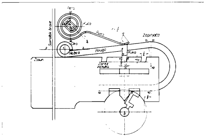
KONSTRUKCIJA ZAPINJAČE I PERA OBICNE ZASUNASTE BRAVE NA DVA OKRETAJA
