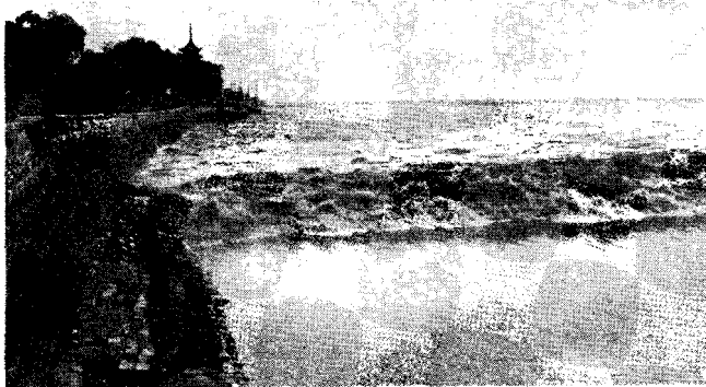
BORE NA TSIEN-TANG-KIANGU (Thorade, Probleme der Wasserwellen , Hamburg 1931)
