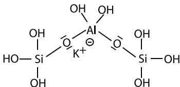
#2 ortho(sialate-siloxo)
