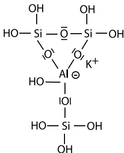
#4 ortho(sialate-disiloxo)
