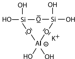
#3 ortho(sialate-siloxo)
