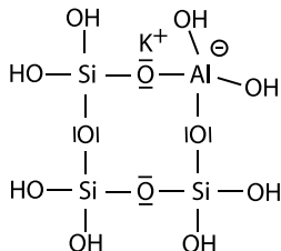
#5 ortho(sialate-disiloxo)
