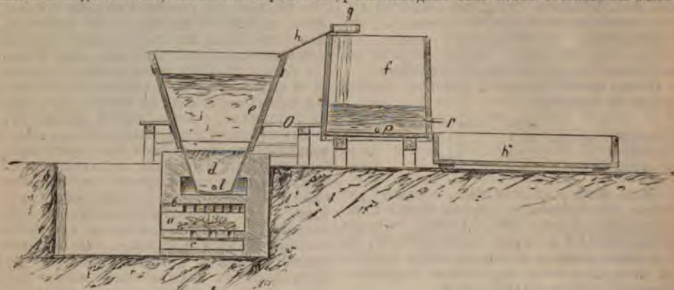
Фиг. 1. Схема салотопленія на небольшихъ русскихъ салотопенныхъ заводахъ. a —топка подъ котломъ; e —зольникъ; d —металлическая часть салотопеннаго котла; e —наставка; f —отстойный чанъ; g —сито; h —желобъ, по которому шквара съ сала спускается въ котель; k —холодильный ларь; l —отверстіе для выпуска воды и шквары. p —отверстіе для выпуска сала; o —помость.
