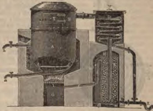
Фиг. 4. Аппаратъ Воля.
