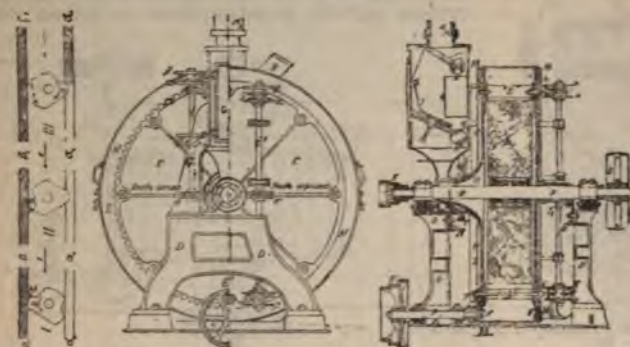
Фиг. 8, 9 и 10. Брусная постава типа Мартена, с горизонтальной осью.
