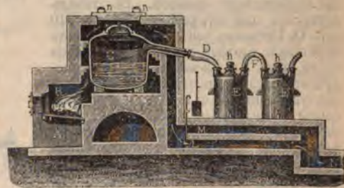
Фиг. 4. Стоячая реторта.
