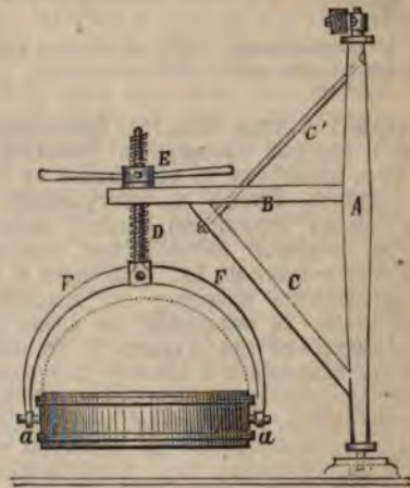
Кранъ для жернововъ.
