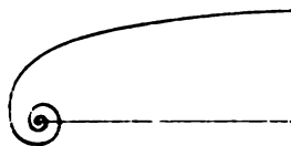
8) Гиперболическая спираль.
