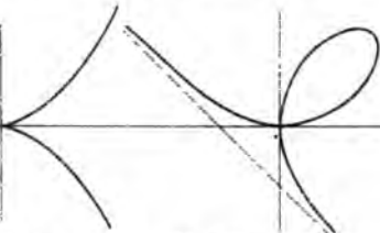
4) Циссоида.
