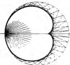
7) Кардиоида или эластическая кривая.
