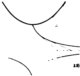
13) Звездчатые кривые.
