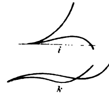
12) Трактория.
