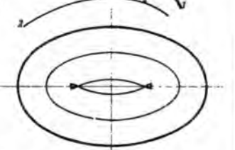
9) Эллипс с параллельными кривыми.
