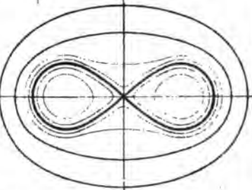
14) Линия Лиссажу.
