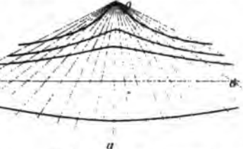
10) Конхоиды: а) Никомеда, б) круговая.
