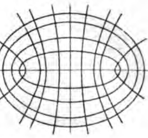
12) Конфокальные кривые 2-го порядка.
