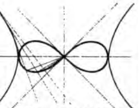
3) Равносторонняя гипербола с подошвенною кривою.
