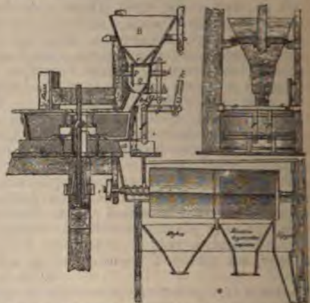
Фиг. 1 и 2. Крупяной поставъ съ кольцевидною воронкою, вращающійся на вертикальной оси. Разрѣзъ въ видѣ сбоку.
