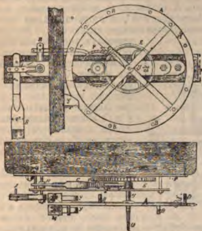
Фиг. 3 и 4. Механизмъ для приведенія въ дѣйствіе задвижки K , поставъ (см. фиг. 1 и 2).
