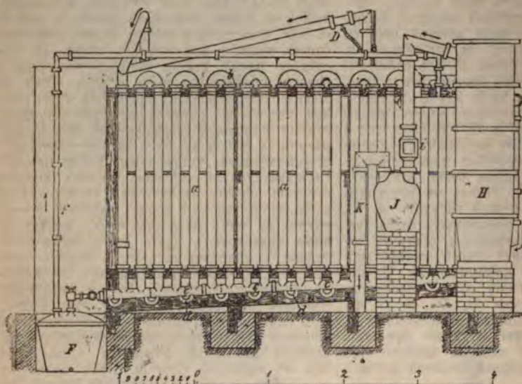
Фиг. 8. Конденсационный аппаратъ Гутманна и Рорманна.
