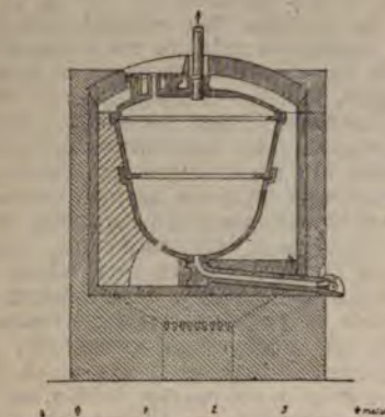
Фиг. 5. Реторта О. Гутманна.
