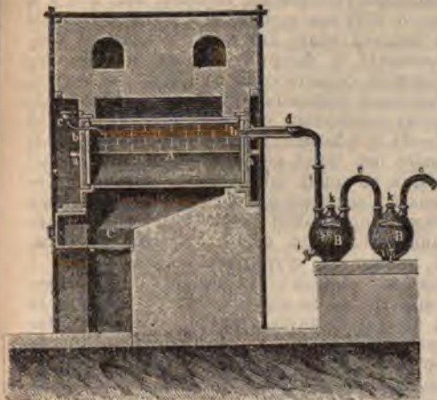
Фиг. 3. Лежачая цилиндрическая реторта.
