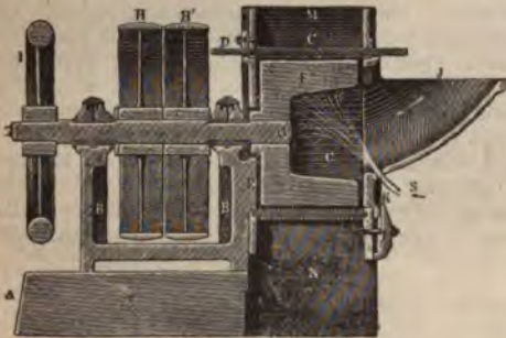
Фиг. 2. Терка Шампонуа.
