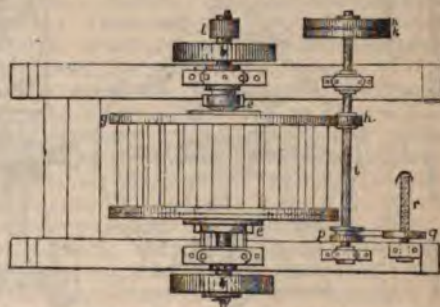
Фиг. 7. Крушьяной поставъ съ горизонтальной осью. Видъ сверху.
