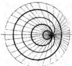
8) Улитка Паскаля.
