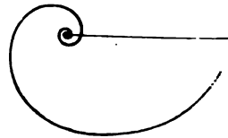
10) Логарифмическая спираль.
