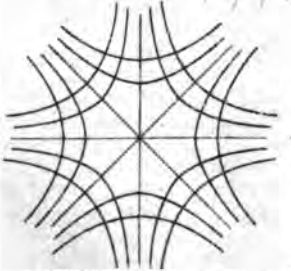
13) Ортогональные траектории (для семейства гипербол)
