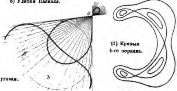
8) Улитка Паскаля.
