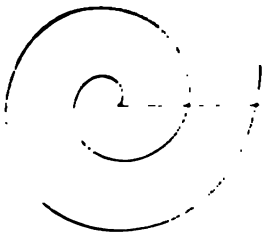
7) Архимедова спираль.
