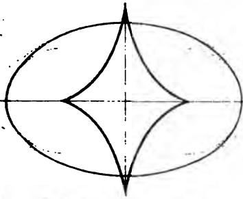
1) Эллипс и его развертка.
