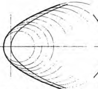
2) Парабола как огибающая ряда окружностей.
