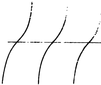
2) Тангенсоиды.
