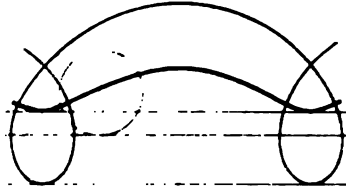
5) Растянутая и сжатая циклоиды.
