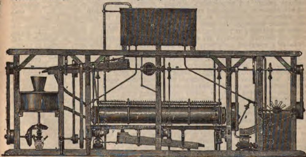
Фиг. 3. Комбинація аппаратовъ для получения К. молока системы В. Ангело.
