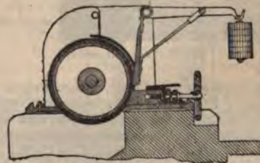
Фиг. 1. Терка В. Ангела.
