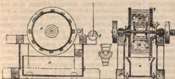
Фиг. 5 и 6. Крушьяной поставъ съ горизонтальной осью. Поперечный и продольный разрѣзы.
