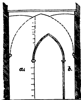
Fig. 4. a. älterer Pfeiler, b. neuer mit Gliederung.
