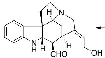
Wieland-Gumlich aldehyde (open form)
