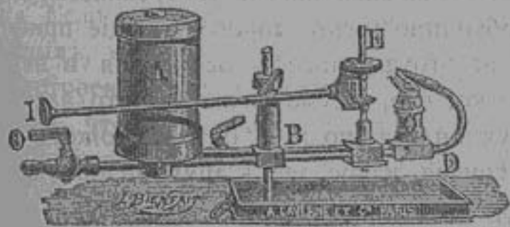
Рис. 36. Горѣлка спирто-кислородная.
