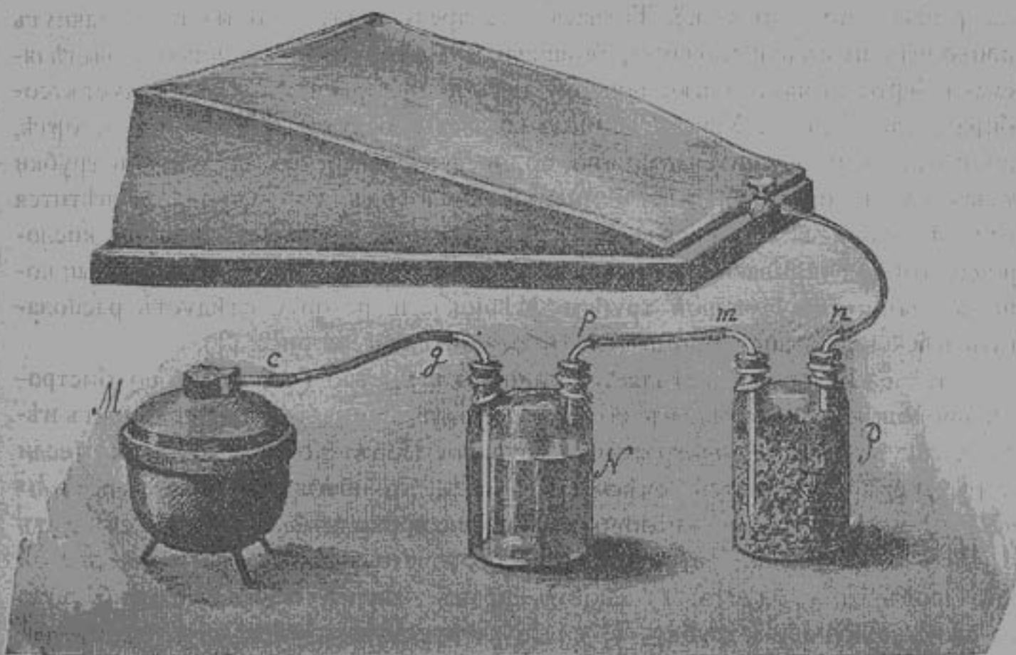
Рис. 45. М—реторта, N—промыватель, P—осушитель, сверху каучуковій мѣшокъ, наполняемый хлористымъ кальціемъ.
