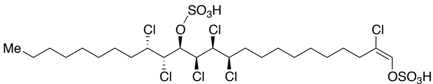
malhamensilipin A
