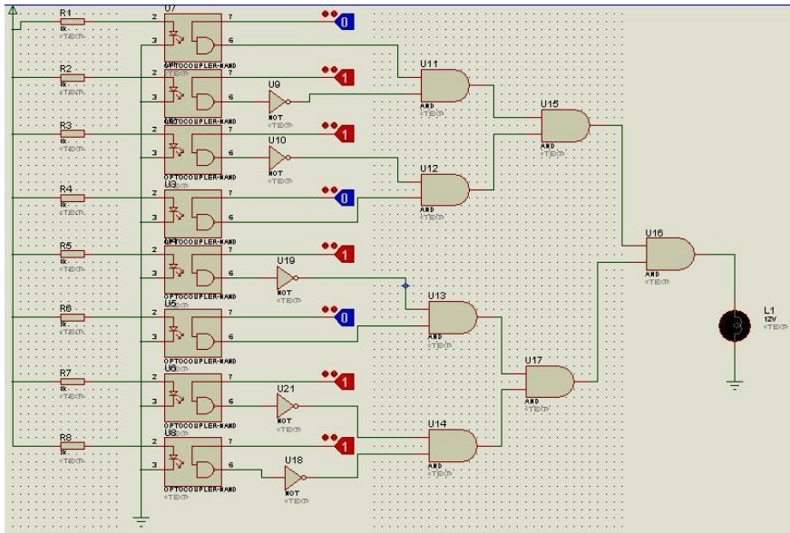
Cerradura electrónica simulado en isis
