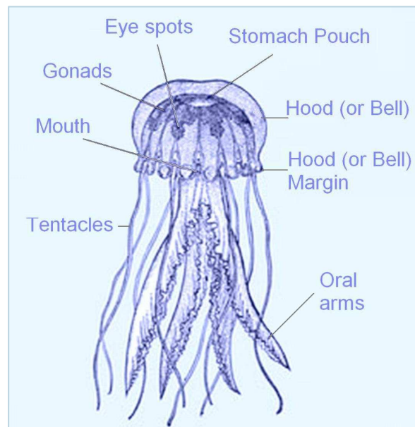
Fig. 13: Coelenterate
