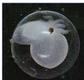
Fig. 18: Cephalopod-embryo.
