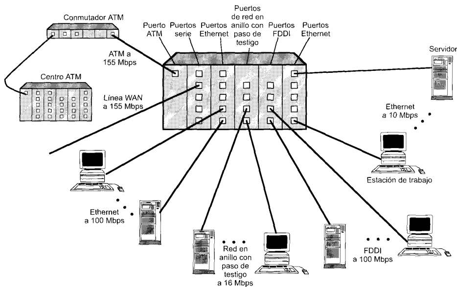
Figura 14.12. Configuración de centro LAN ATM.
