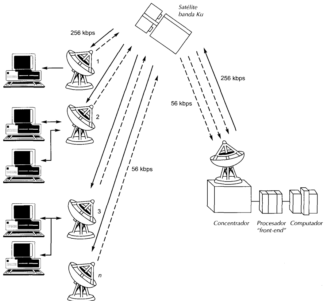
Figura 4.6. Configuración VSAT.
