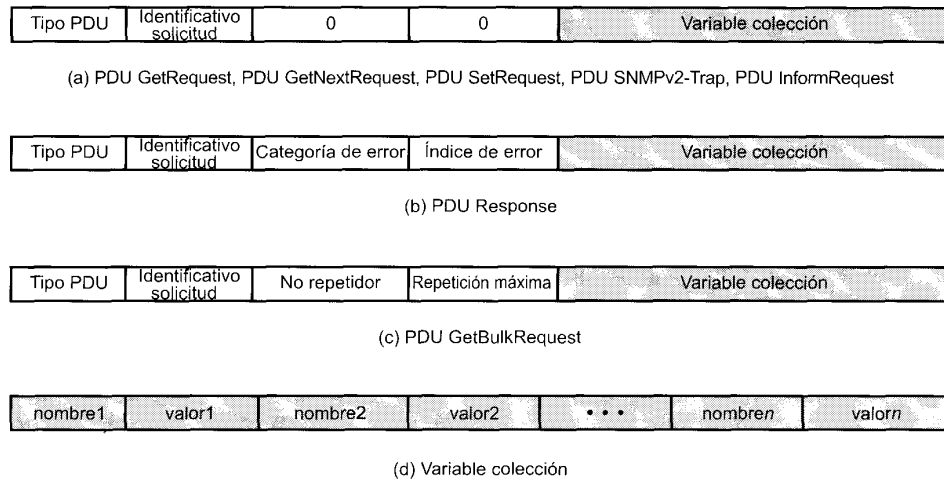
Figura 19.6. Formato de PDU de SNMPv2.
