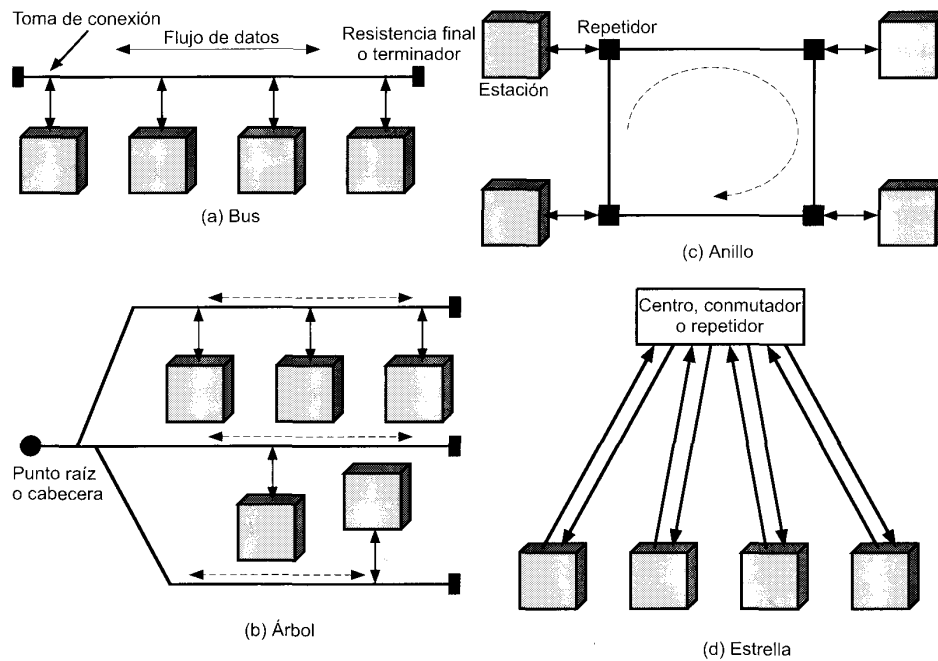
Figura 13.3. Topologías LAN.
