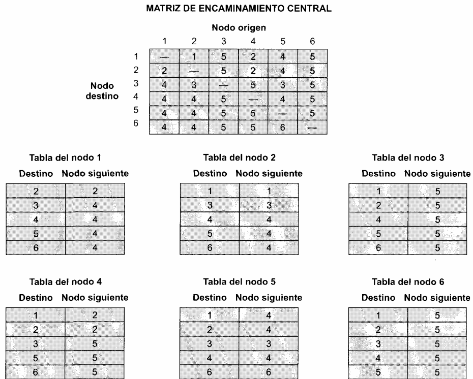
Figura 10.7. Encaminamiento estático (haciendo uso de la Figura 10.6).
