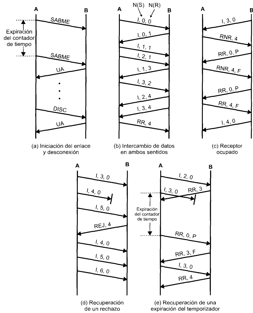
Figura 7.12. Ejemplo de funcionamiento de HDLC.
