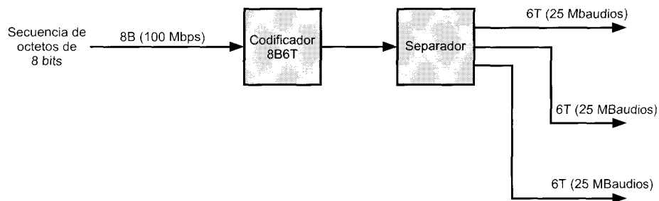
Figura 14.19. Esquema de transmisión 8B6T.
