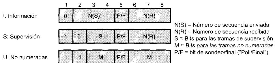
(c) Formato del campo de control de 8 bits
