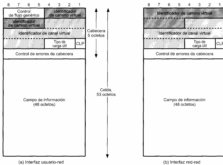
Figura 11.4. Formato de celda ATM.
