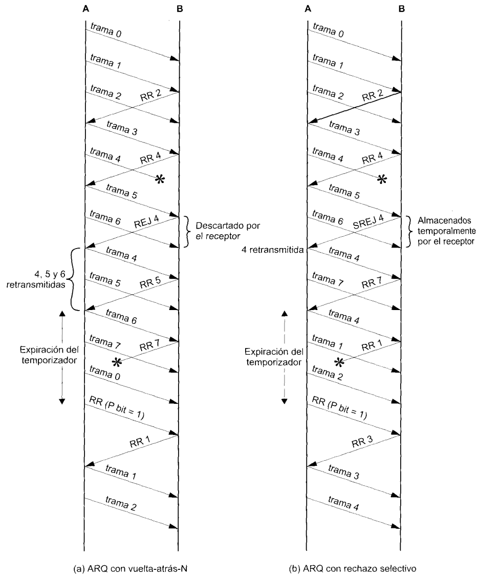
Figura 7.9. Protocolos ARQ con ventana deslizante.
