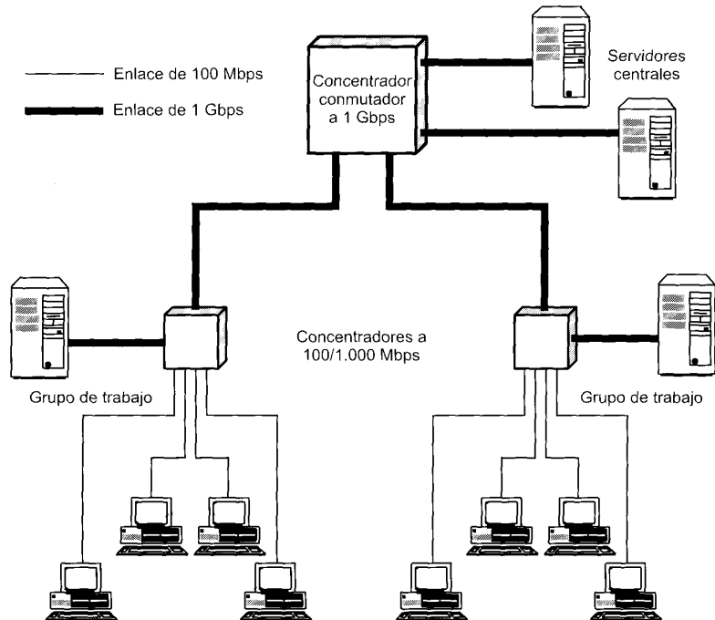
Figura 14.4. Ejemplo de configuración para Gigabit Ethernet.
