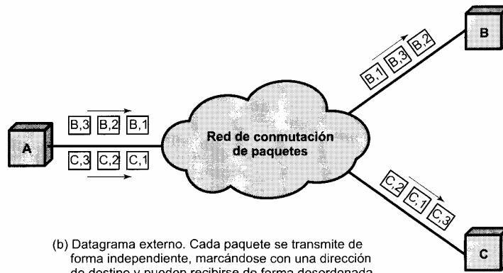
Figura 10.4. Operación de circuito virtual y de datagrama externos.
