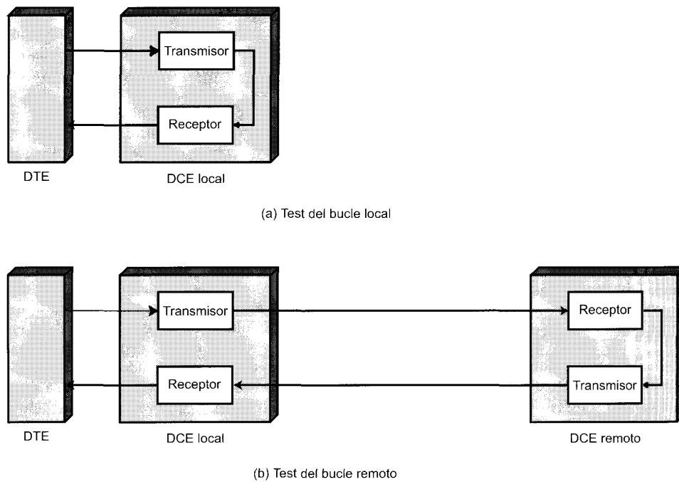
Figura 6.6. Bucles local y remoto.
