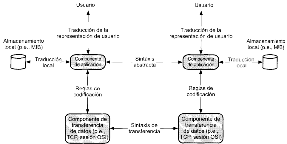
Figura 19.2. El uso de las sintaxis abstracta y de transferencia.
