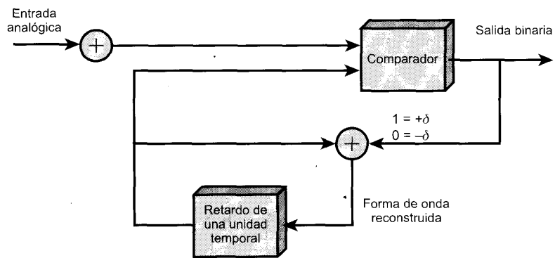
(a) Transmisión
