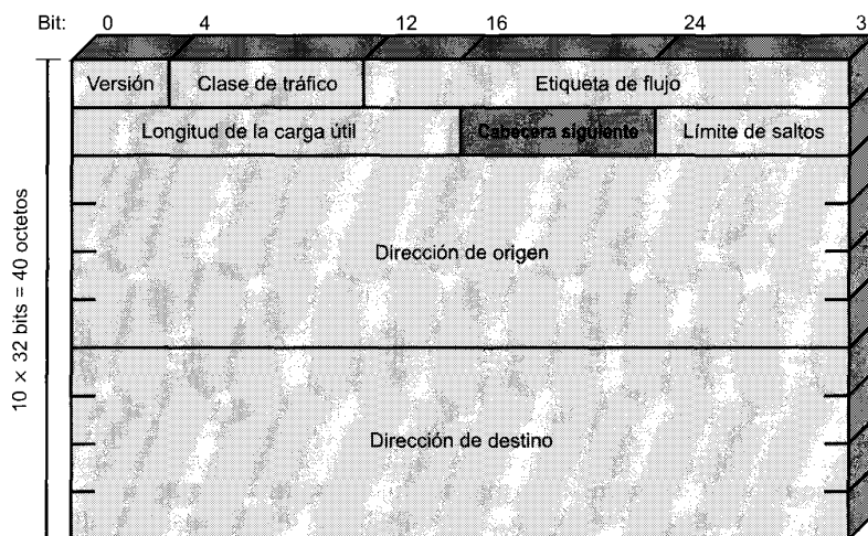
Figura 15.11. Cabecera IPv6.
