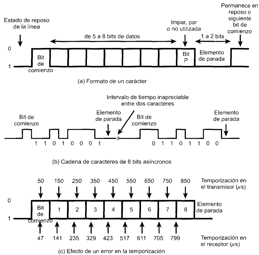
Figura 6.1. Transmisión asincrónica.
