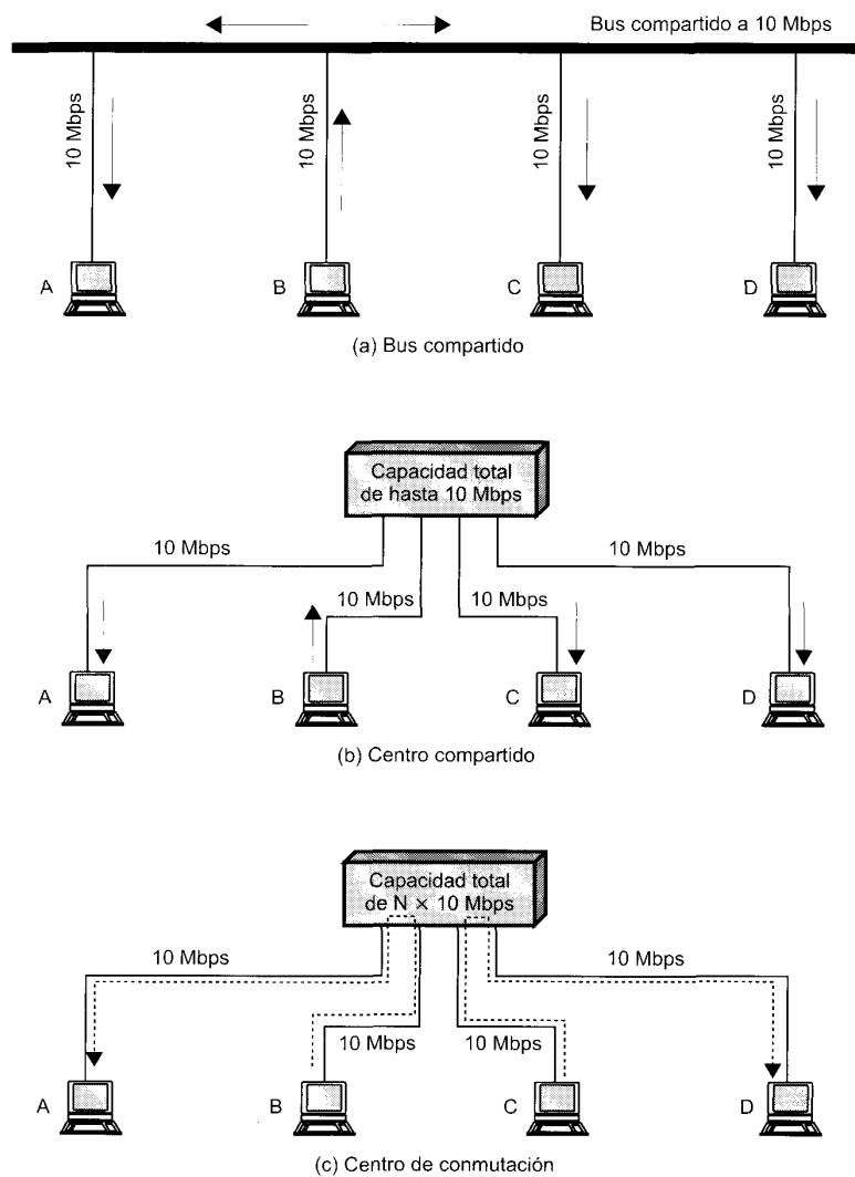
Figura 13.10. Centros y conmutadores en una LAN.
