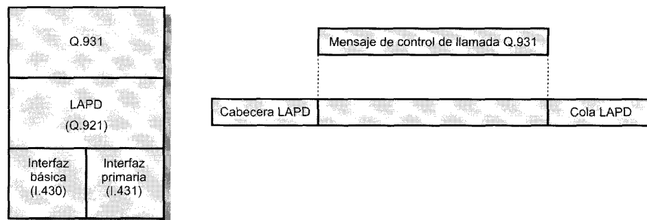
Figura A.9. Arquitectura del protocolo de control de llamadas.
