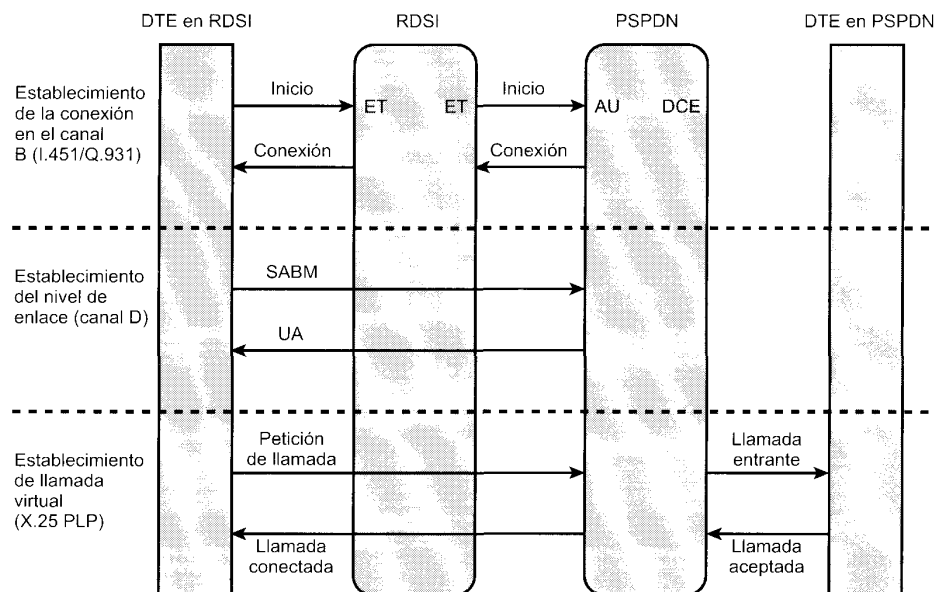
Figura A.6. Inicio de llamada virtual.
