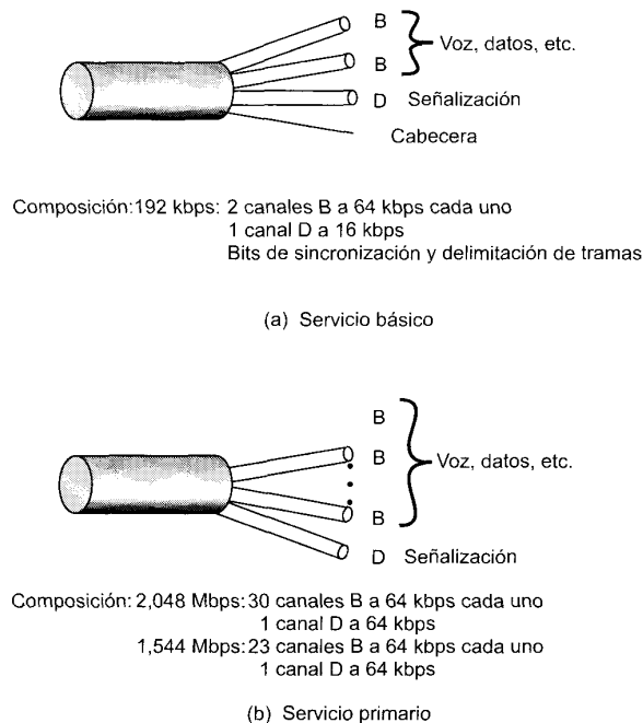
Figura A.3. Estructura de canal RDSI.
