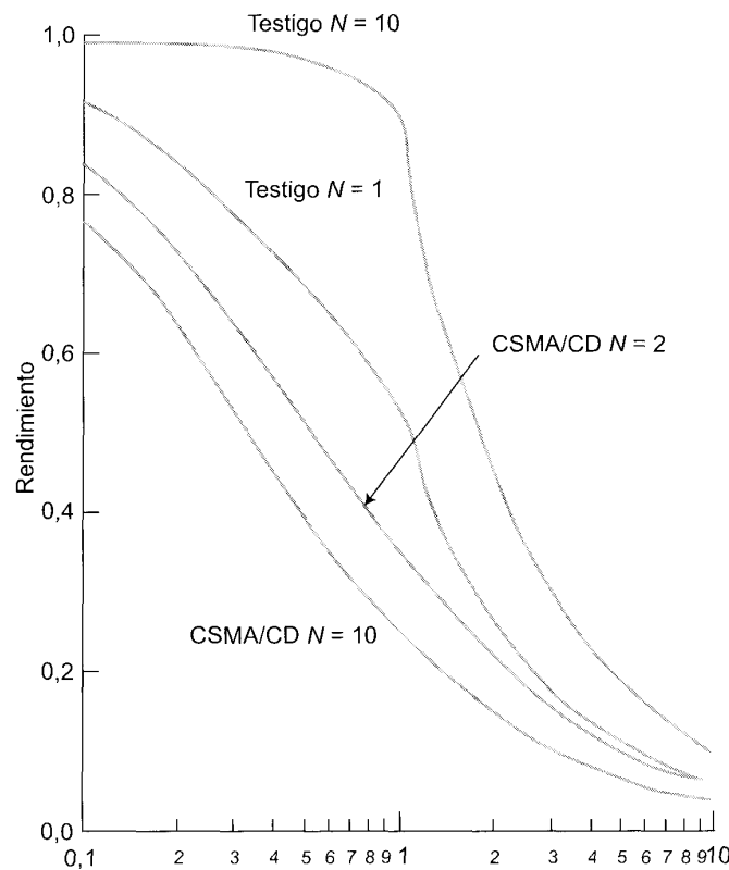
Figura 14.22. Rendimiento en función de a para las técnicas de paso de testigo y CSMA/CD.
