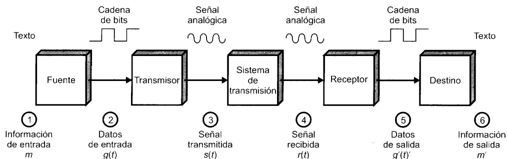
Figura 1.2. Modelo simplificado para las comunicaciones de datos.
