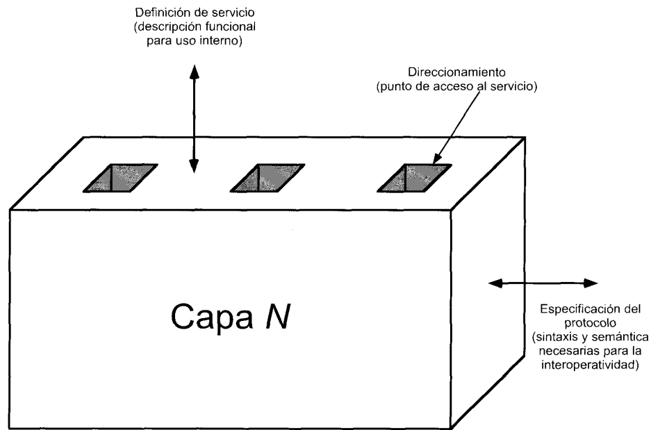
Figura 2.8. Normas específicas de capa.
