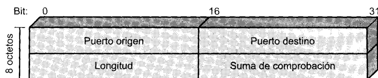
Figura 17.15. Cabecera UDP.
