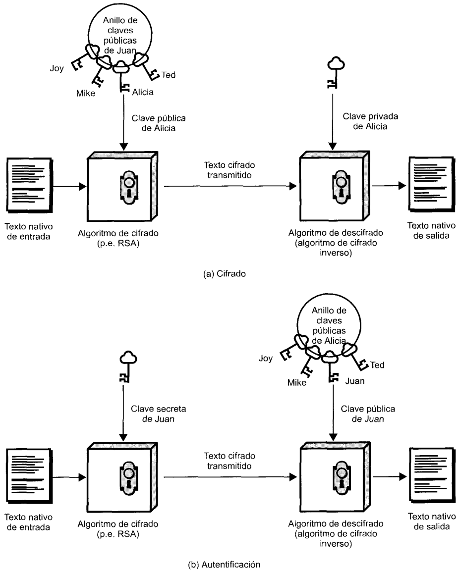
Figura 18.11. Cifrado de clave pública.
