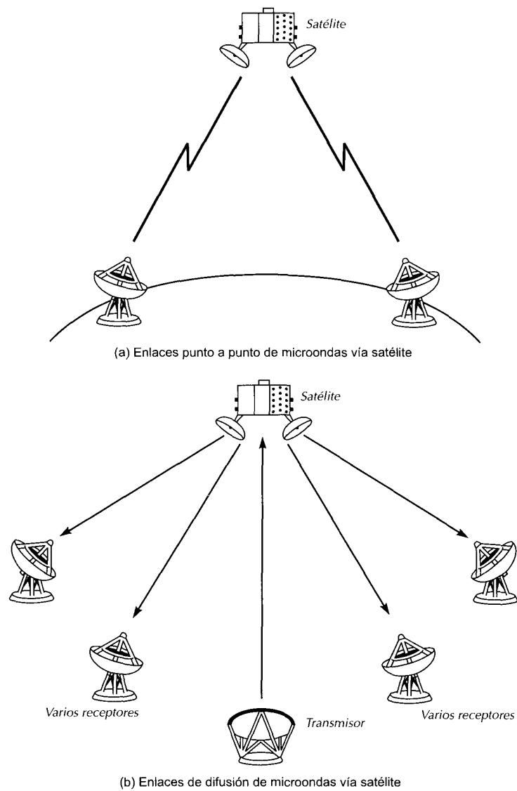
Figura 4.5. Distintas configuraciones de comunicaciones vía satélite.
