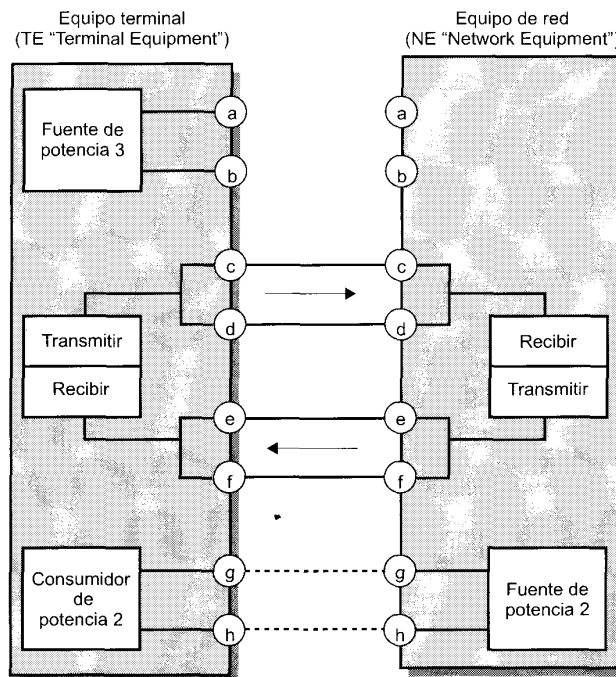
Figura 6.9. Interfaz RDSI.
