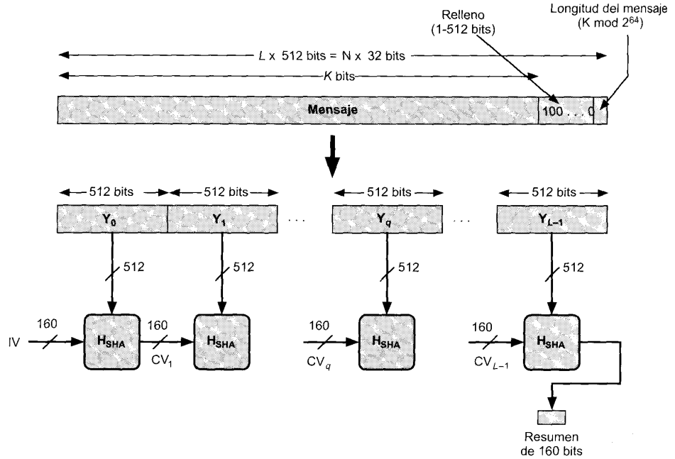
Figura 18.9. Generación de resumen de mensaje utilizando SHA-1.
