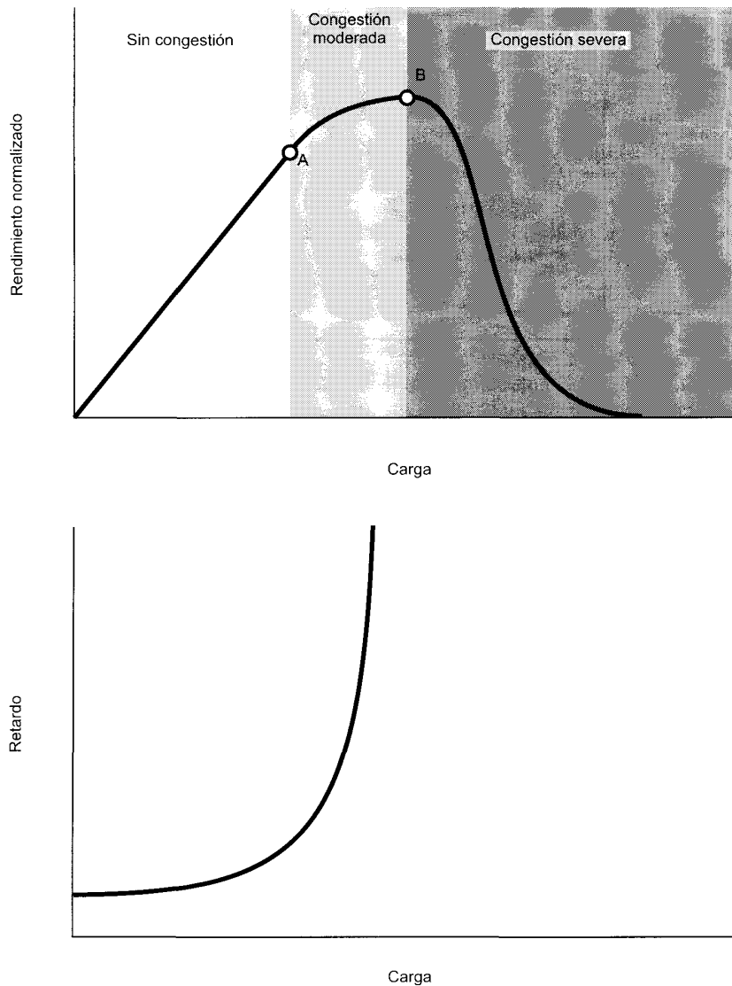
Figura 12.4. Efectos de la congestión.
