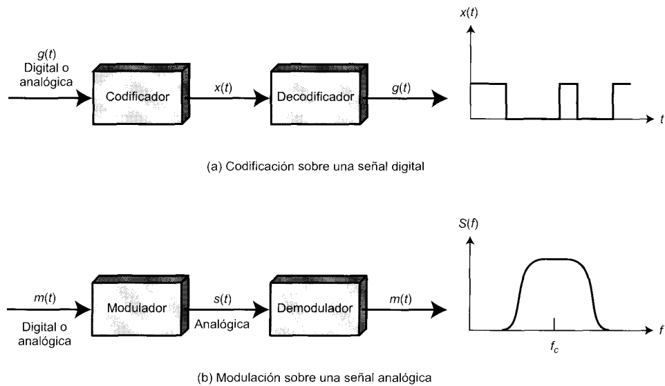
Figura 5.1. Técnicas de codificación y modulación.
