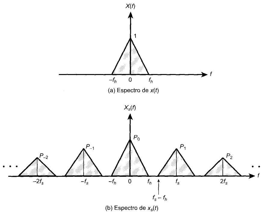
Figura 5.27. Demostración del teorema de muestreo.
