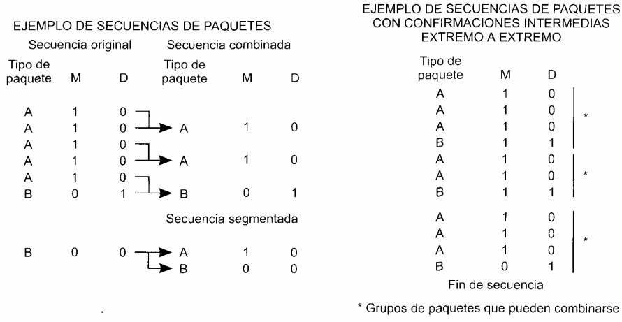
Figura 10.19. Secuencias de paquetes X.25.
