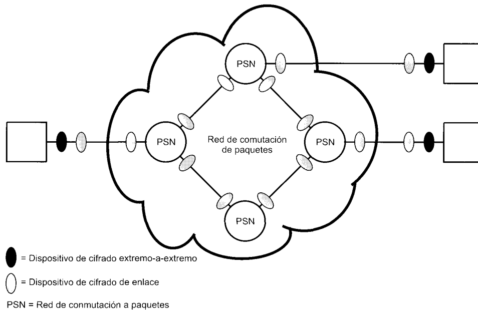
Figura 18.5. Cifrado a través de una red de conmutación a paquetes.
