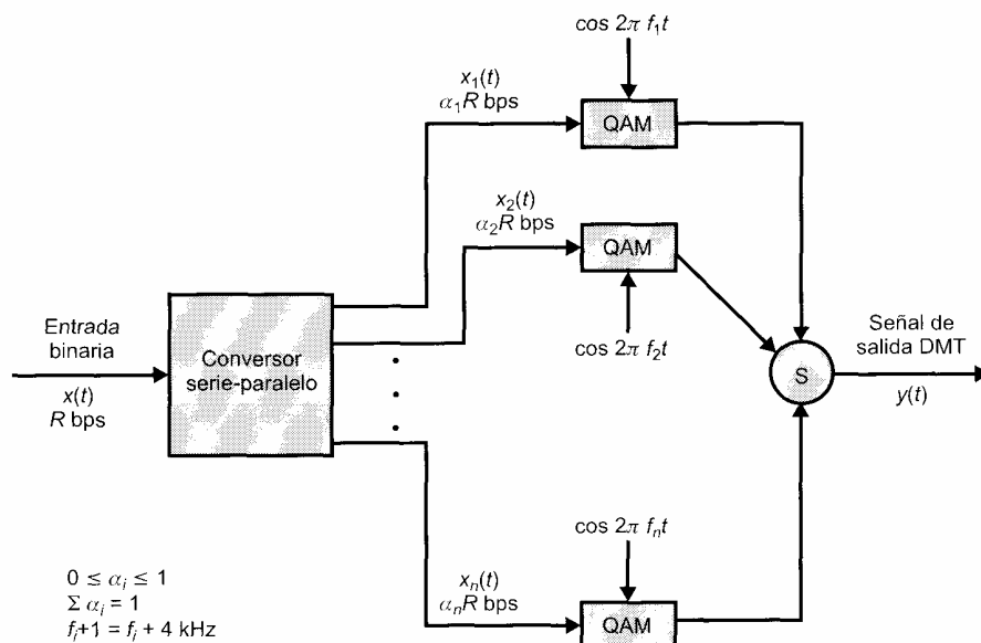
Figura 8.20. Transmisor DMT.
