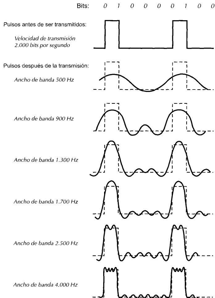
Figura 3.8. Efecto del ancho de banda en las señales digitales.
