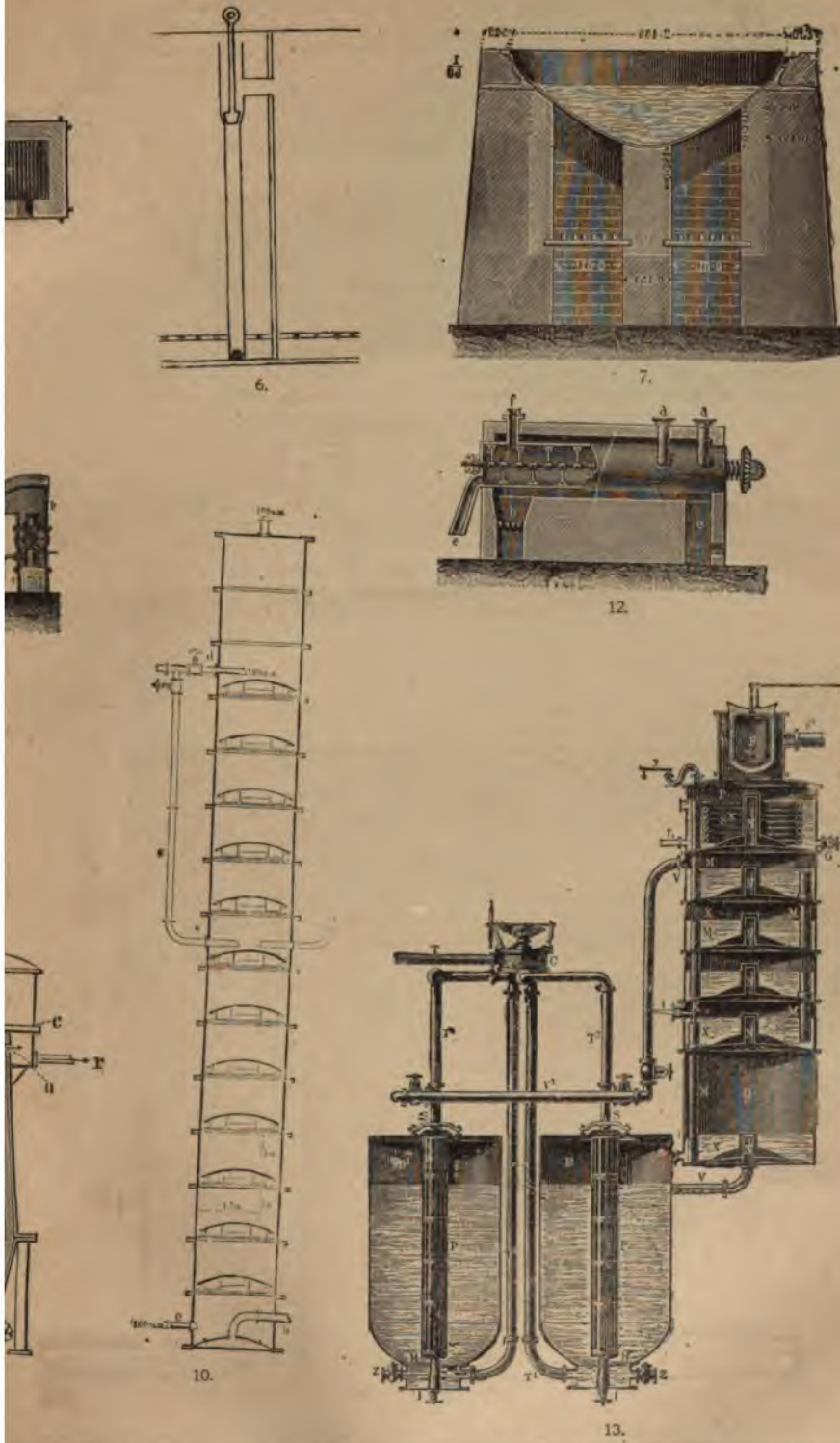
6. (горизонтальный разрьз). 4. Она же (виъшній видъ). 5. Аппаратъ Дёплова-Шанкса для выщелачиванія сырого содоваго щелока нижнимъ огнемъ. 8. Абсорберъ Сольвея для насыщешя раствора-фильтръ для отдълешя кислой У. соли отъ маточнаго раствора. 12. Кальцинировочная печь. 13. Аппаратъ для аммиака Сольвея.
