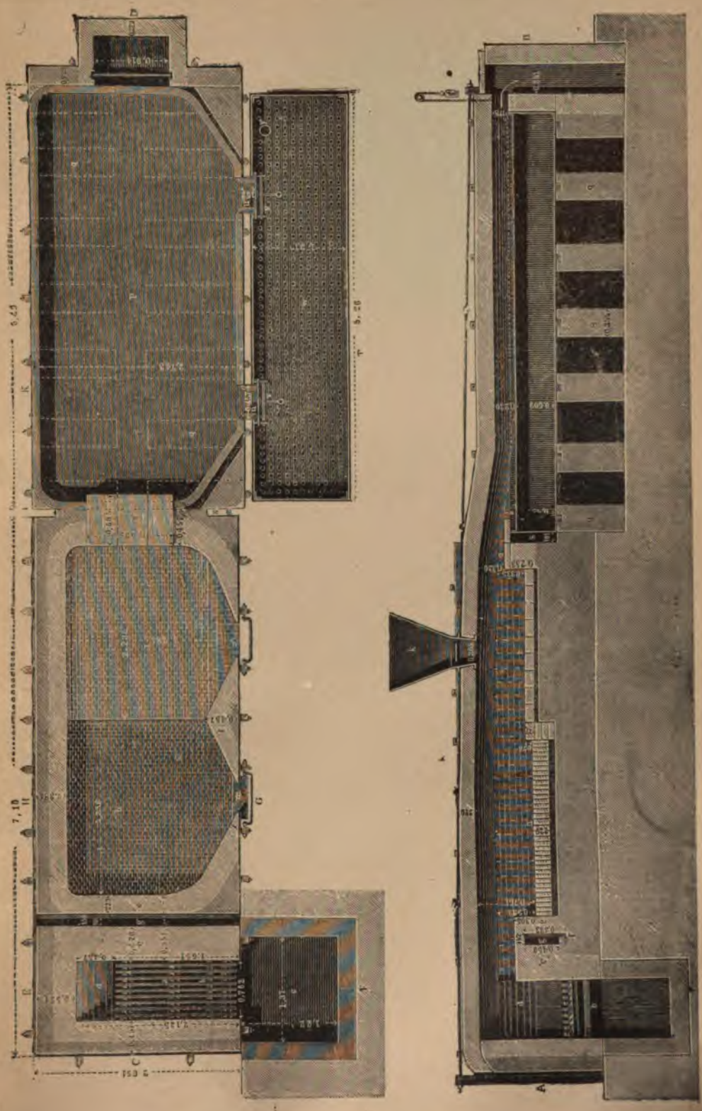
Английская леблановская содовая печь съ выпарнымъ чреномъ и ф льтромъ при ней въ горизонтальномъ и вертикальномъ разрьзахъ.
