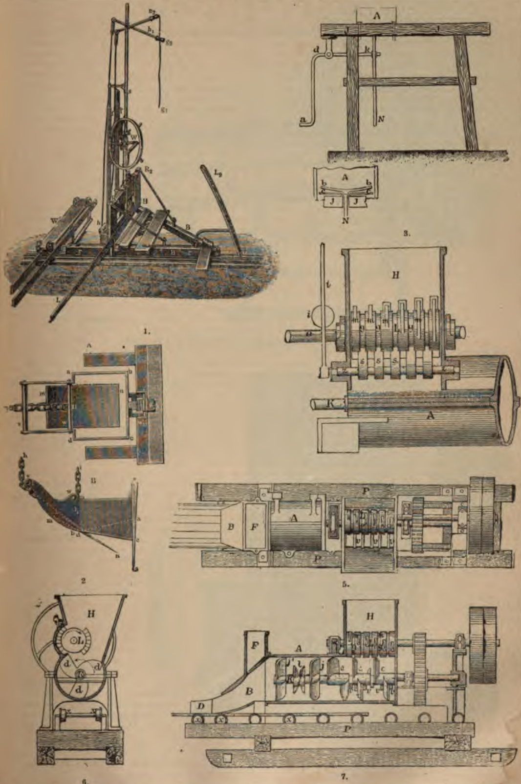
1. Машина Бржозовскаго для вырѣзки торфа. 2. Устройство ея ножей: А—планъ, В—боковой видъ. 3. Станокъ для приготовления столоваго торфа. 4. Устройство дробителя въ машинѣ Шликкейна. 5. 6 и 7. Планъ, поперечный и продольный разрѣзъ машины для прессованія торфа Шликкейна.
