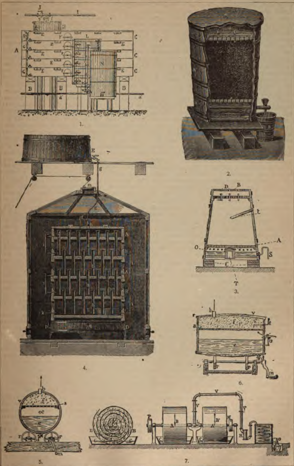
1. Аппарат Клодона. 2. „Essigbilder“. 3. То же—усовершенствованный. 4. Аппарат Зингера. 5 и 6. Аппарат Михаэлиса. 7. Аппарат Виллона.
