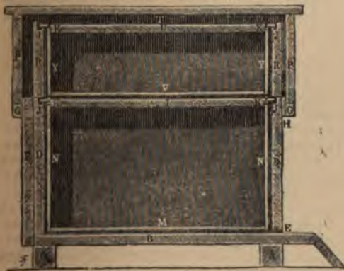
11. Улей Лангстрота съ позднѣйшими усовершенствованіями Дадана.
