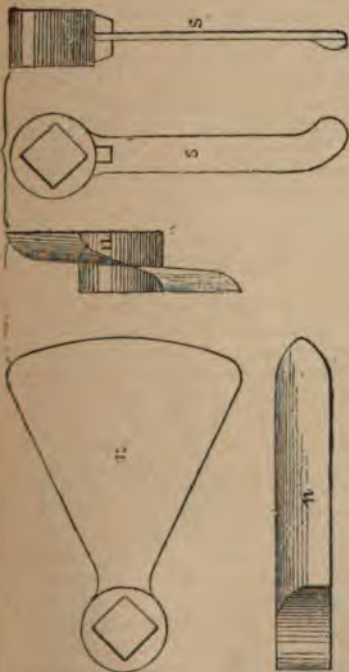
2. Ножи машины для наливного формованного торфа.
