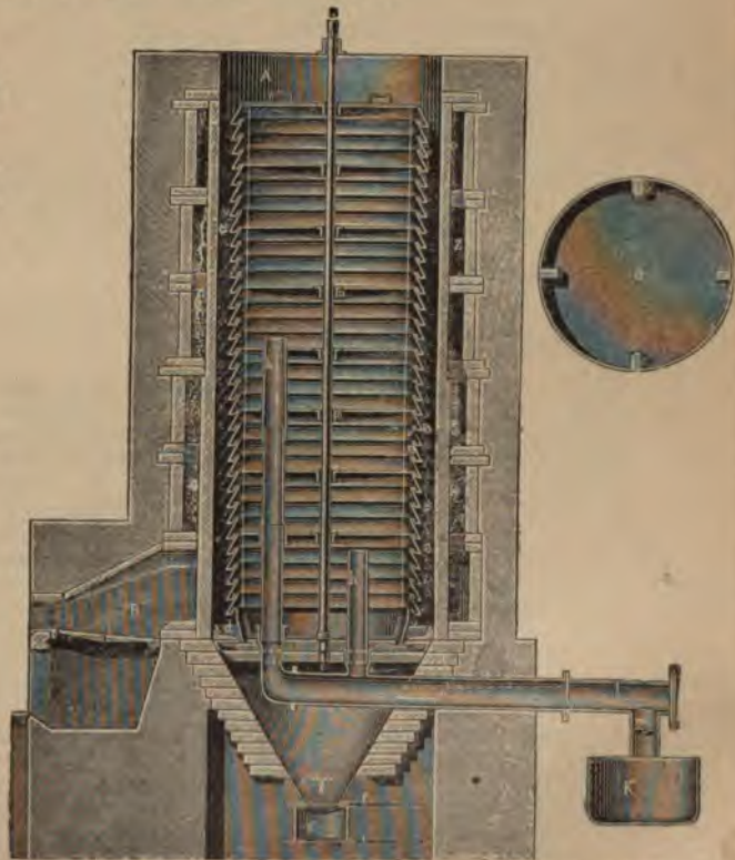
3. Стоячая реторта Родле для коксования бурого угля и торфа.
