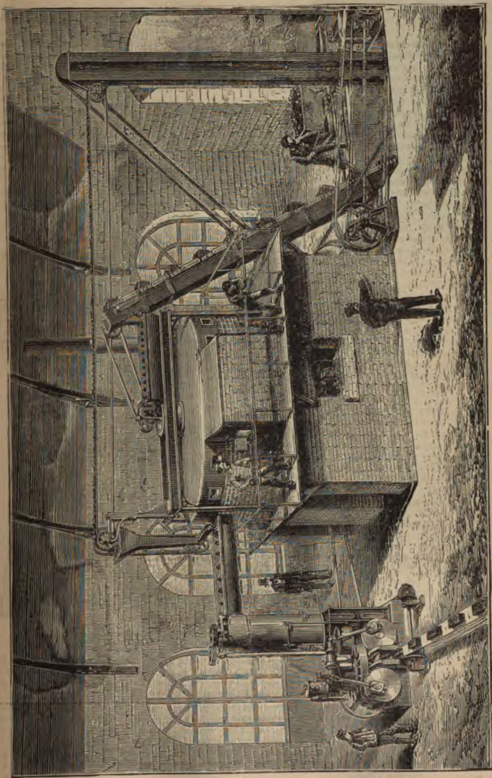
Общий видъ устройства для производства угольныхъ брикетовъ.
