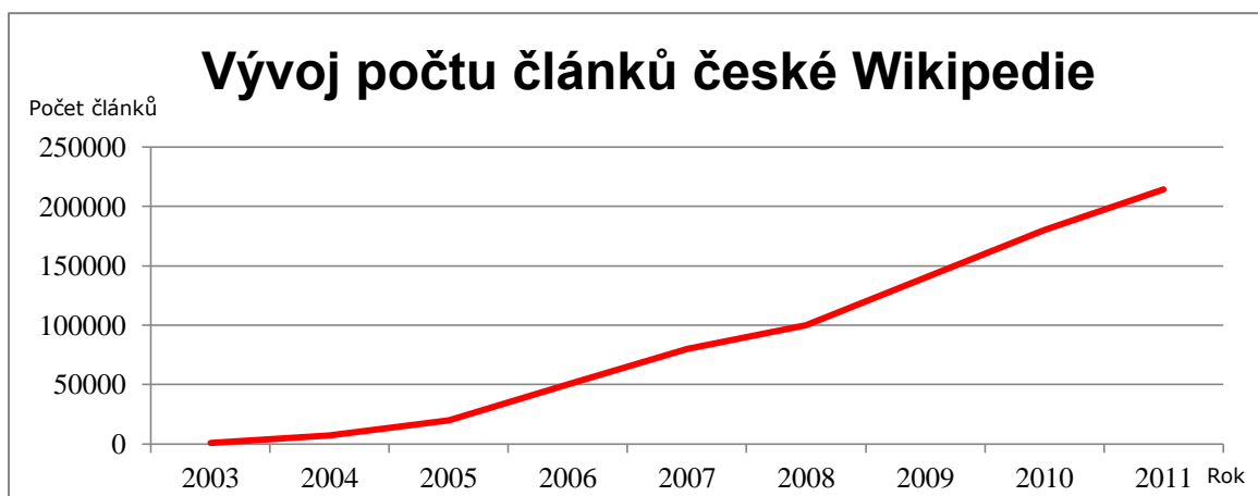
Graf 1: Vývoj počtu článků české Wikipedie
