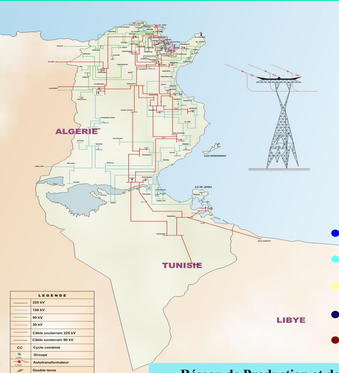
Réseau de Production et de transport d'énergie électrique
