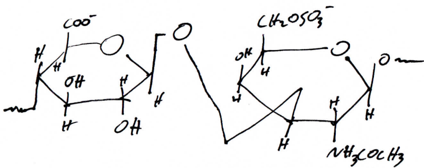
Chondroitin 6-sulfate
