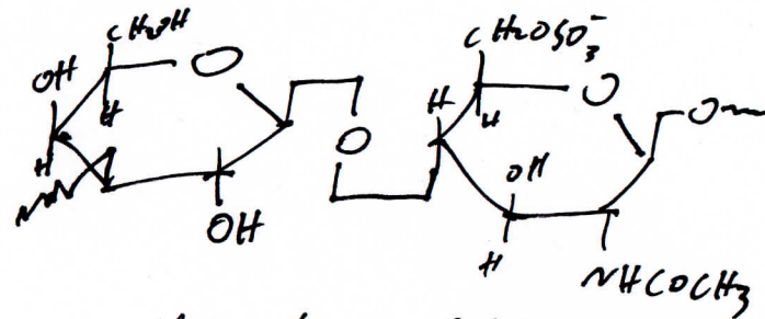
Keratan Sulfate
