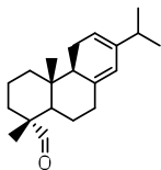
e: levopimaradienal
