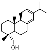
d: levopimaradienol
