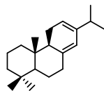
c: levopimaradiene
