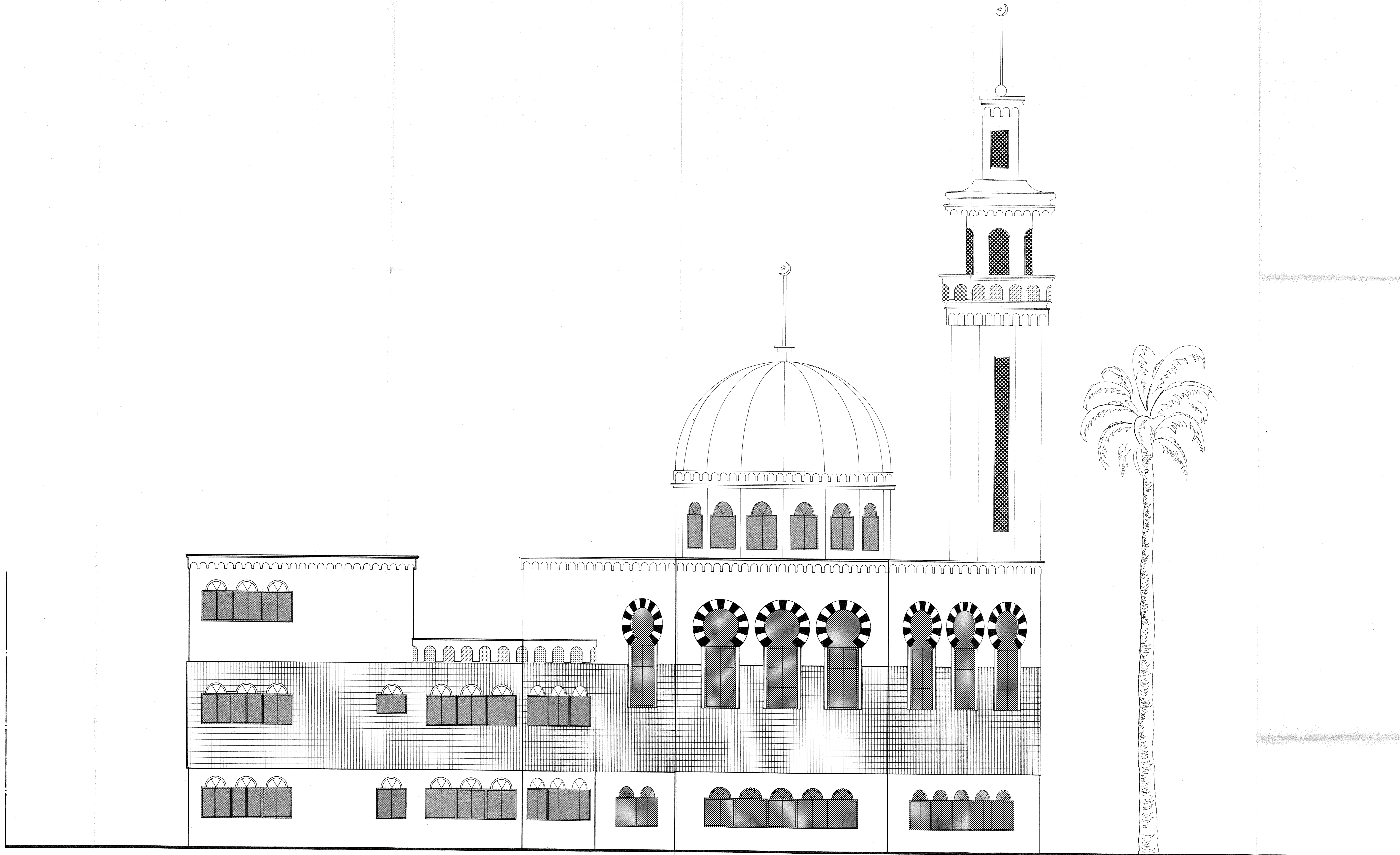
ELEVACION SUR-PONIENTE
